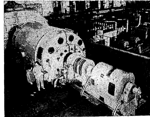
金竹山电厂排除“四人帮”的干扰破坏，坚持抓革命促生产，半年提前超额完成国家规定的各项指标。今年又提前八十三天完成了年度计划，有力地支援了工农业生产。图为四号机组在运转发电。
