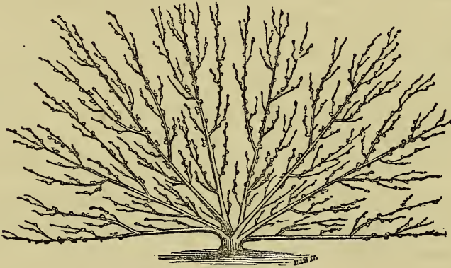
Fig. 114. Fan-shaped Espalier.
