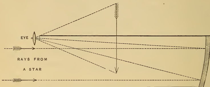
Le Mairean or Herschelien Reflecting Telescope
