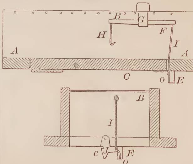
70095—N. L. Janney—Butter Stamp.
