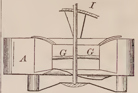
71461—A. H. Crozier— Water Wheel.
