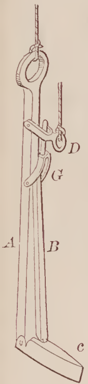
72050—A. Knapp—Horse Hay Fork.
