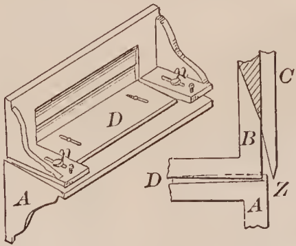
68298—D. L. Gibbs—Mortising Machine.
