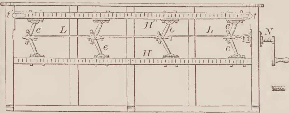
69907—Force & Renwick—Tenter Bar.
