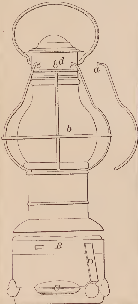
72759—J. O. Smith—Lantern.
