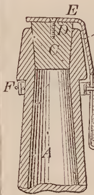
68484—H. S. Carley—Bottle Stopper.
