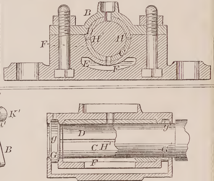
71313—P. P. Lane— Journal Box.
