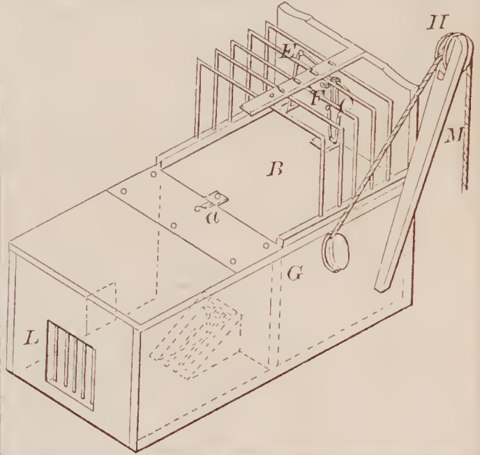
71321—G. J. Parham— Animal Trap.
