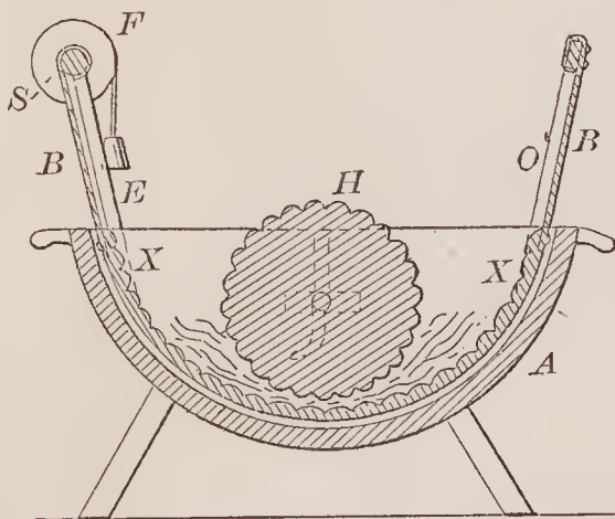
67642—J. B. Francis— Washing Machine.
