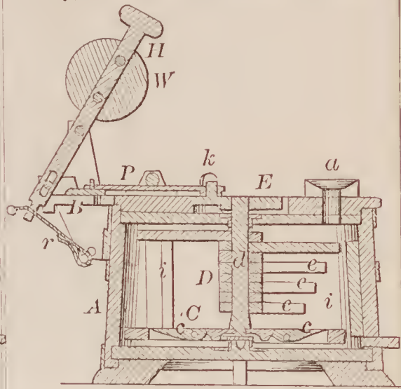
71472—J. J. Everst—Churn.
