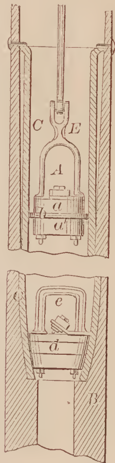
72884—B. H. Naves—Pump Piston.
