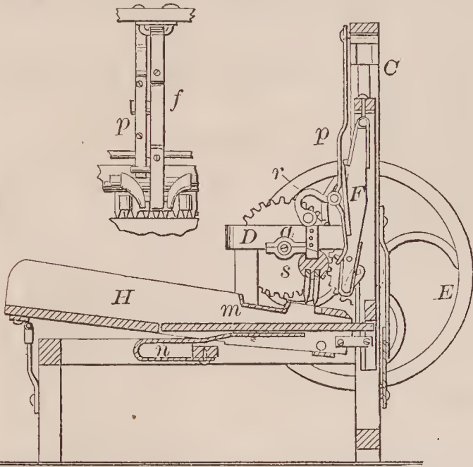
68240—A. Saeger—Wool Packer.
