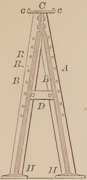
72859—A. B. Ives— Metallic Column.
