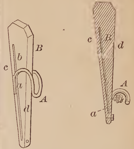
72823—W. M. Doty—Clothes Pin.
