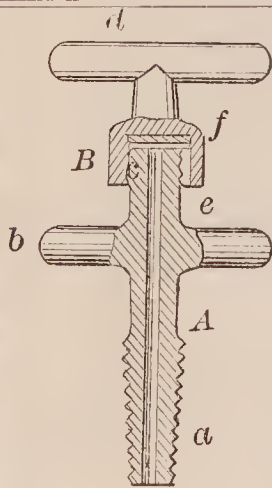
66929—O. N. Wood— Vent Plug.
