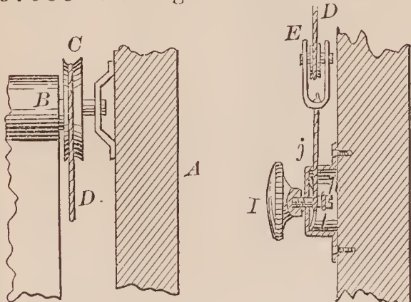
67086—H. Voigt—Curtain Fixture.
