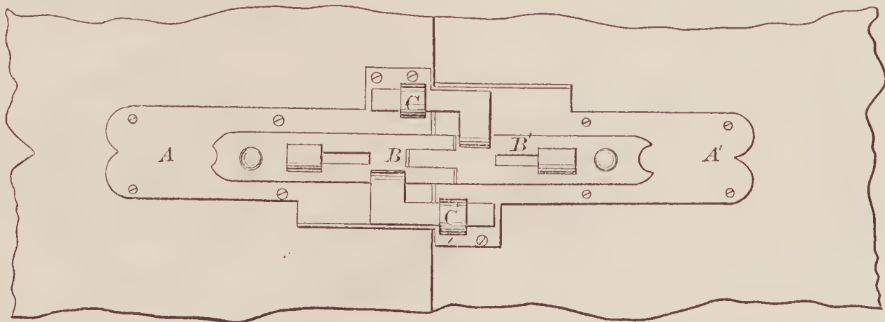
72600—P. Burke—Shutter Bolt.
