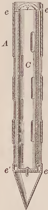
71496—J. D. Kellogg, Jr.—Tube Well.
