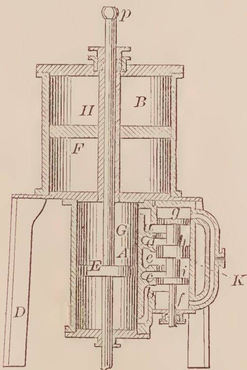
66976—J. L. Lay— Steam Engine.
