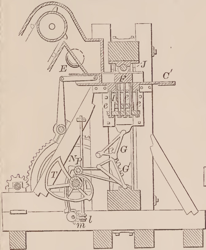
66983—J. Miller— Harvester Rake.
