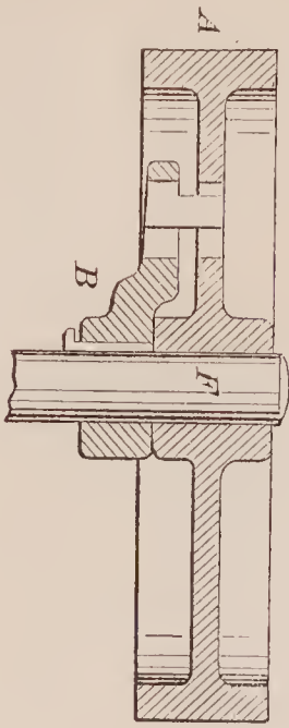
71212—E. S. Pierce—Balance Wheel.
