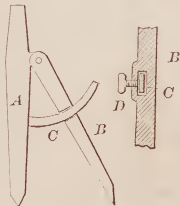
71370—E. S. Fisher—Dividers.
