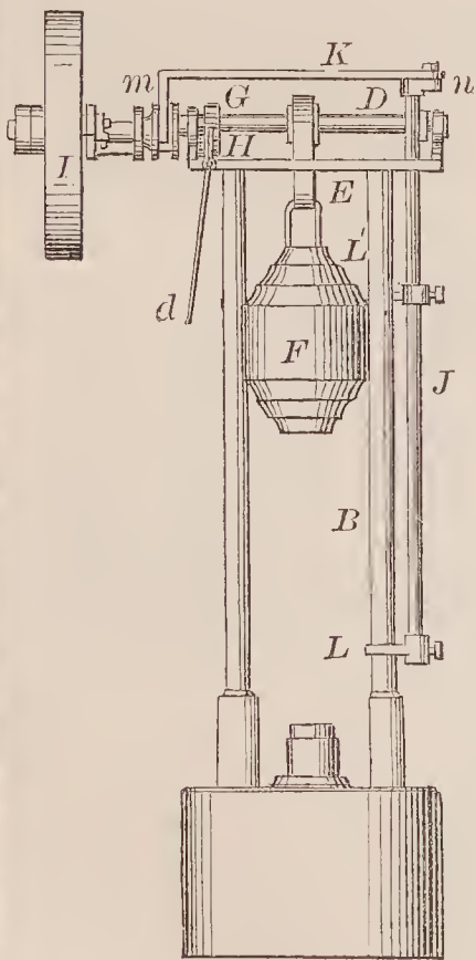
66879—L. H. Olmsted—Drop Hammer.
