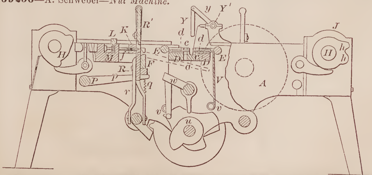
69256—A. Schwebel— Nut Machine.
