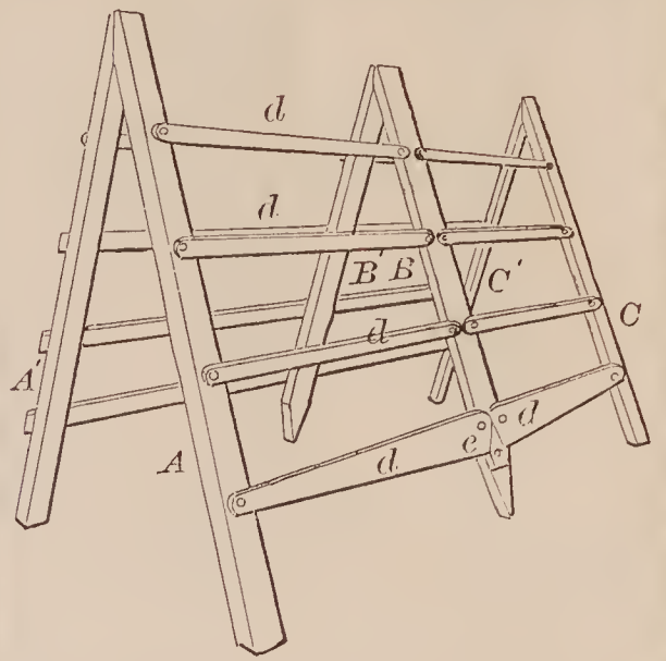
67102—L. S. Calkins— Clothes Dryer.
