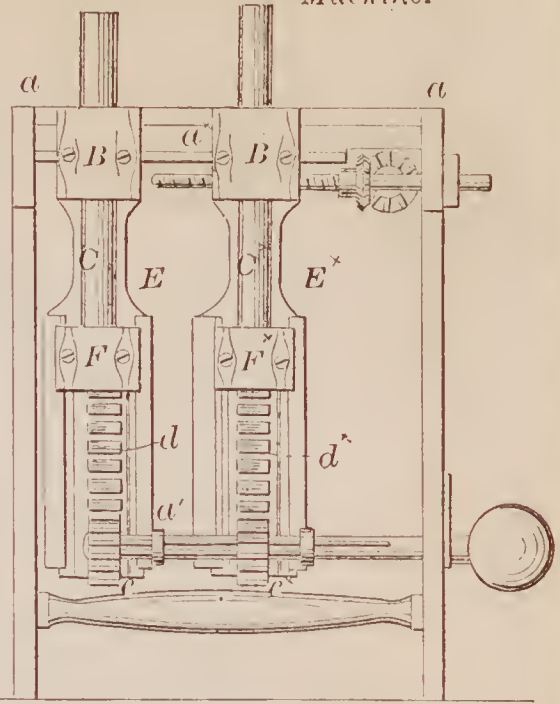
70592—R. N. Meriam— Planing Machine.
