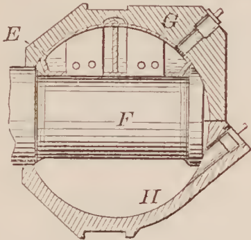
70697—G. H. Clemens—Journal Box.
