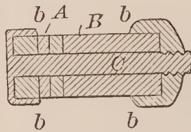
66996—O. B. Smith—Loom Picker.
