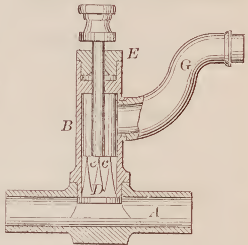
70919—J. E. Tucker— Faucet.
