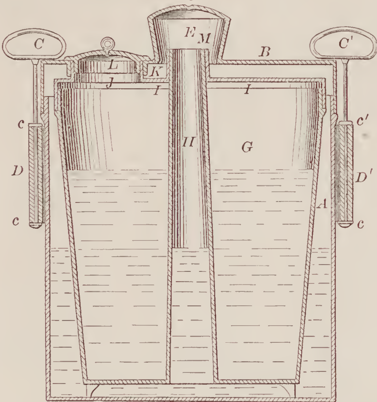
69890—H. Adler— Boiler.
