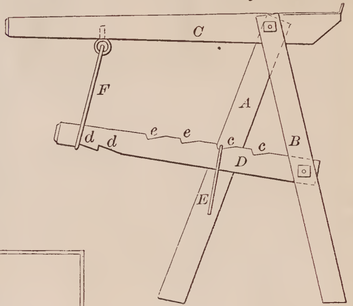
68395—O. B. Sutton— Carriage Jack.
