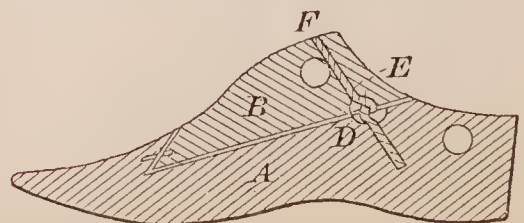
70648—A. Taylor—Last.
