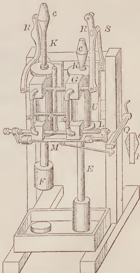
67392—F. R. Wilson— Valve Gear.
