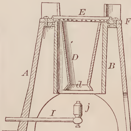
70395—J. Q. Birkey— Gas Stove.
