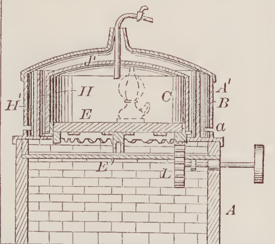
72645—J. A. Kinkle— Oven.
