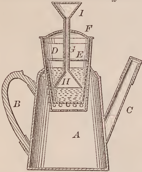
72353—J. Zimmerman—Coffee Pot.
