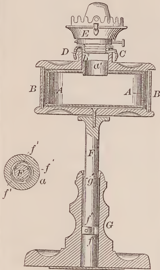
70867—J. Lee—Lamp.
