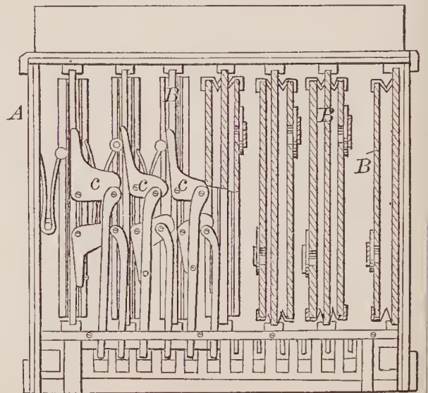
71593—K. Ebermeyr—Melodeon.
