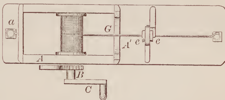
70060—J. N. Williams, Jr.— Grain Separator.
