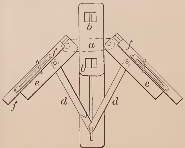
72906—J. W. Richardson—Mitre Box.
