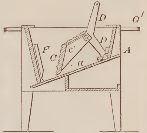
67581—M. S. Prentice—Washing Machine.
