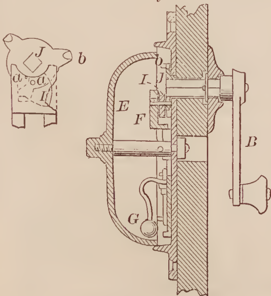
67030—Delavan & Dyson—Door Bell.
