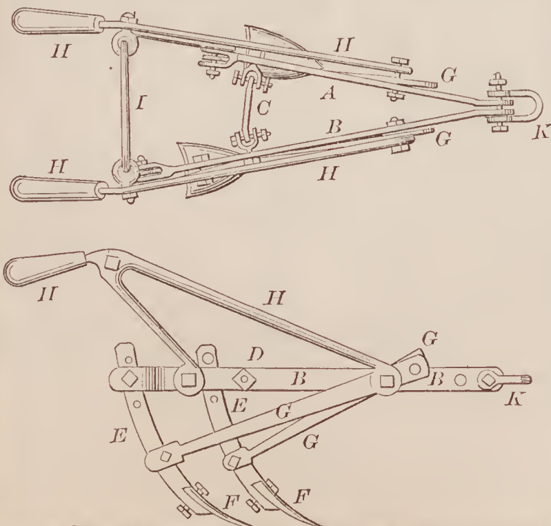
70972—J. R. Davis—Plow.
