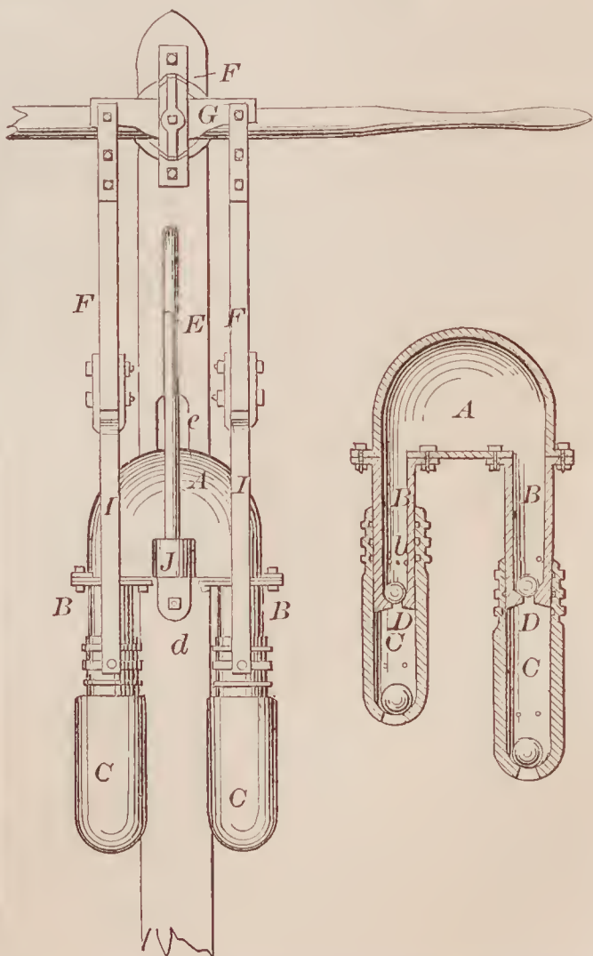
70244—J. A. Morrell—Pump.
