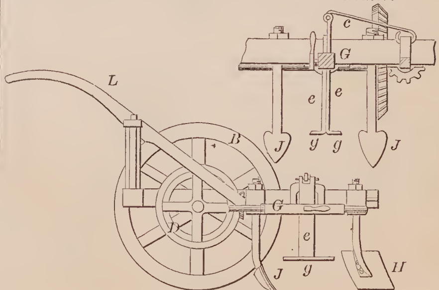
72479—E. H. & E. B. Goelet—Cotton Cultivator.
