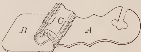
67753—J. R. Haggerty— Hemmer for Sewing Machines.
