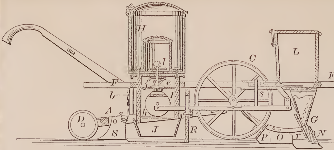
72333—J. Stark—Seed Planter.
