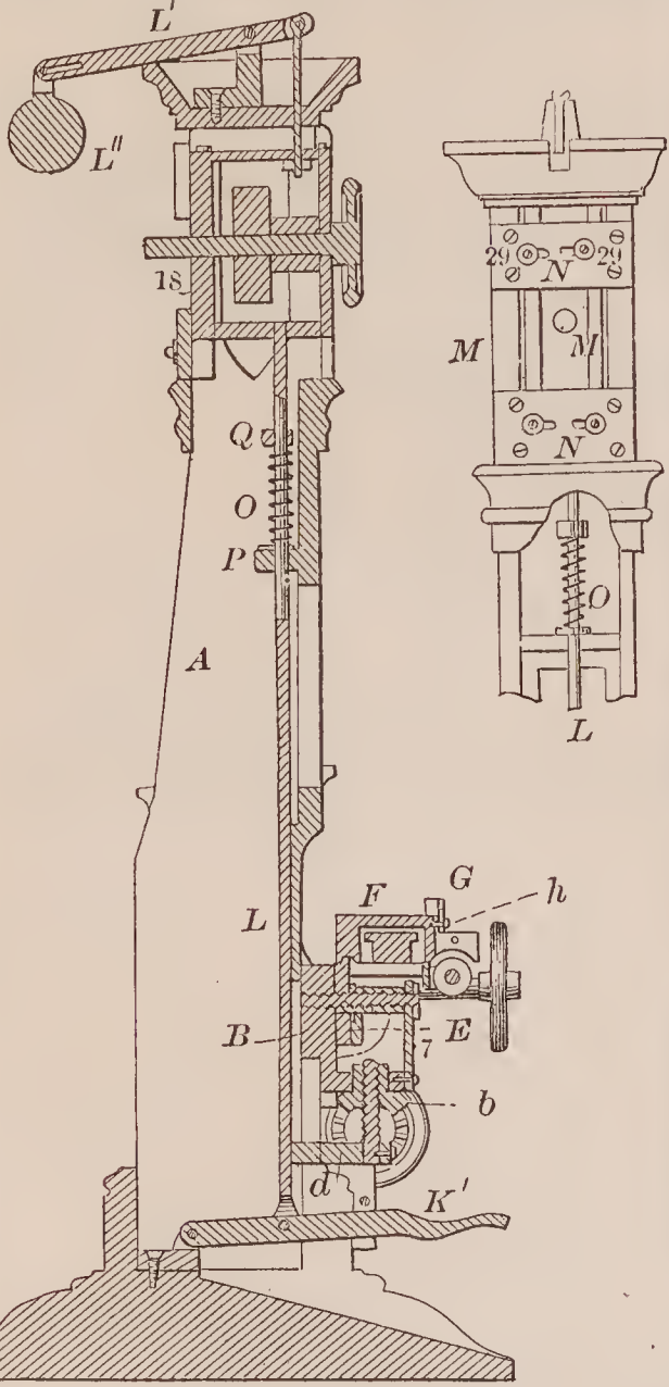
68298—D. L. Gibbs—Mortising Machine.
