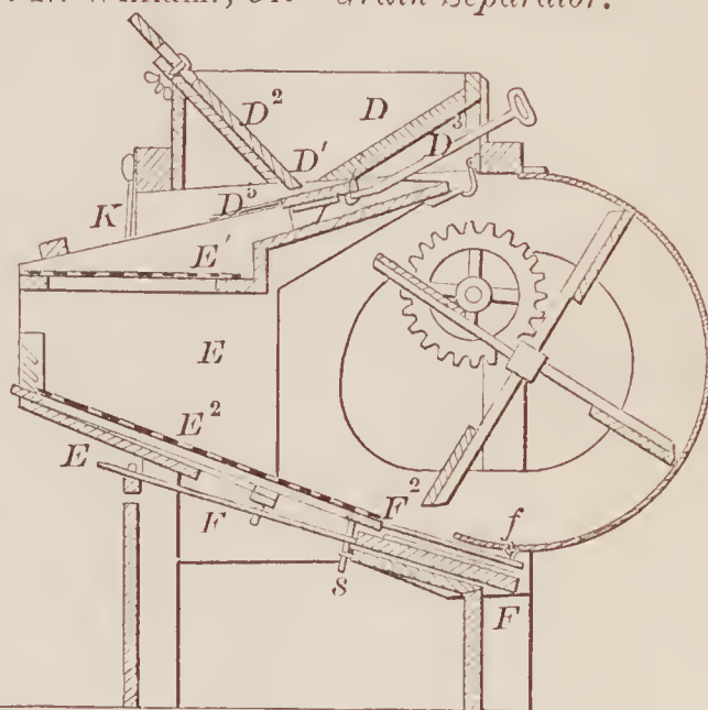
70060—J. N. Williams, Jr.— Grain Separator.
