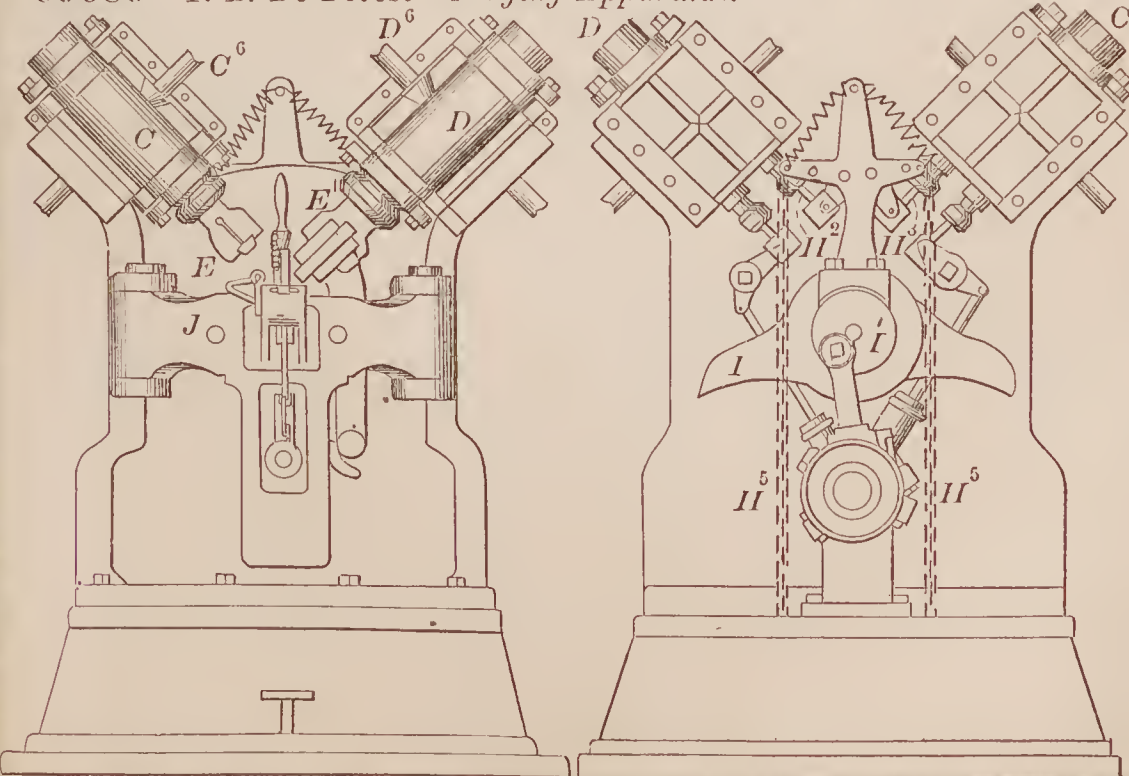
69080—T. B. De Forest—Forging Apparatus.
