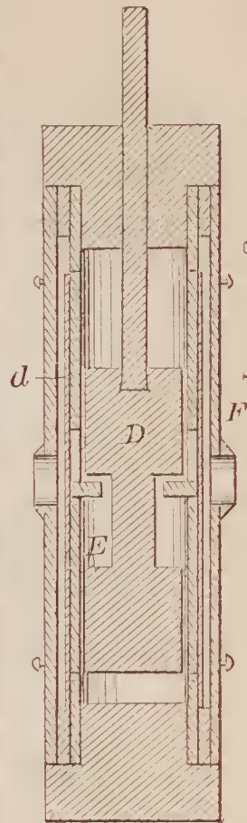
70842—J. M. Hirlinger—Pump.
