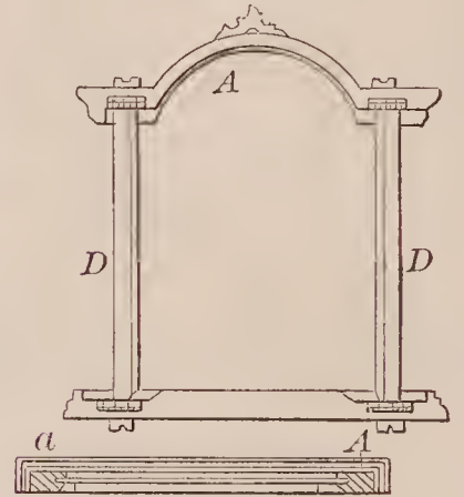
68730—O. L. Gardner— Mirror Frame.
