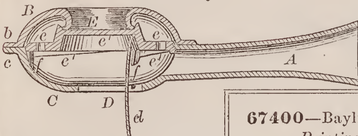
67399—W. W. Ball—Tuyere.
