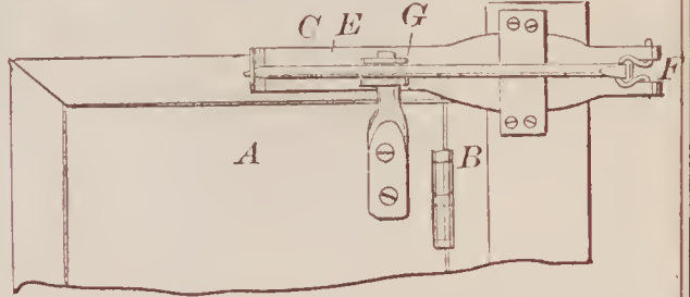
67525—H. S. Frost— Door Spring.
