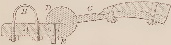
66792—W. L. Camp— Washing Machine.
