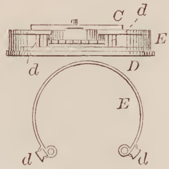
67223—O. F. Stedman— Watch.
