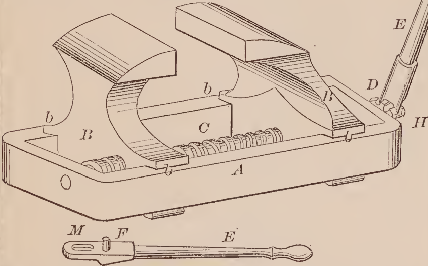
72921—P. Shellenbock—Vise.
