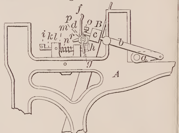
71480—F. Haigh— Loom.
