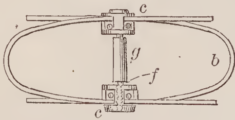
67795—G. H. Palmer— Mortise Knob Latch.
