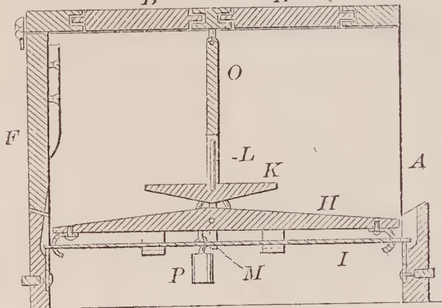
67959—I. N. Connell—Animal Trap.
