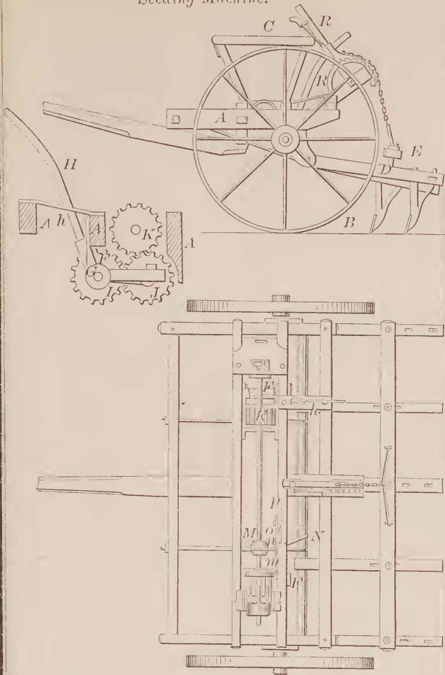
69532—Barber & D. C. & G. W. Van Brunt— Seeding Machine.
