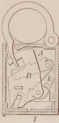
70409—J. L. Chambers— Register Padlock.
