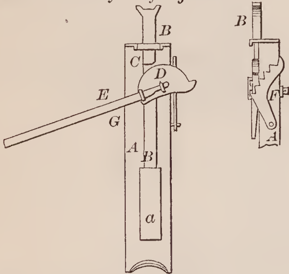
70647—Tait & Avis—Refrigerator.
