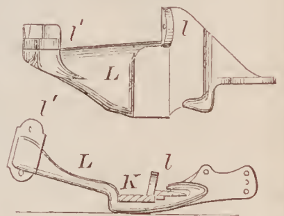
67883—L. G. Kniffen— Harvester.
