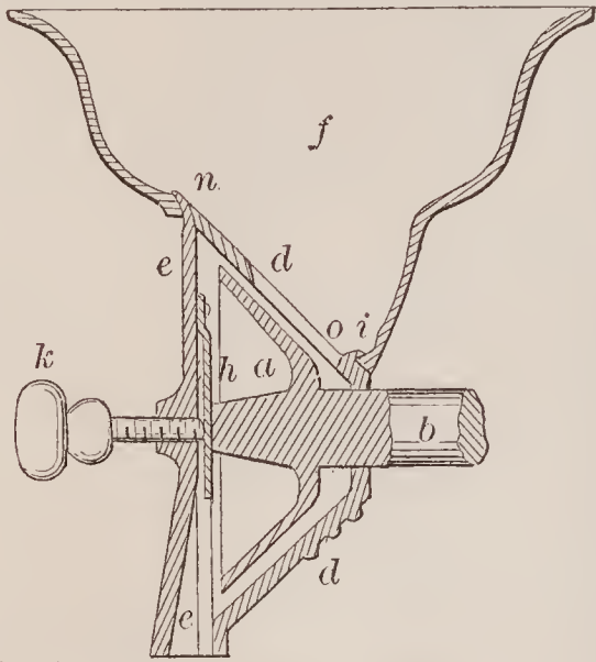
67618—J. Watrous, Jr.— Coffee Mill.
