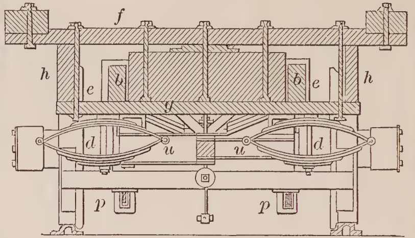
70491—Woolsey & Hubbell—Sled.
