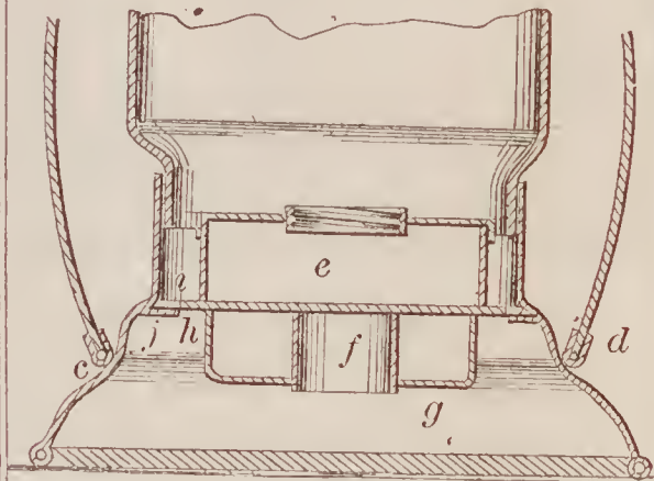
67510—J. E. Cross—Lantern.
