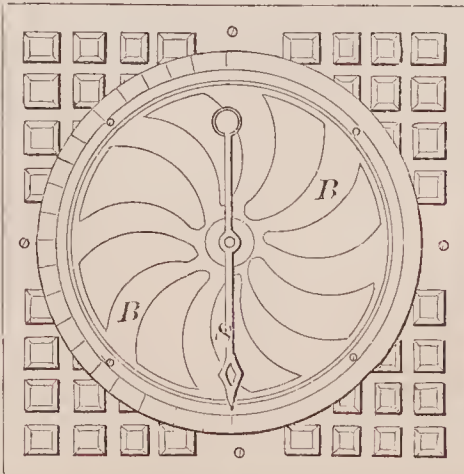
72084—J. T. Buckley—Automatic Register.
