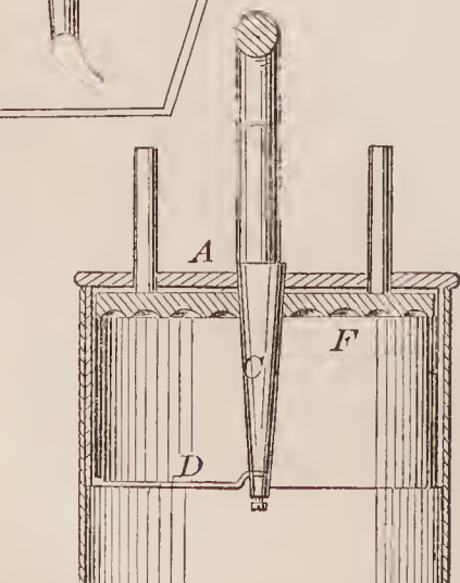
69690—A. N. Merritt— Butter Cutter.
