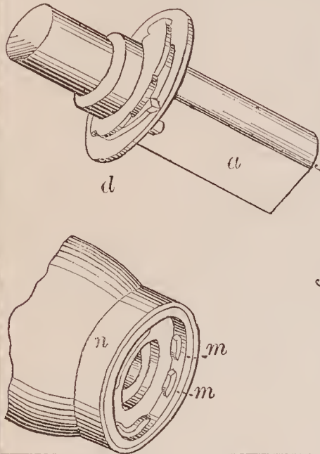
70100—J. L. Manlove—Seed Planter
