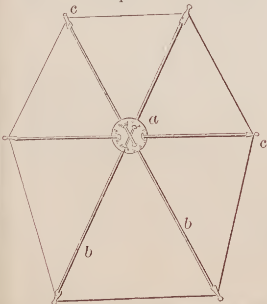
71232—J. Shepard—Kite Frame.
