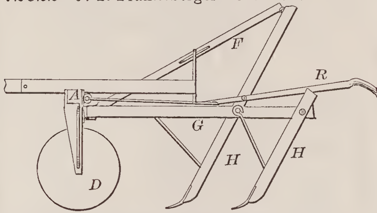
72622—J. T. Frankeberger—Cultivator.
