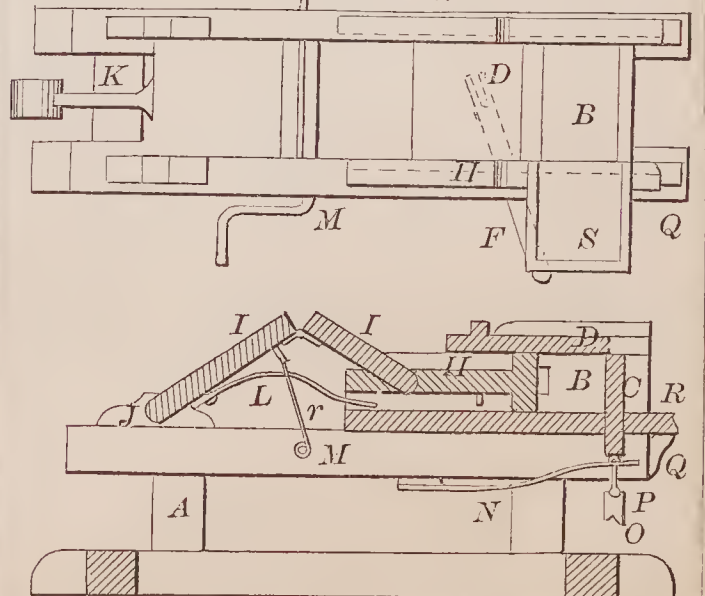
70999—M. S. Harsha— Concrete Brick Machine.
