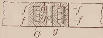
68687—J. Beck—Ticket Punch
