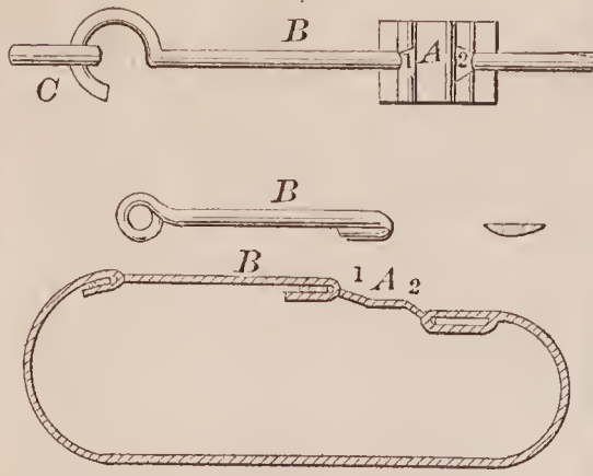
71338—J. R. Speer—Cotton Bale Tie.
