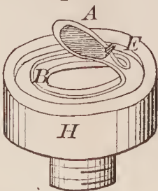
69763—H. G. Cady—Pump Valve.
