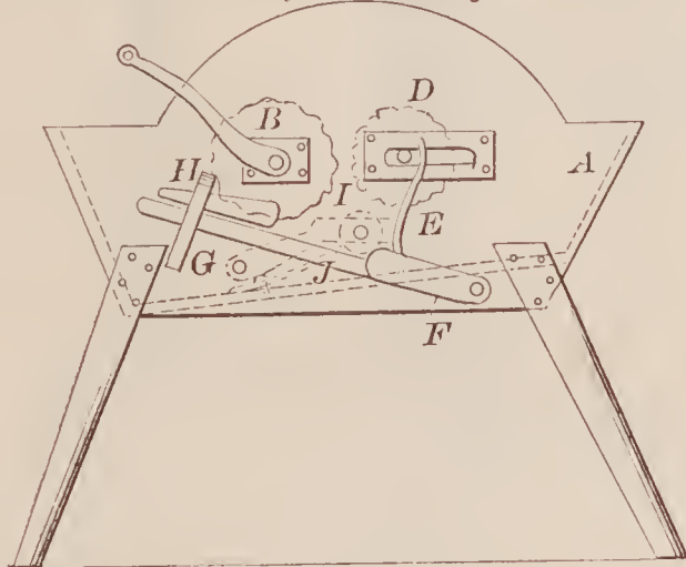
66775—J. G. Bailey—Washing Machine.
