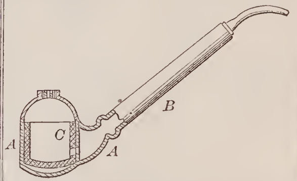
67299—J. S. Hawley—Tobacco Pipe.
