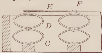
67776—M. Le Page— Spring Bed Bottom.
