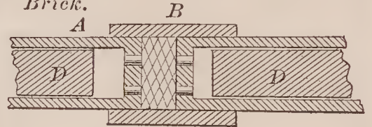
68244—O. W. Seely—For Pressing Brick.
