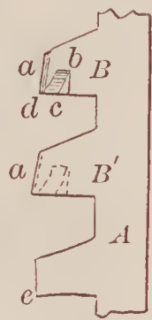
67369—W. R. Stephenson—Saw.
