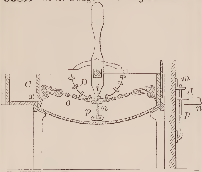
66811—J. G. Dodge—Washing Machine.
