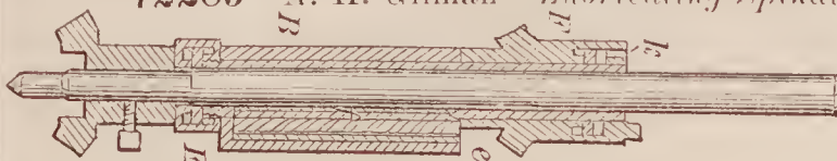
72285—A. H. Gilman—Lubricating Spindles.
