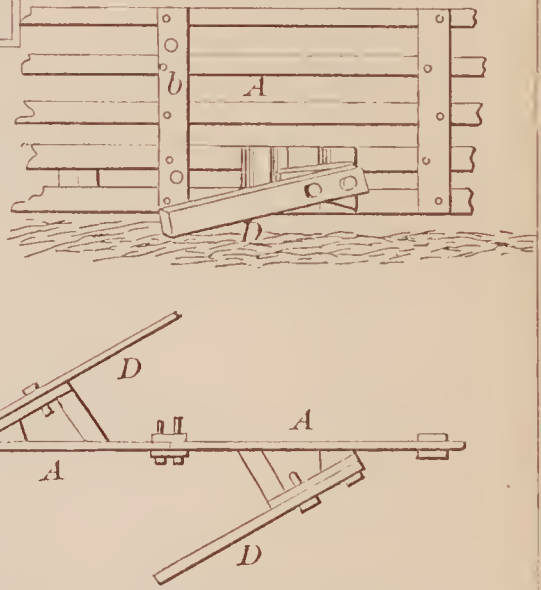
72474—W. K. Fuller—For Ventilating Mill Stones.
