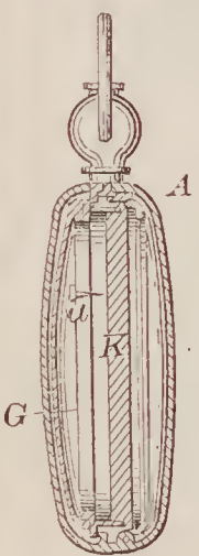
67224—O. F. Stedman— Watch Case.
