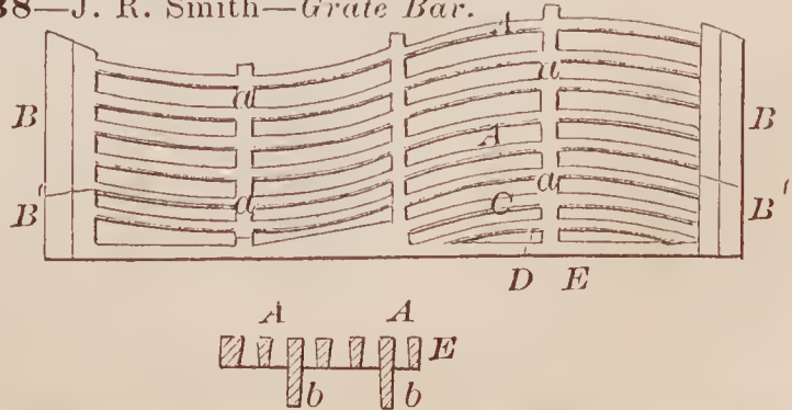
70638—J. R. Smith— Grate Bar.
