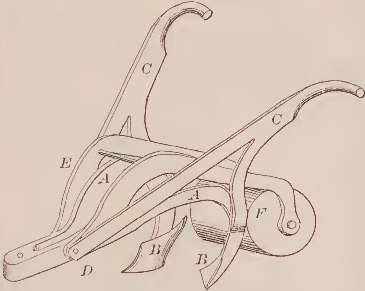
68329—A. J. Combs— Corn Coverer.
