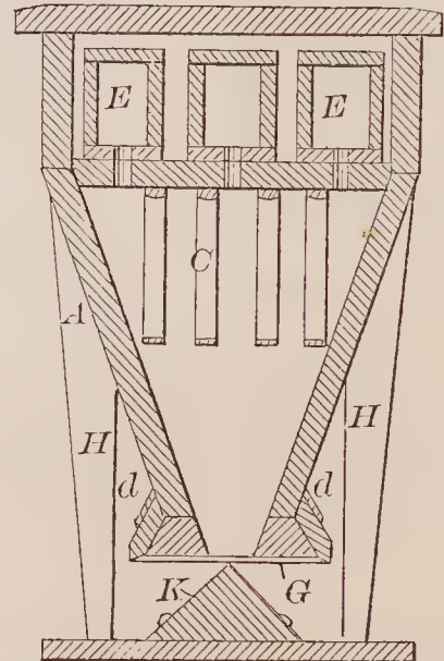
72308—J. R. Martin—Beehive.
