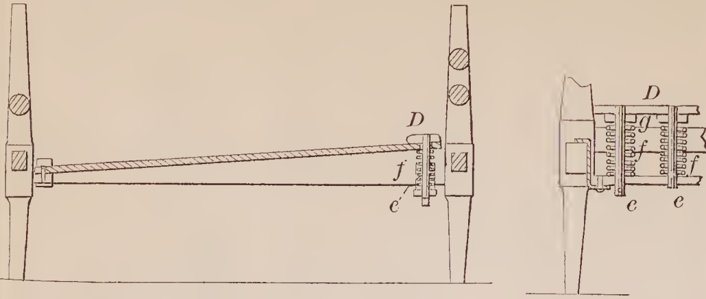
70687—A. Bingham— Bed Bottom.
