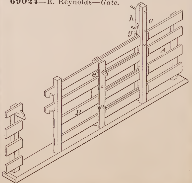
69024—E. Reynolds— Gate.
