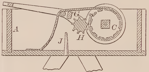
67014—J. A. Ayres—Screwdriver.
