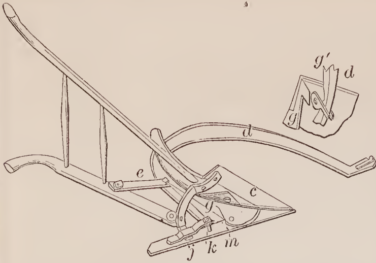
69867—J. Vandegrift— Plow.
