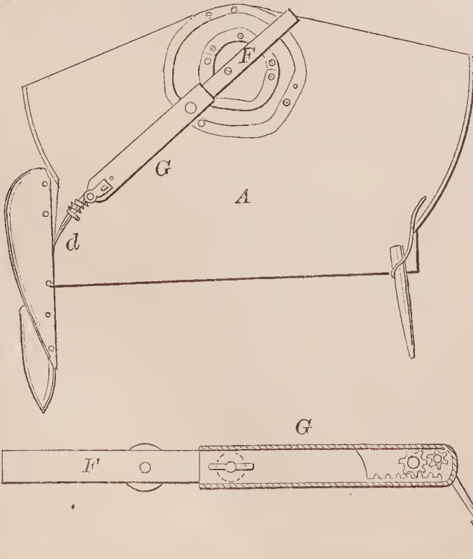
66983—J. Miller— Harvester Rake.
