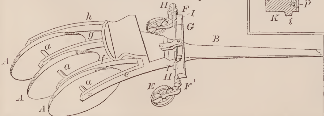
66802 —M. A. & I. M. Cravath— Revolving Plow.
