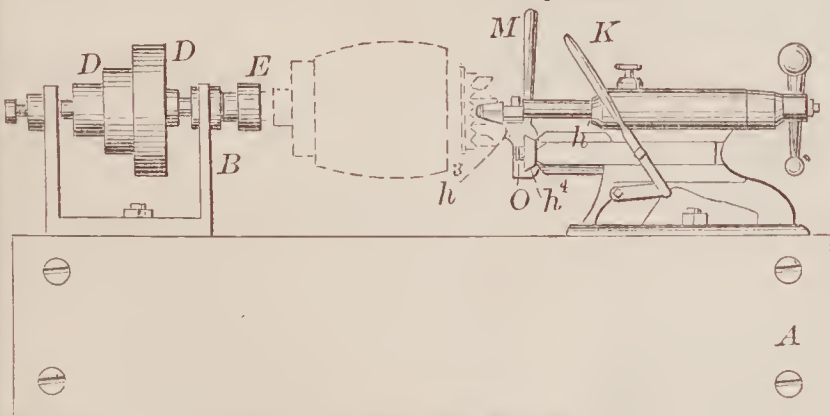
67757—S. L. Hart— Wood Turning Lathe.
