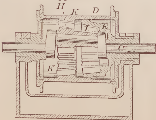
70122—J. F. Rochow—Hoisting Apparatus.
