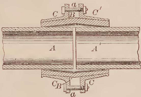
68388—J. H. Rhodes—Pipe Joint.
