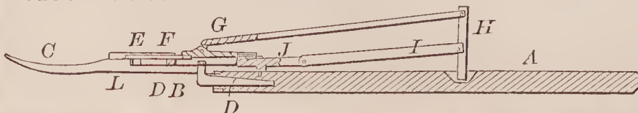
71971—E. G. Bullis—Grain Fork.
