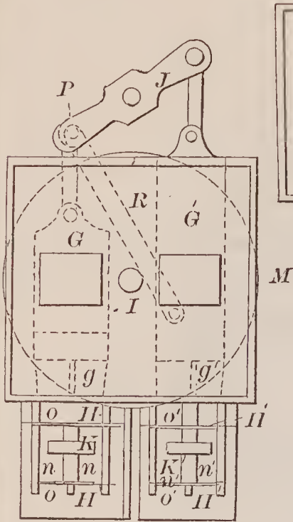
67551—H. & O. Jarecki—Engine Lubricator.
