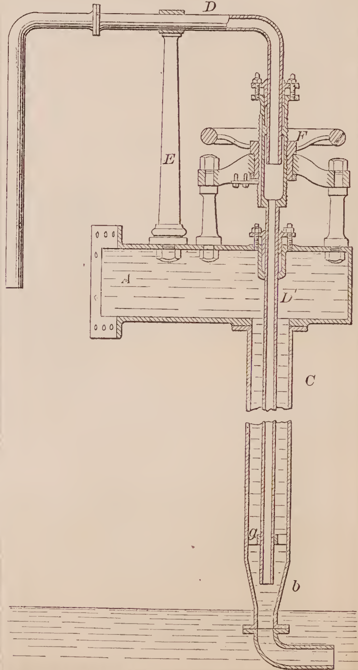
68382—F. Ortlieb— Condenser.
