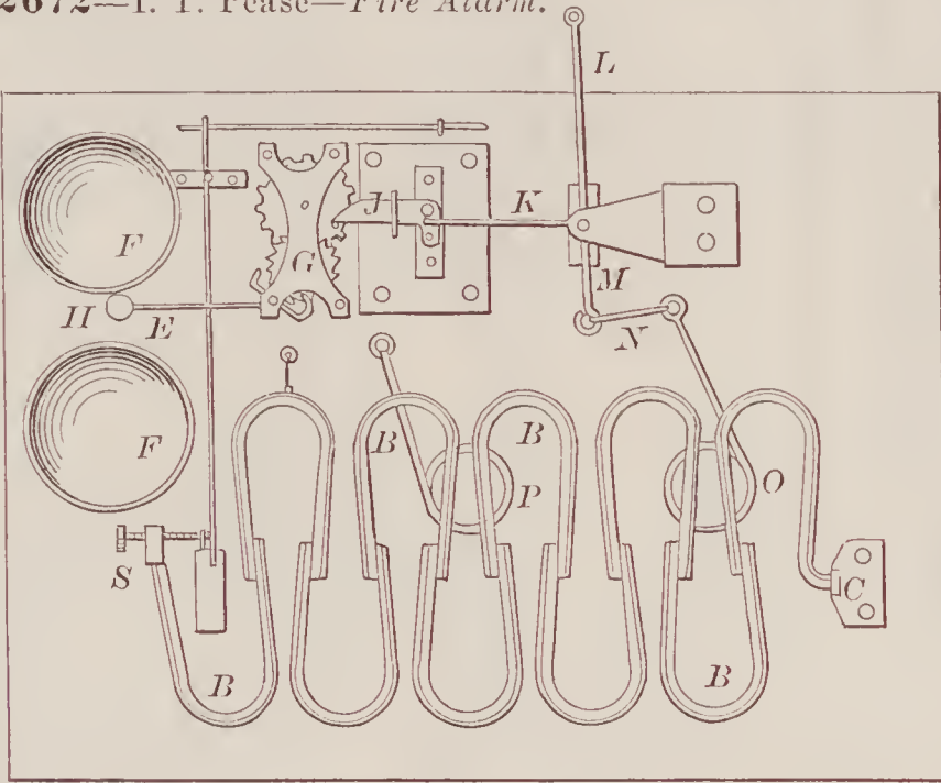
72672—I. T. Pease— Fire Alarm.
