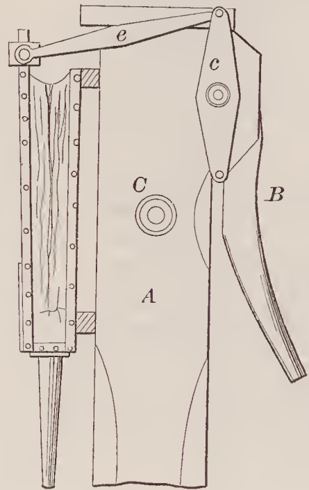
72620—G. R. Forsyth—Pump.
