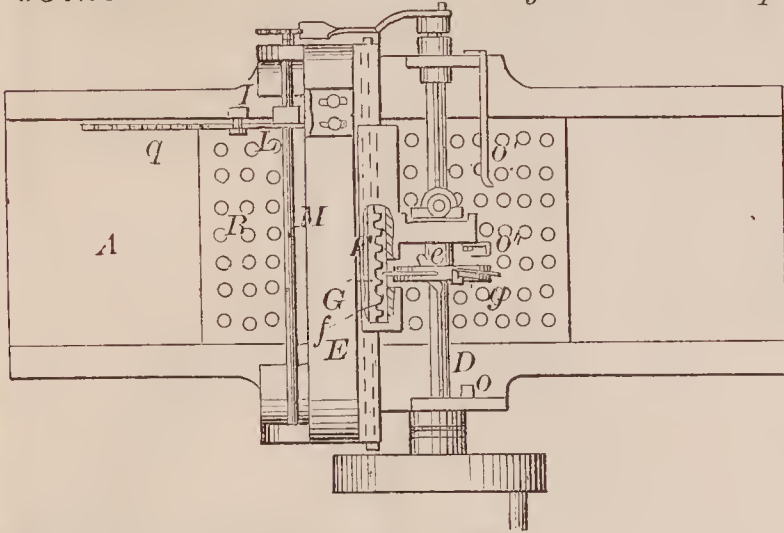
68726—D. Fuller— Gate.
