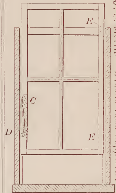
72313—J. N. McIntire—Sash Stopper.
