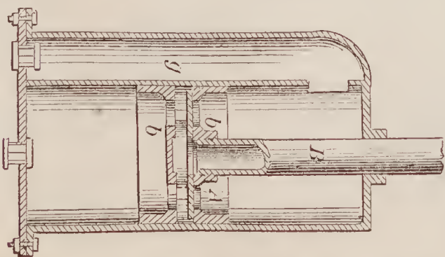
67291—C. B. Gill— Pump Piston.
