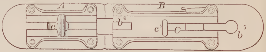
70173—J. M. & M. L. Cummings—Shutter Bowing Bolt.
