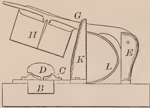
68786—Pidault & Elieze dit Lagieze—Breech-Loading Fire Arm.
