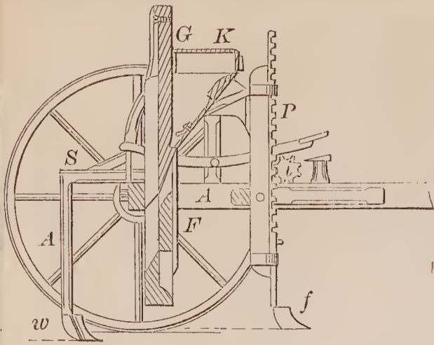
68841—R. & J. L. Cassaday— Corn Planter.
