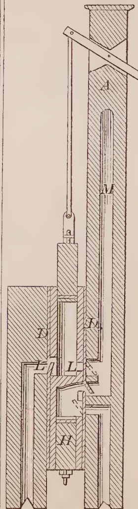
70443—J. T. Kimbel— Pump.
