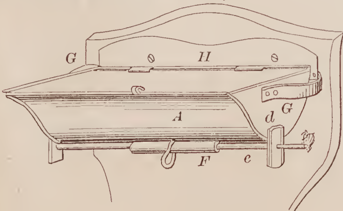
70362—A. Roesler— Match Safe.
