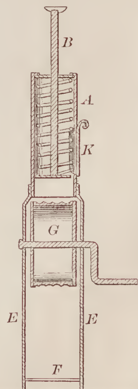
67616—L. Von Frober—Nutmeg Grater.
