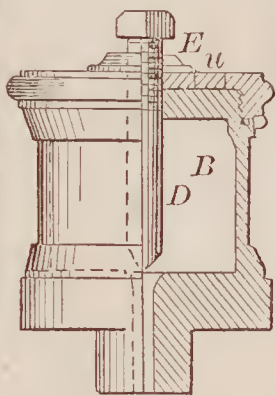
71332—M. Sellers— Journal Lubricator.
