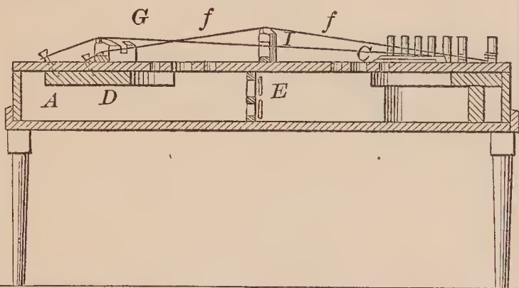
72824—E. Durand—Dulcimer.
