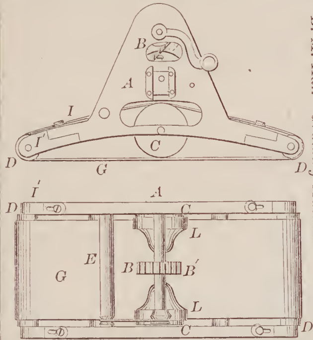
67756—W. E. Hardin— Plow.
