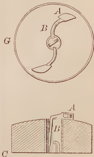
72474—W. K. Fuller—For Ventilating Mill Stones.
