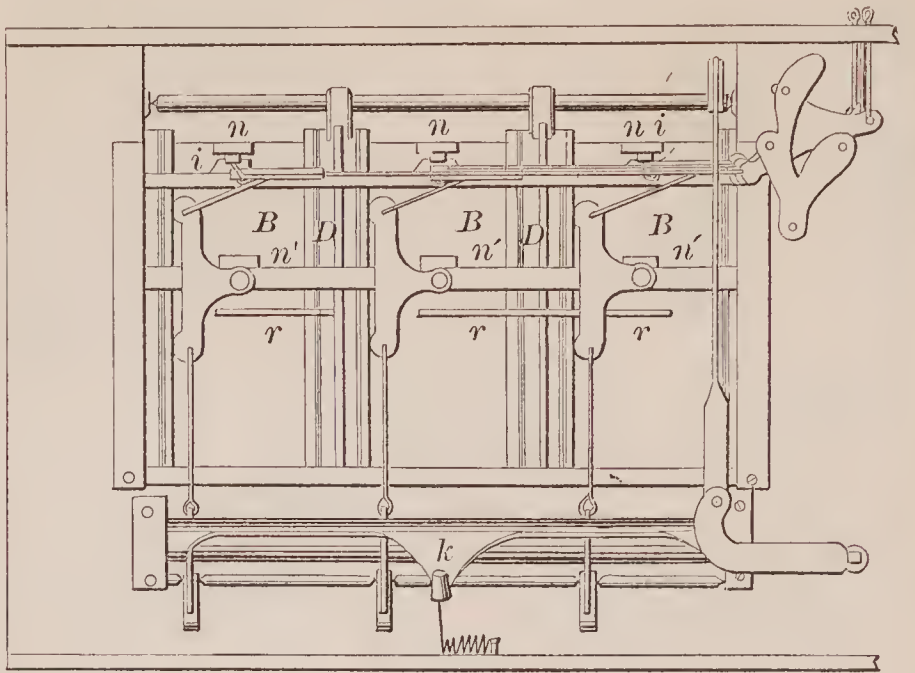
71214—H. B. Porter—Hotel Annunciator.
