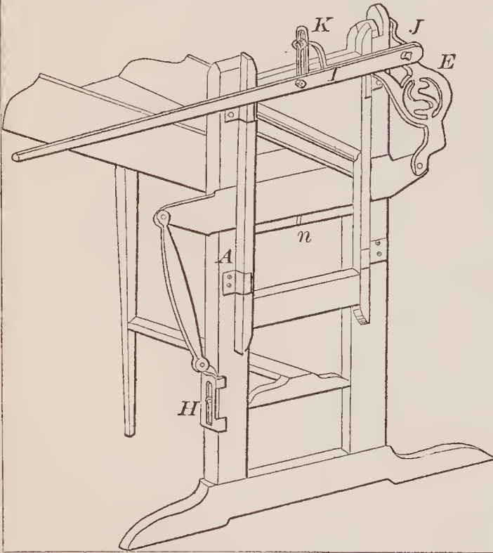
69918—J. L. Knoll— Dumping Sled.
