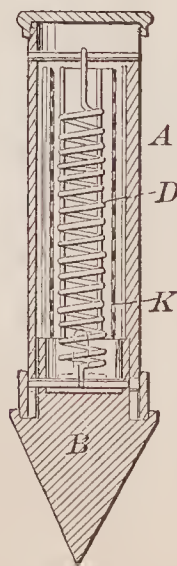
69762—H. G. Cady—Well Point.
