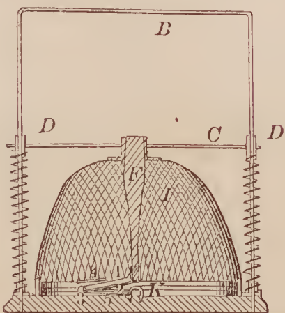
68651—S. S. Rain—Animal Trap.
