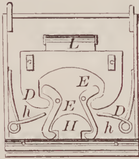
72692—A. M. Smith— Sash Lock.
