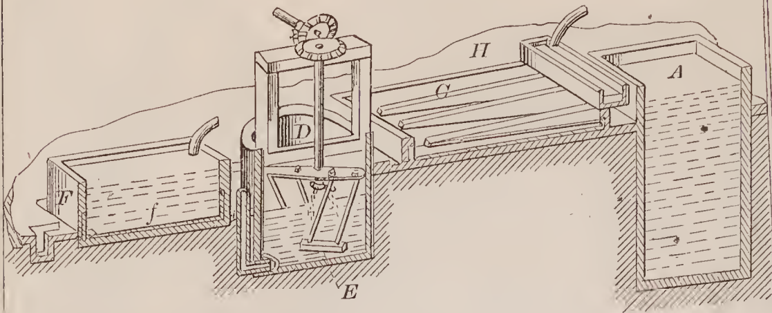
67516—A. Erkenbrecher— Starch Agitator.
