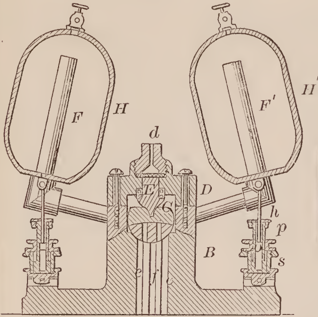
66993—G. A. Riedel—Automatic Boiler Feeder.
