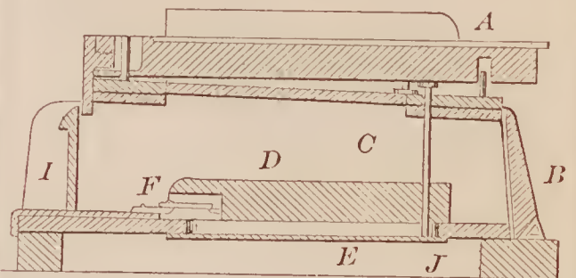
67150 —G. Wood— Melodeon.
