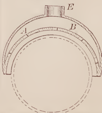
72074—J. B. Oldershaw—Hot Air Conductor.
