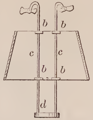
71168—E. K. Haynes—Lamp Shade.
