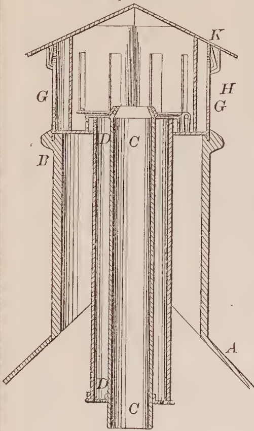
70993—B. J. Goodsell— Chimney Cowl.
