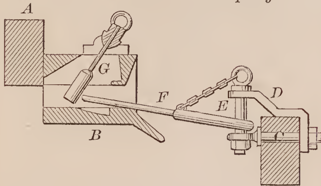
71560—G. Watt— Plow.
