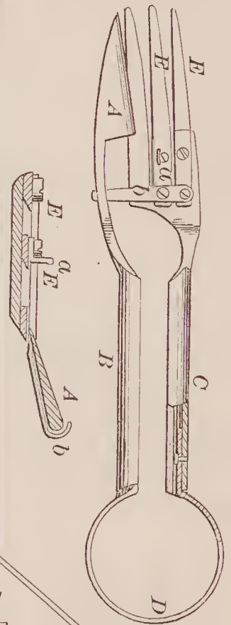
69513—E. Van Doren—Sheep Shears.
