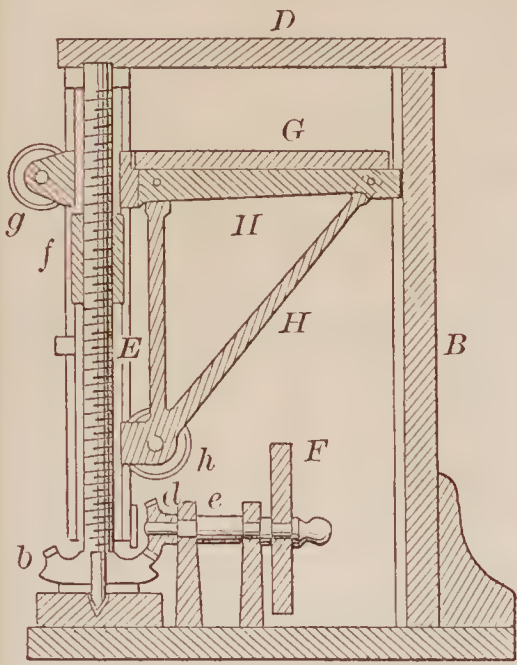
70387—E. H. Ashcroft— Elevator.
