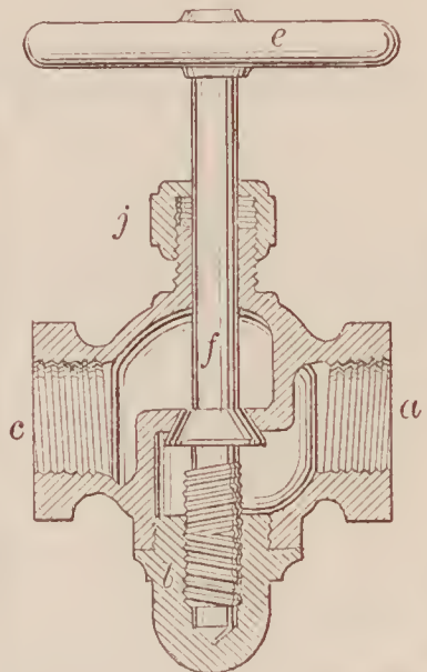
66862—M. S. Marshall—Gas Stove.
