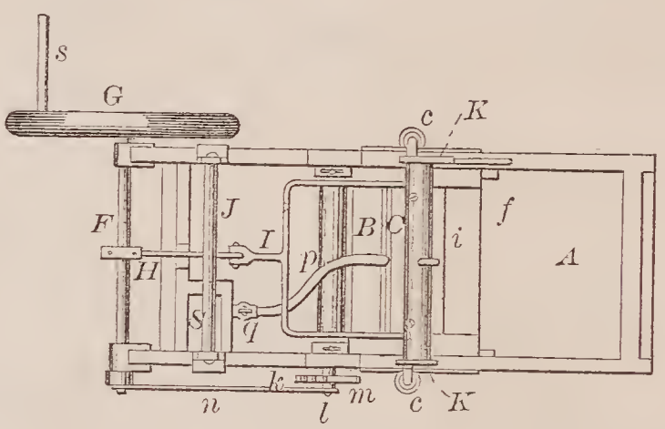
69263—J. B. Slawson—Omnibus Fare Box.
