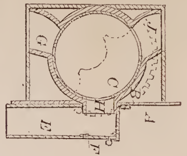
70792—R. Boyd—House Ventilator.
