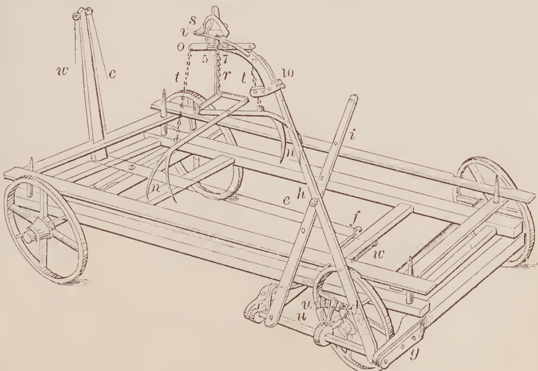
71250—A. Vose— Hay Loader.
