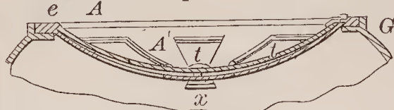
67603—J. Stephen—Pot Hole Lid.
