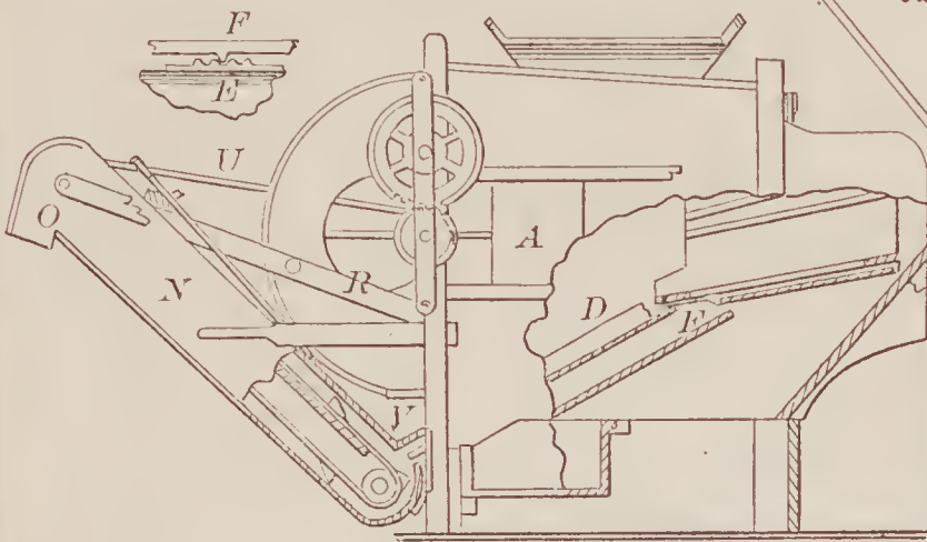
67260—J. J. Bradner—Fanning Mill.
