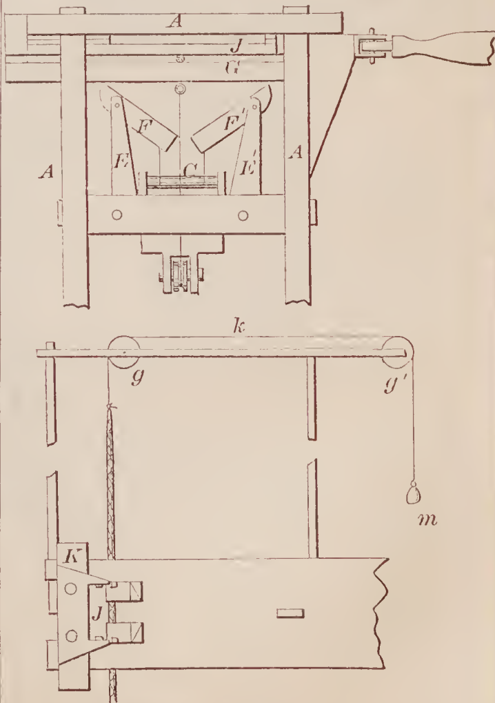
70501—H. Axtel— Whip Rolling Machine.
