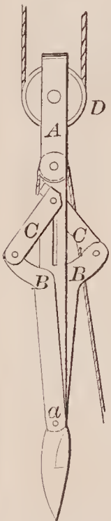
71343—P. Vanderbelt, Jr.—Horse Hay Fork.
