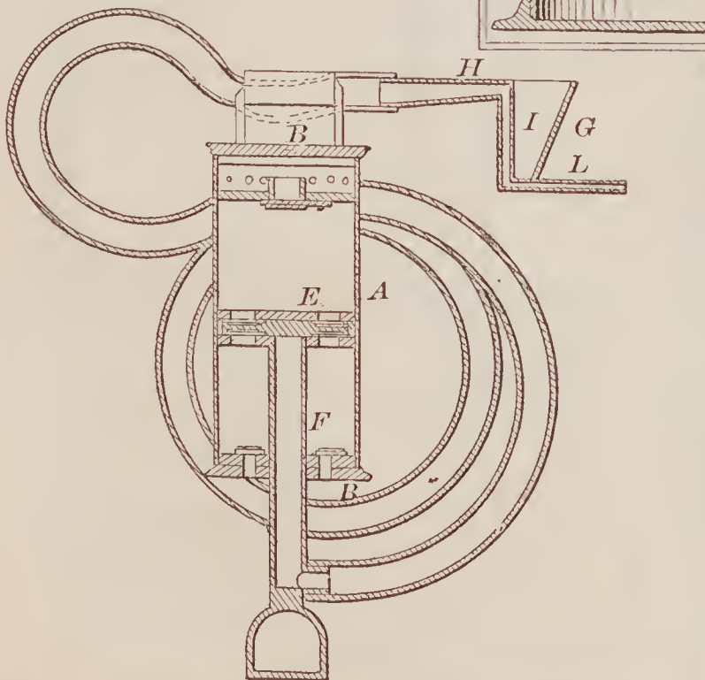
67580—E. W. Poston—Sand Ejector.
