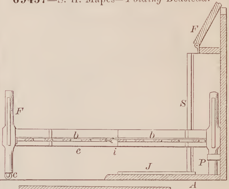
69457—S. H. Mapes—Folding Bedstead.
