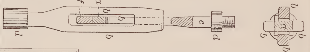
66816—J. C. Eastman—Drill Jar.
