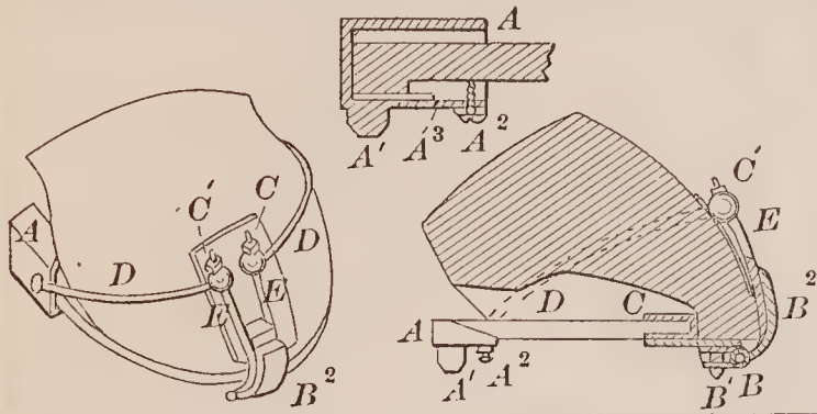
70508—J. Bevis—Washing Machine.
