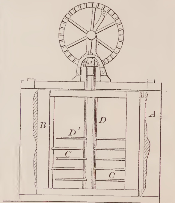
70009—H. H. Macklin— Churn.
