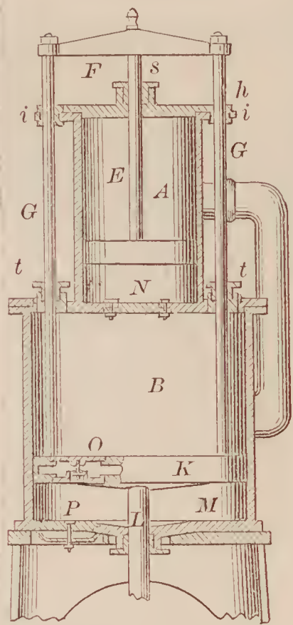
66972—J. L. Lay— Steam Engine.
