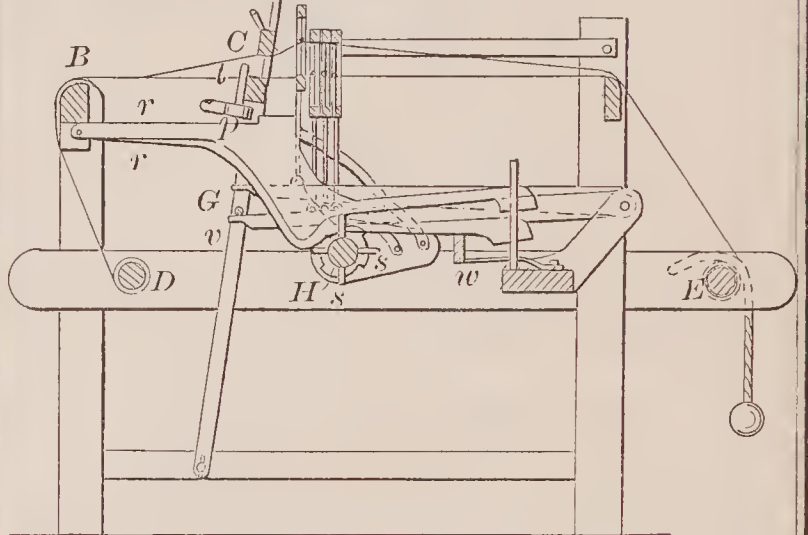
70964—H. M. Cooper—Loom.
