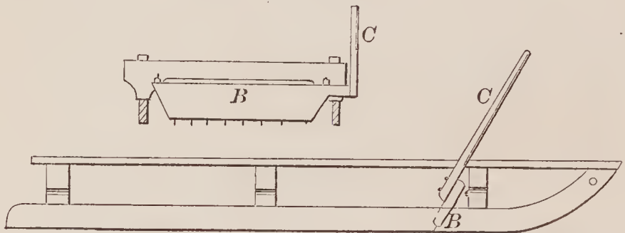
69692—T. S. Minniss— Sled Brake.
