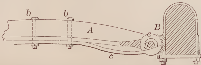
68515—J. Knox— Thill Coupling.
