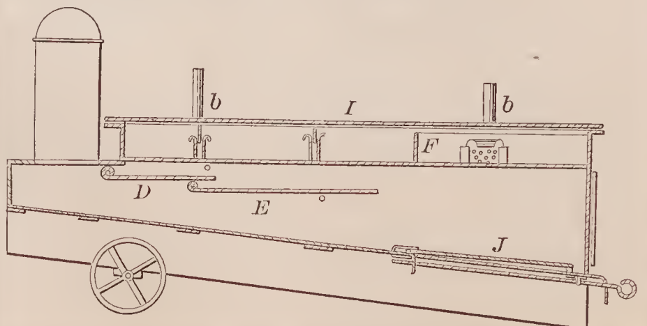
72326—H. A. Plumb—Portable Evaporator.
