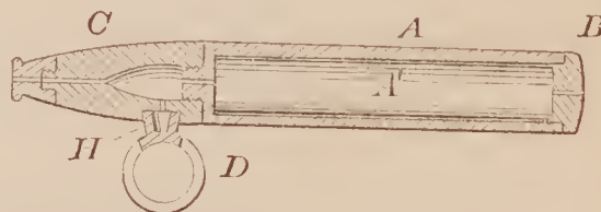
72915—J. M. Scott—Mechanical Movement.
