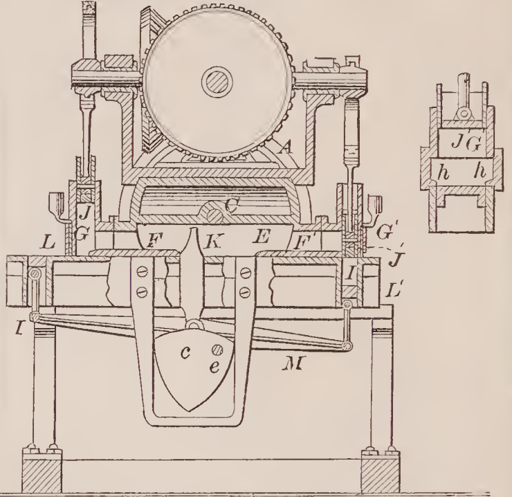
71466—H. Dueberg— Brick Machine.
