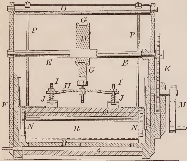
70508—J. Bevis—Washing Machine.
