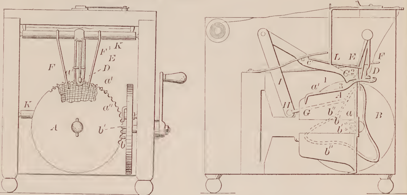
72294—J. E. Hignutt—Cinder Shovel.
