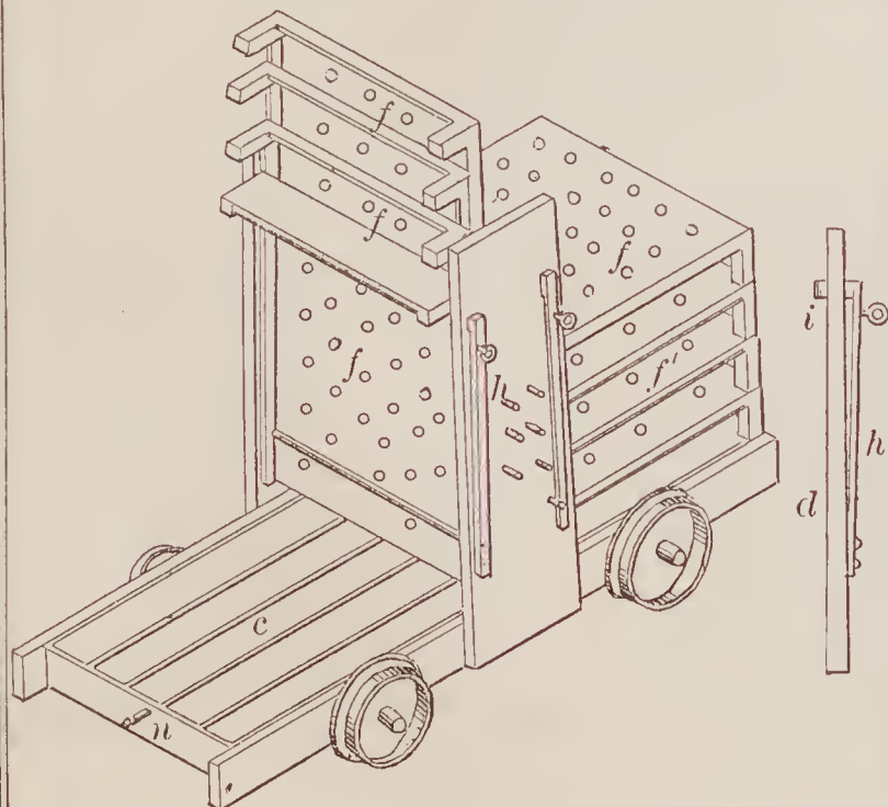
67632—J. K. Caldwell—Brick Car.
