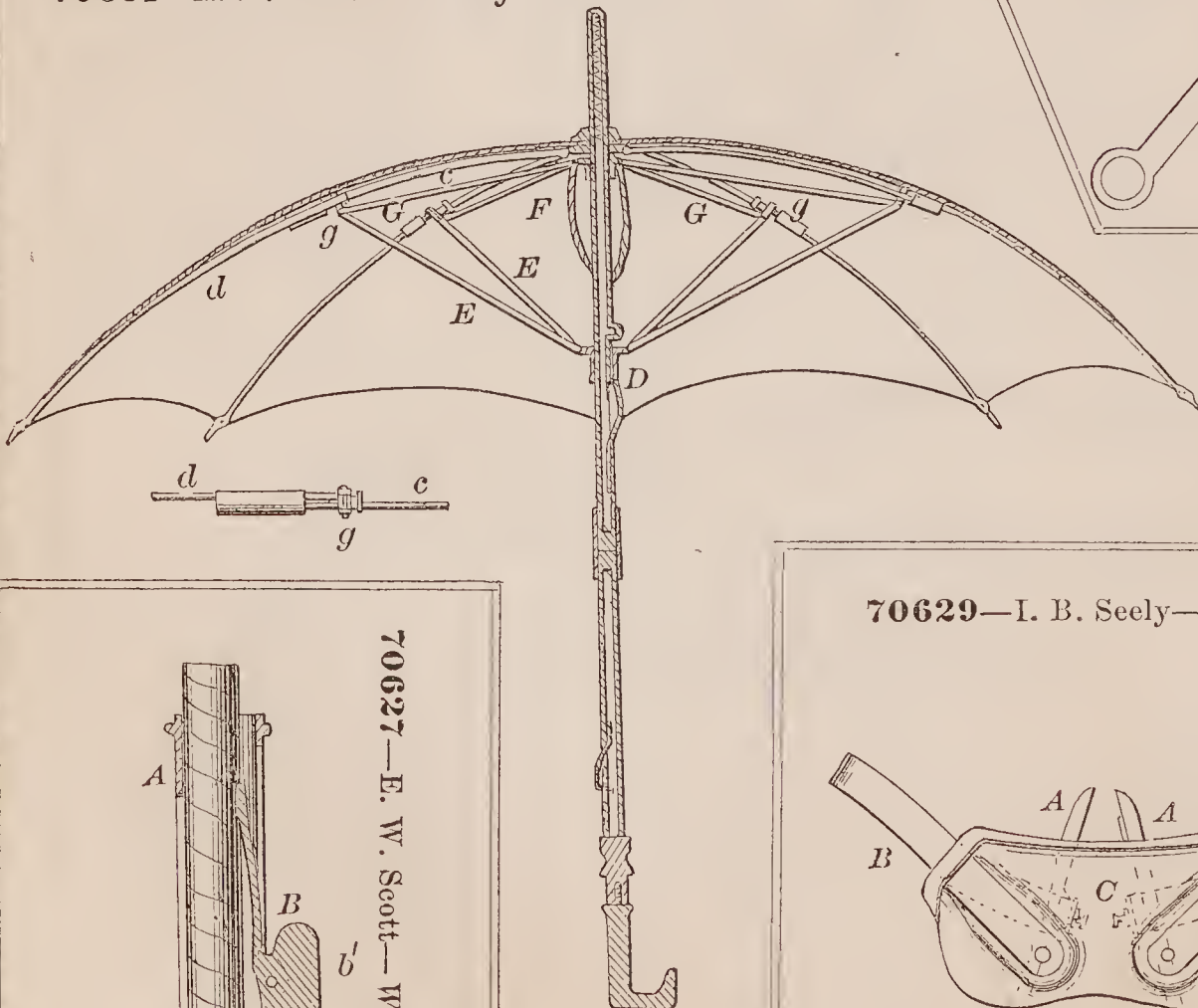
70631—A. B. Shaw—Folding Umbrella.
