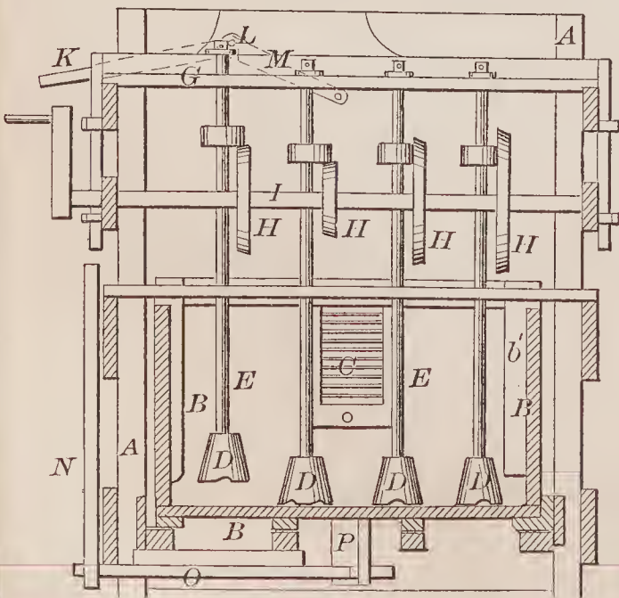
69726—J. Vail—Washing Machine.
