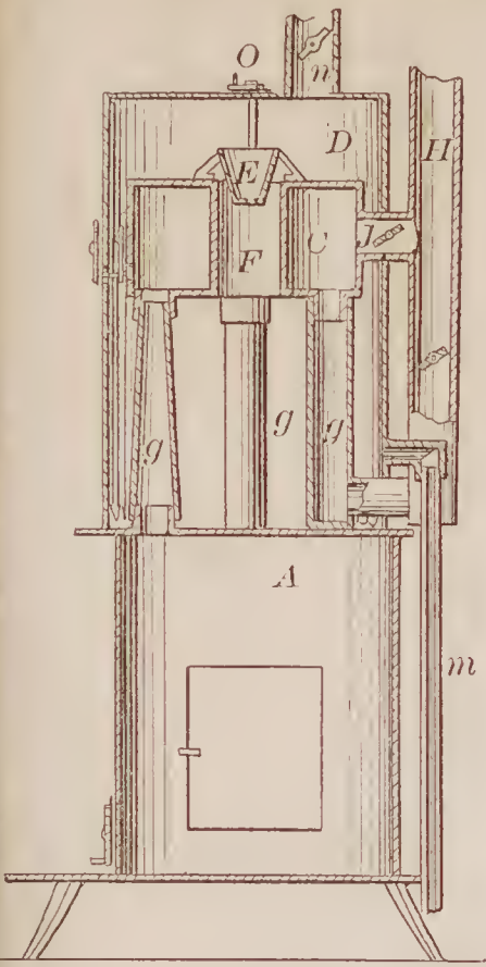
71399—J. A. Marvin—Heater.
