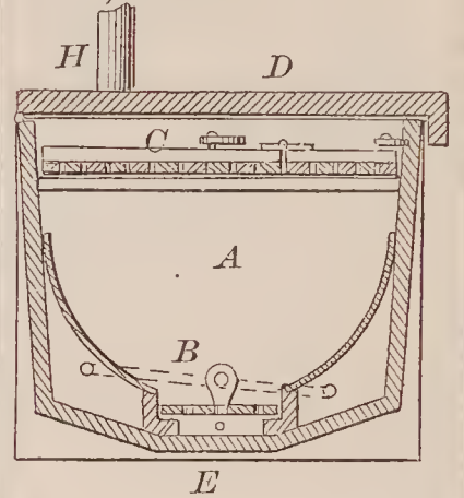
66833—W. S. Haight—For Hopping Beer, Ale, &c.
