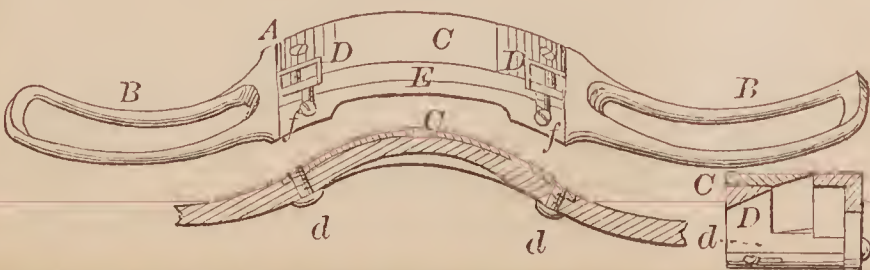
72724—F. S. Dawes—Heel Shave.
