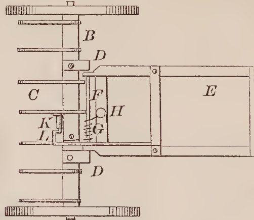
70548—O. Graham—Farm Gate.
