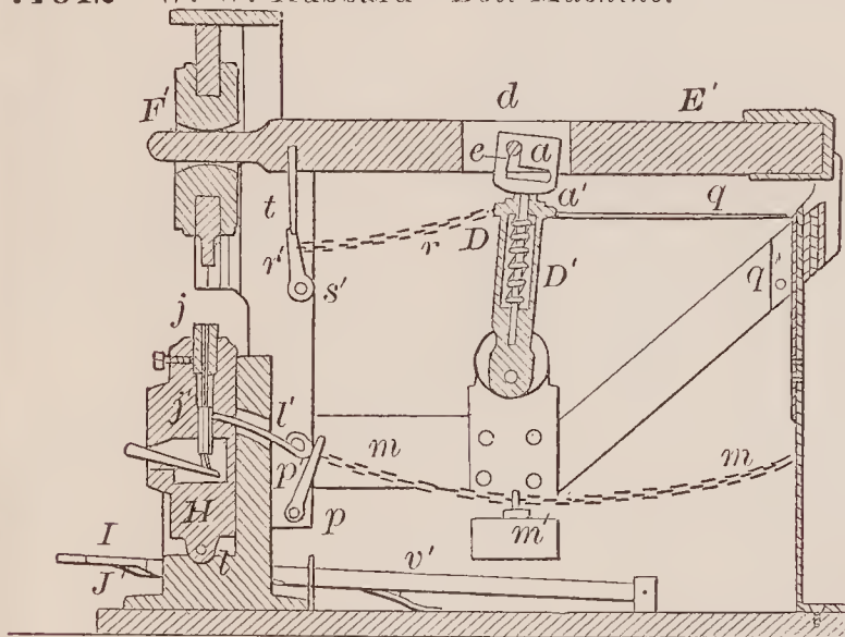
71012—W. W. Hubbard— Bolt Machine.
