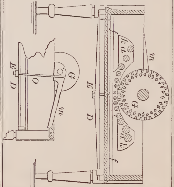
71874—J. H. Haskell— Washing Machine.
