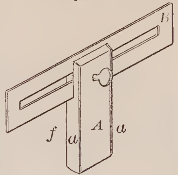
67338—J. Morass—Square.
