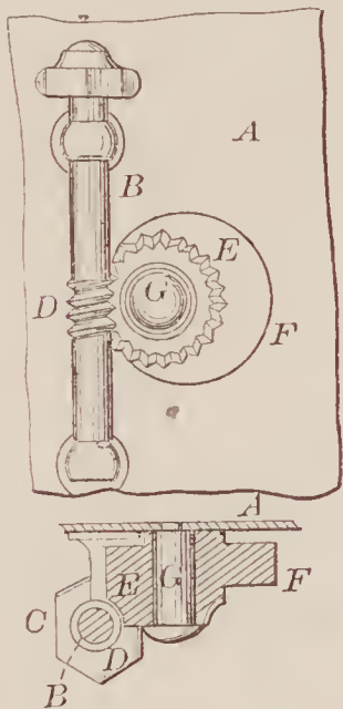
67802—E. Robinson— Wagon.
