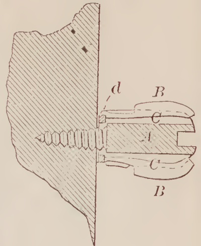
69959—J. Barelay— Carriage Knob.
