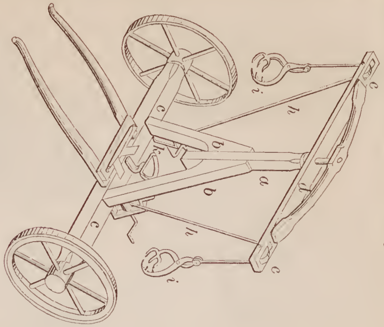
70189—Forshee & McCland—Hay Stacker.
