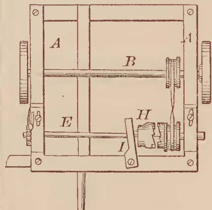
72756—T. E. Platt—Harvester.
