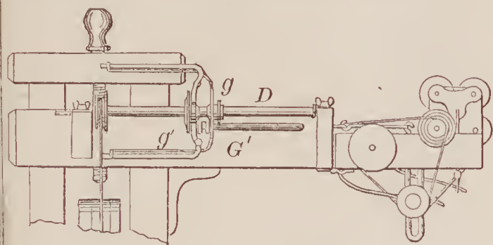
69728—F. Voegtli—Spinning Machine
