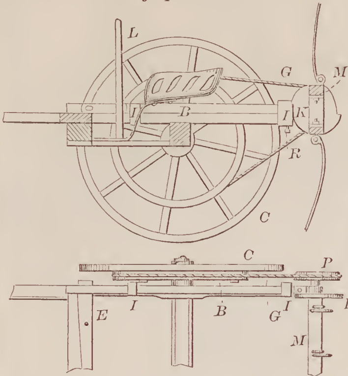
67221—Seymour & Taylor— Horse Rake and Hay Spreader.
