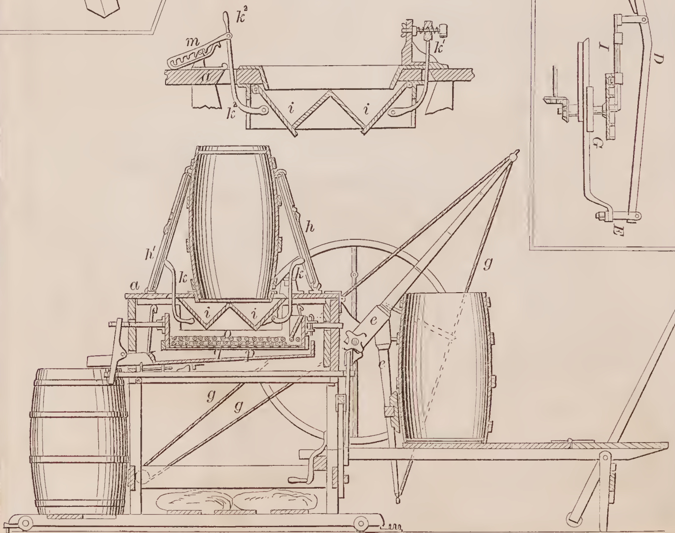
71328—J. J. Rink—Sifting Machine.
