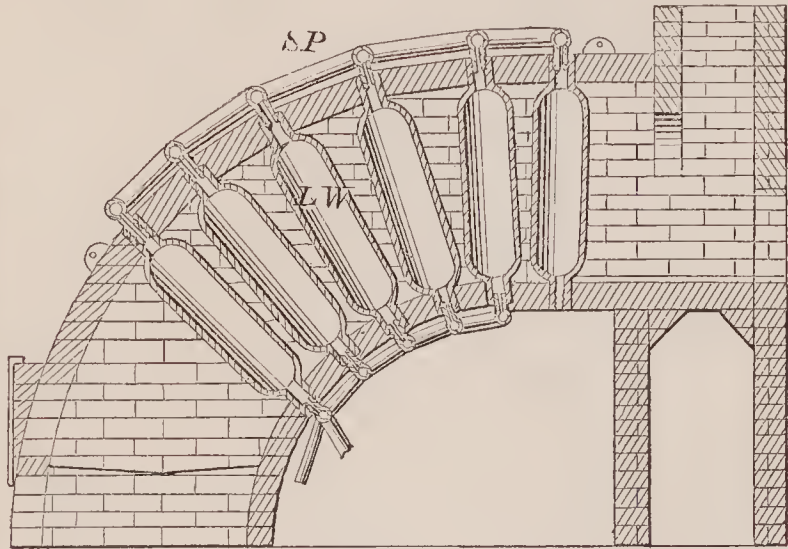
71903—I. R. Oakford— Steam Generator.
