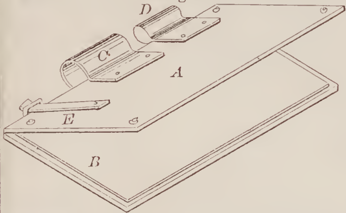
69616—J. E. Billings— Automatic Blotter.
