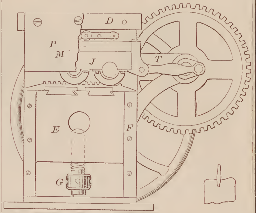
66901—M. H. Spaulding— Churn.
