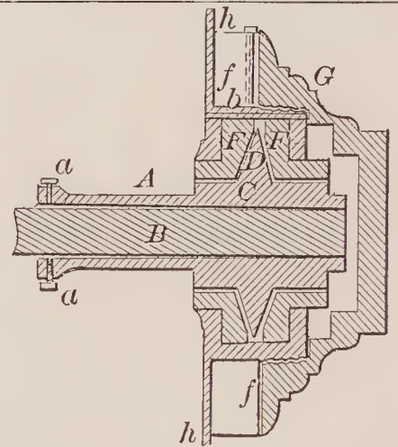
69761—G. E. Burt—Hay Spreader.
