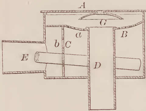
70037—A. F. Smith—Ventilator.
