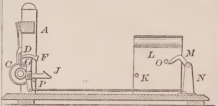
70402—H. D. Briggs— Spinning Jack.
