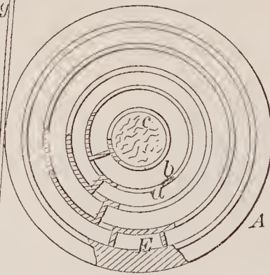
67283—C. H. Frost—Base Burning Stove.
