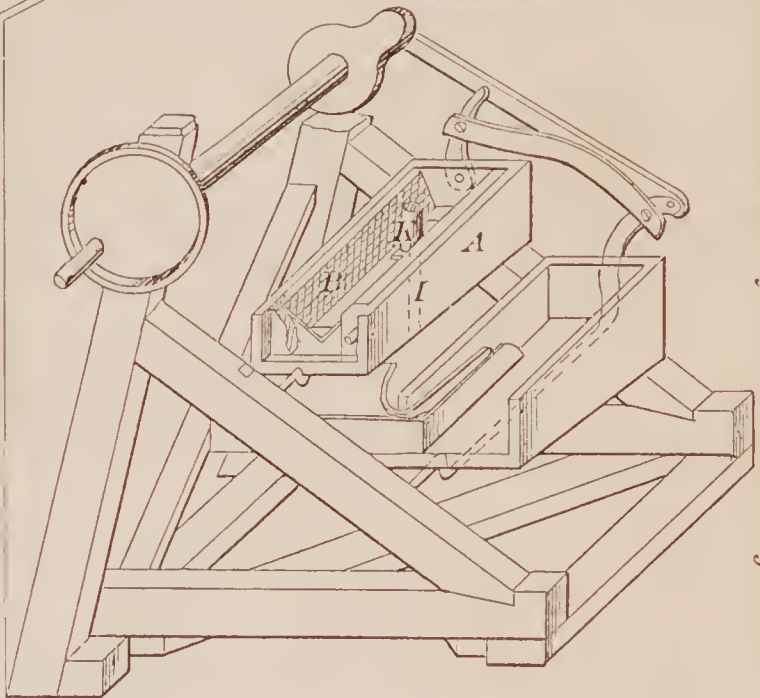
69030—N. S. Ryder—For Washing Ores.
