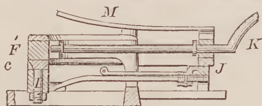
71807—W. H. Staats— Railroad Switch.
