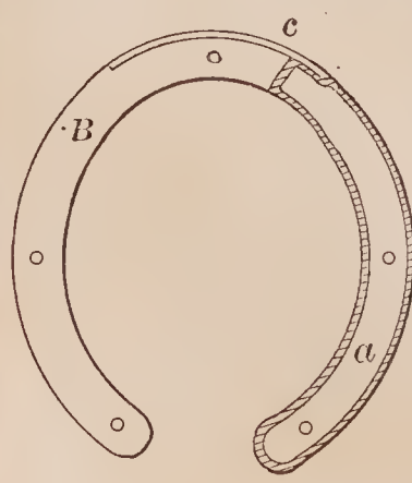
69146—A. S. Wilkenson—Horse Shoe.
