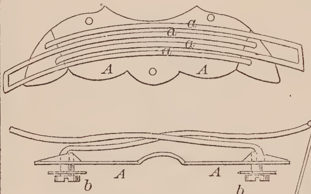
68988—T. A. Huffer—Rein Holder.
