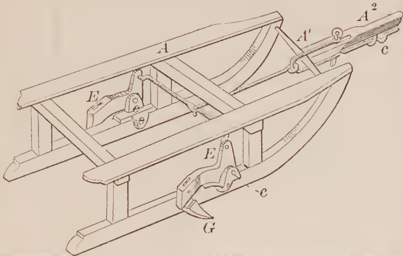
70828—E. K. Gardner— Railroad Gate.
