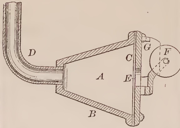
70471—A. R. & N. B. Reynolds— Tempering Steel.
