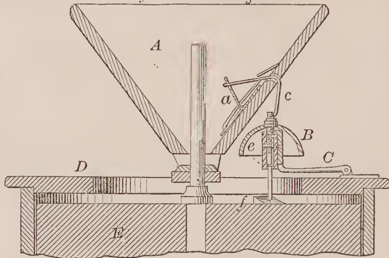
68539—C. N. Taylor—Grinding Mill.
