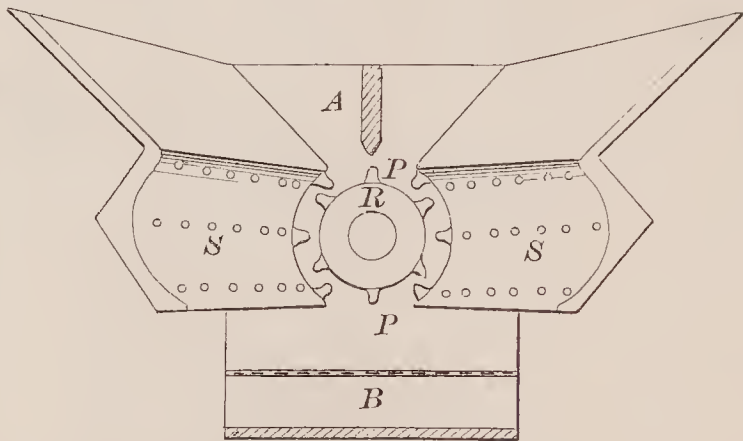
71273—W. H. Bridgens— Pea Sheller.
