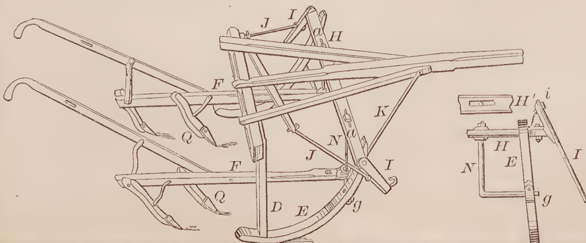
70111—E. Peck— Cultivator.
