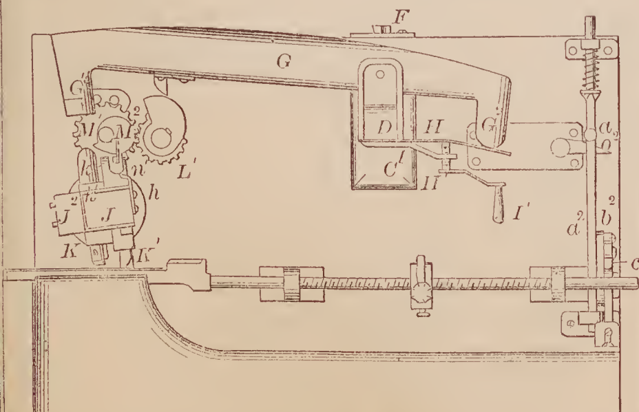
68946—E. Bucklin, Jr.— File Cutting Machine.
