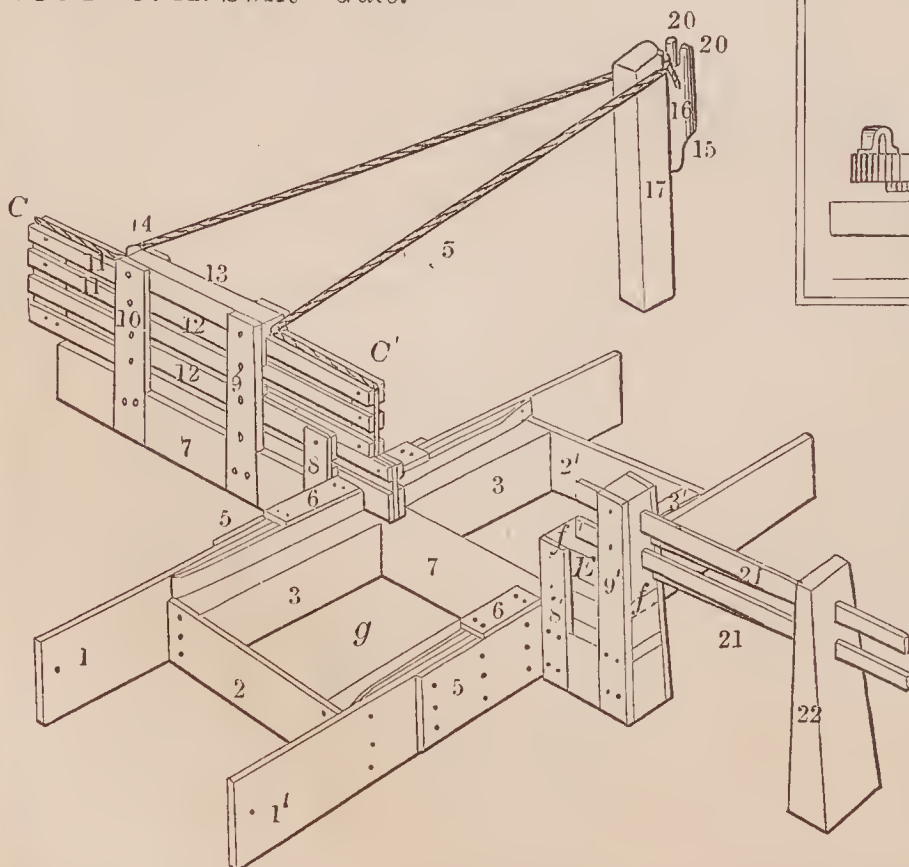
68804—J. M. Swift—Gate.
