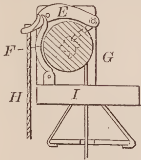
66995—G. F. Smith—Venetian Blind.
