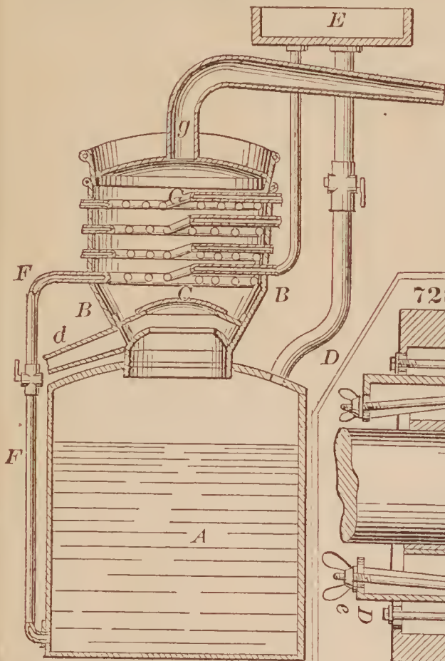
72816—H. G. Dayton—Spirit Still.
