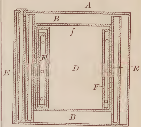
70390—E. H. Ashcroft— Safe.
