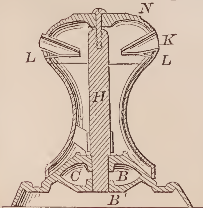
70820—J. Edson—Capstan.
