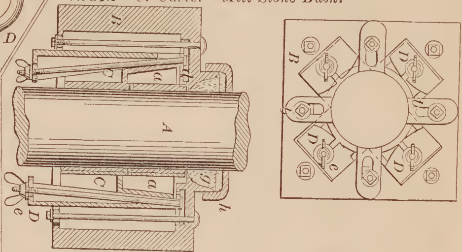
72821—L. A. Dochez—Axle Box.
