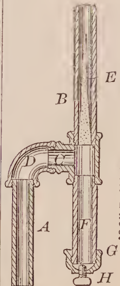
72359—M. L. Bassett—Well Tube.
