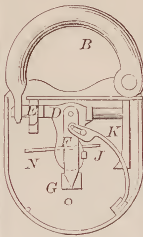
68527— W. H. Murphy— Padlock.
