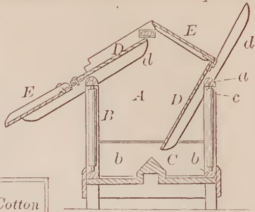
68150—B. F. Barker—Butt Hinge.
