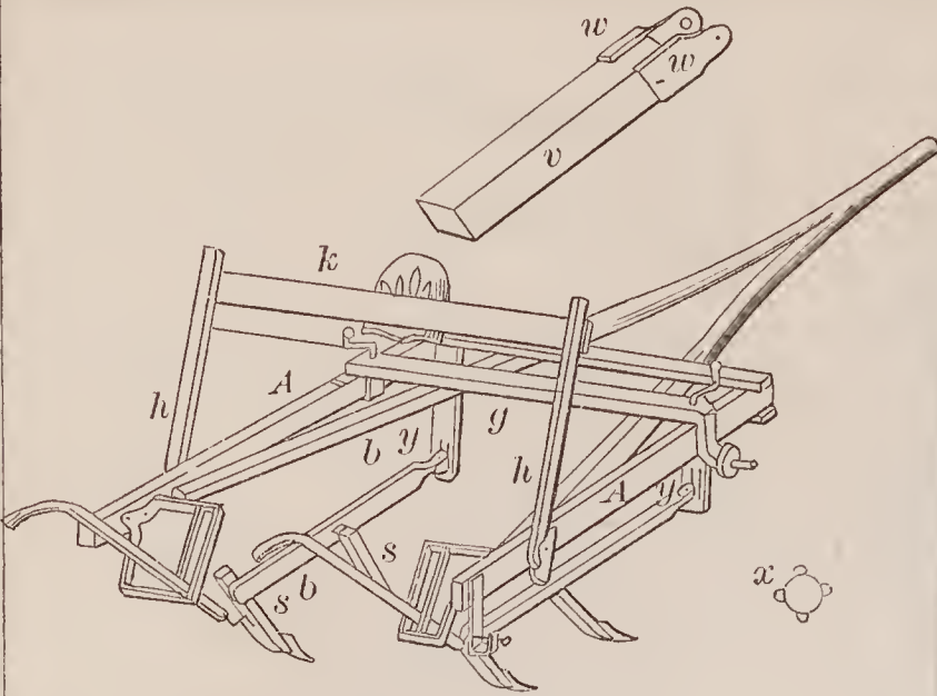
67173—W. A. & C. E. Dryden—Cultivator.
