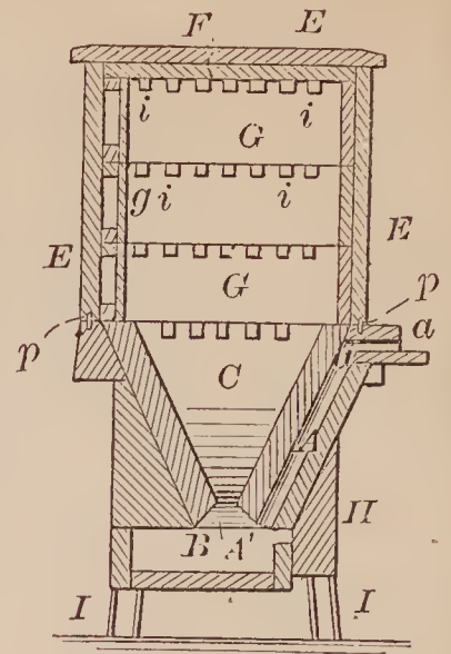
72918—L. & A. M. Shafer—Beehive.
