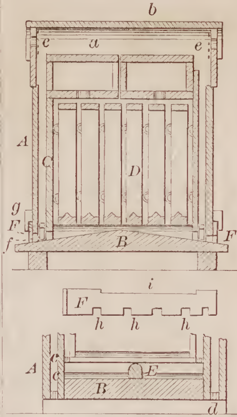
71385—C. H. Haskins—Car Ventilator.
