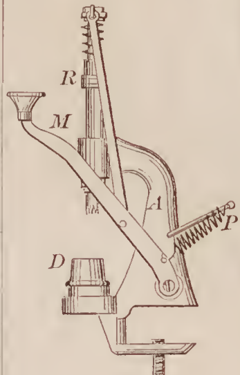
71069—S. A. Russell—Fruit Seeder.
