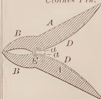
68510—J. P. R. James— Clothes Pin.
