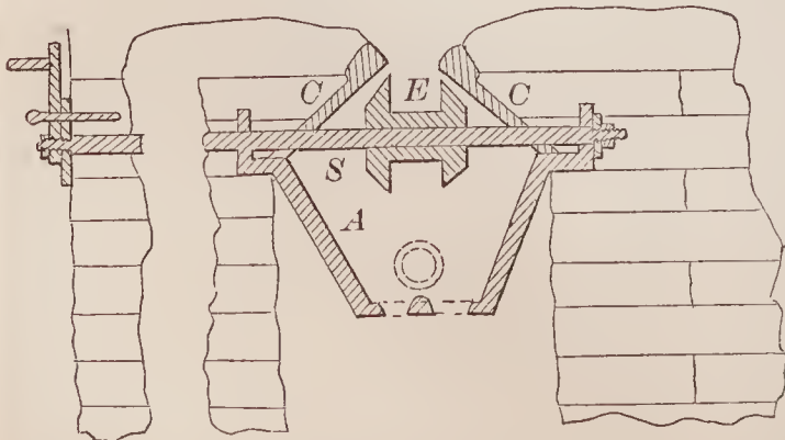
69973—J. W. Crannell—Tuyere.
