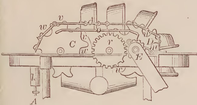
68753—A. H. Knapp— Water Elevator.
