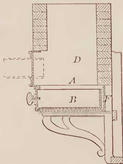
72151—E. S. Phelps, Jr.—Chimney.
