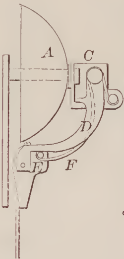
71627—D. Liebrich—Door Gong.
