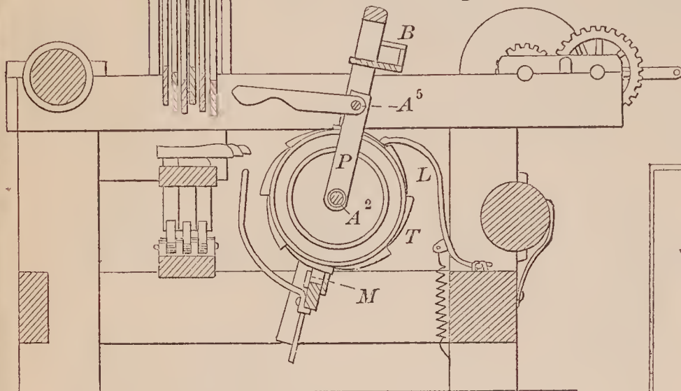
68969—T. A. Dugdale—Hand Loom.
