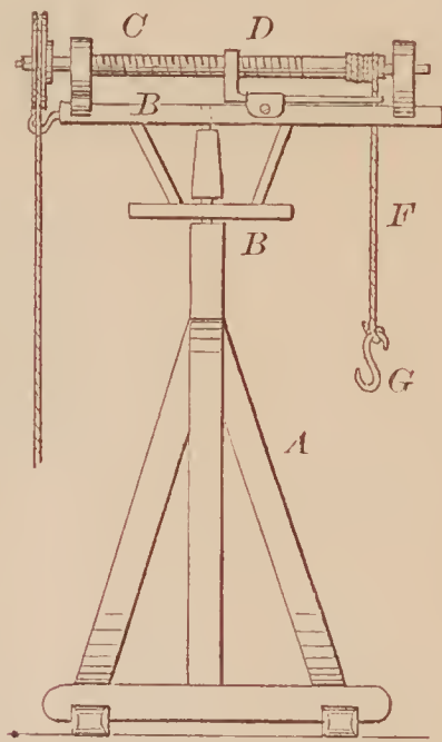
72801—J. S. Coffman— Rotary Crane.
