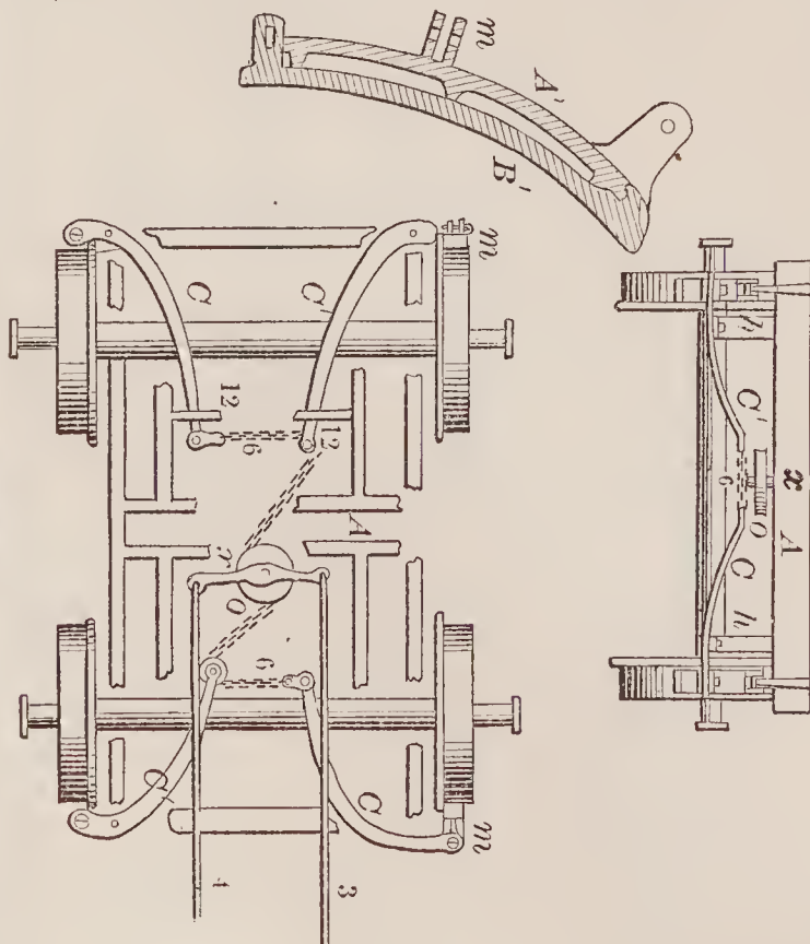
71591—Dunham & Widney—Car Brake.
