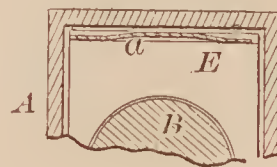
72821—L. A. Dochez—Axle Box.
