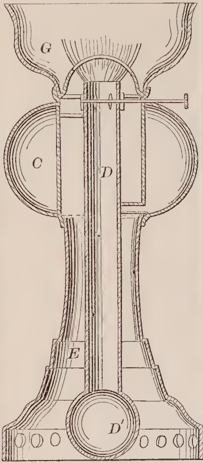
71268—G. A. Beidler— Lamp.
