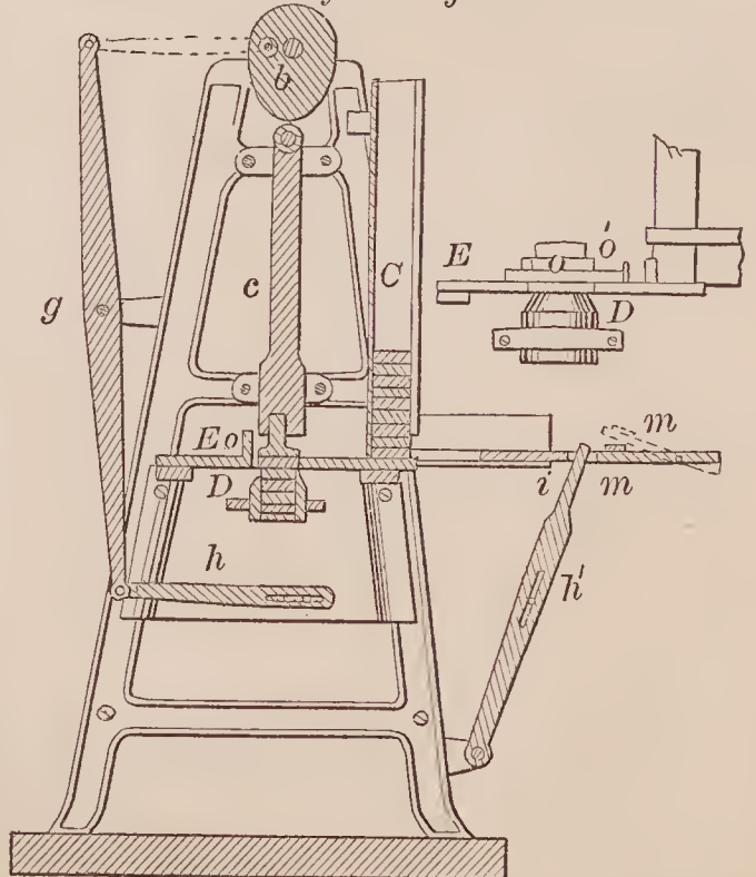
72505—J. Kirby— Bung Cutter.
