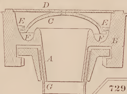
72909—J. S. Rogers—Sink Trap.
