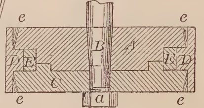
68989—N. Hunt—Engine Piston.
