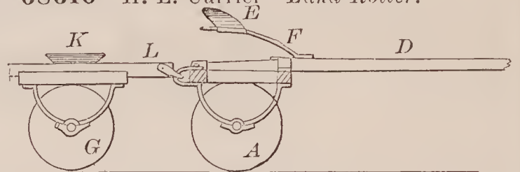
68610—H. L. Currier—Land Roller.
