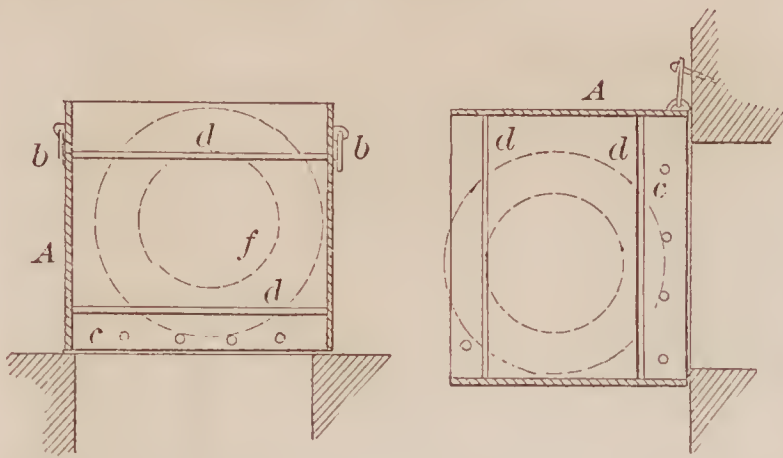
68231—G. H. Peacock—Carbureting Apparatus.
