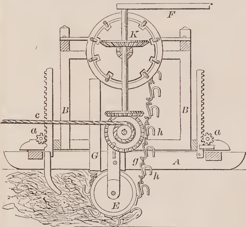
72140—A. H. & T. S. Whitacre—Ditching Machine.
