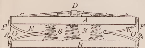
71014—H. L. Huntington— Spring Bed Bottom.
