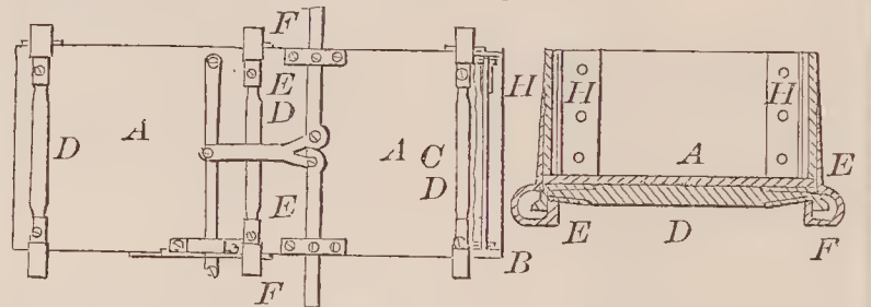
66882—D. H. Peterson—Wagon Box.
