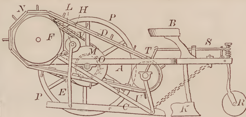
68309—N. S. Noyes—Potato Digger.
