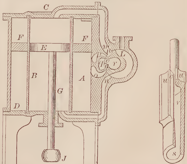
66975—J. L. Lay— Steam Engine.
