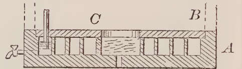
67283—C. H. Frost—Base Burning Stove.
