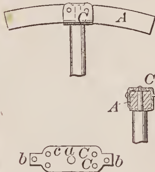
69757—R. Brooks, Jr.—Carriage Wheel.
