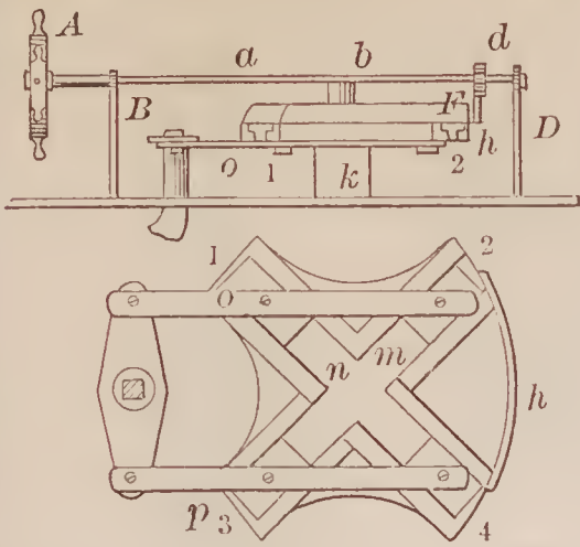
70255—J. Perkins— Steering Apparatus.
