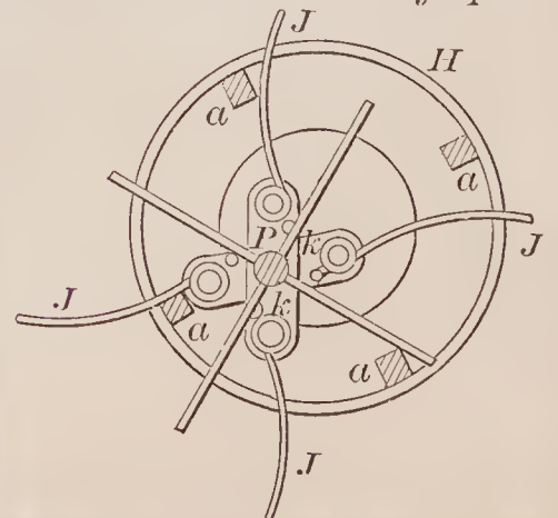
69761—G. E. Burt—Hay Spreader.
