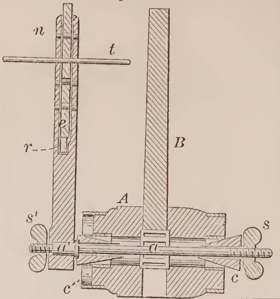
69287—W. S. Weed—Reversible Butt Hinge.
