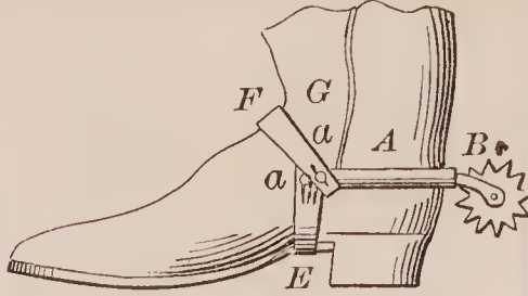
71462—B. A. Davis— Spur
