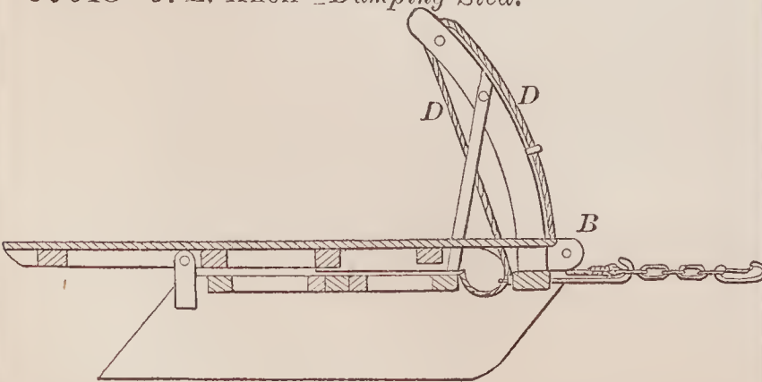
69918—J. L. Knoll— Dumping Sled.
