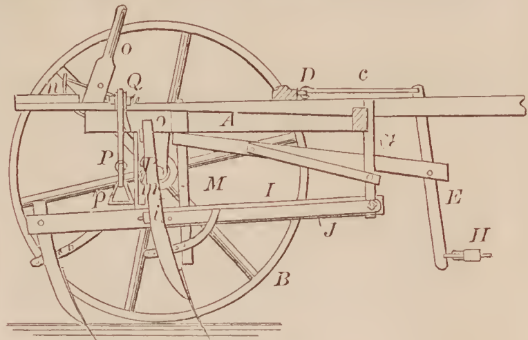
67093 —J. Wilson— Cultivator.
