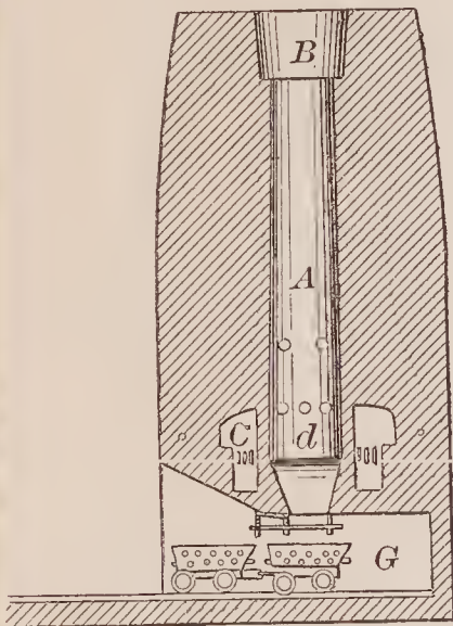
70234—J. L. Livingston—Lime Kiln.
