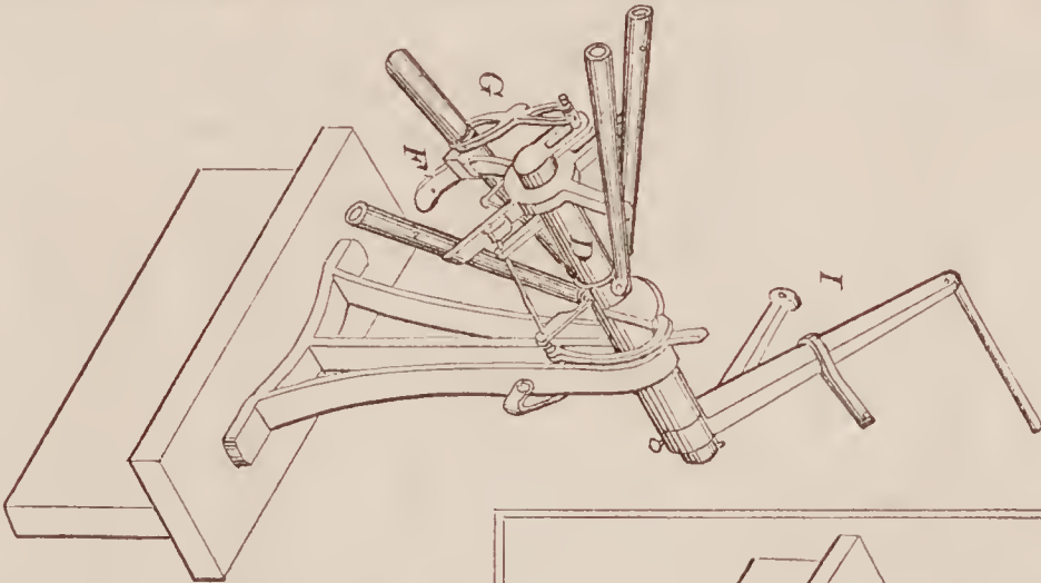
72198—H. A. M. Harris— Harvester Rake.
