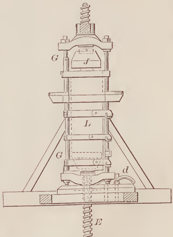
67230—D. R. Torbet— Cotton Press.
