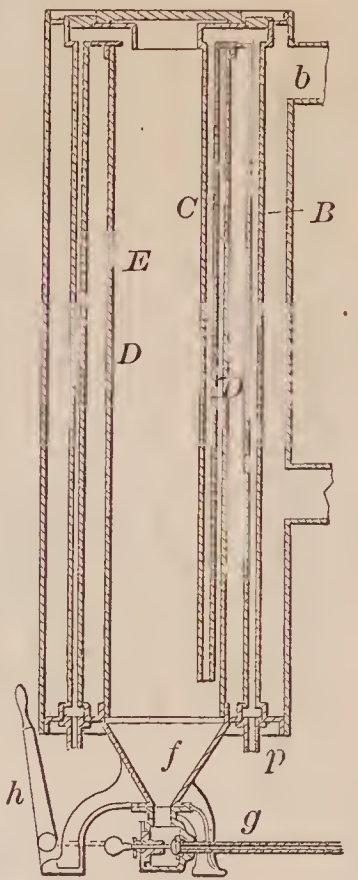
68435—D. M. Graham—Gas Apparatus.
