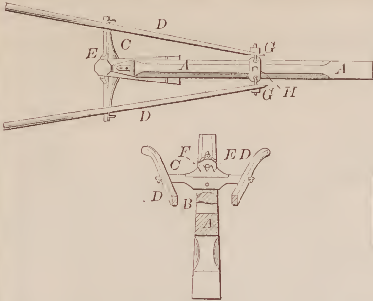
72087—J. H. Rowley—Churn.
