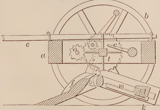
67148 —J. M. Wilcox— Potato Digger.
