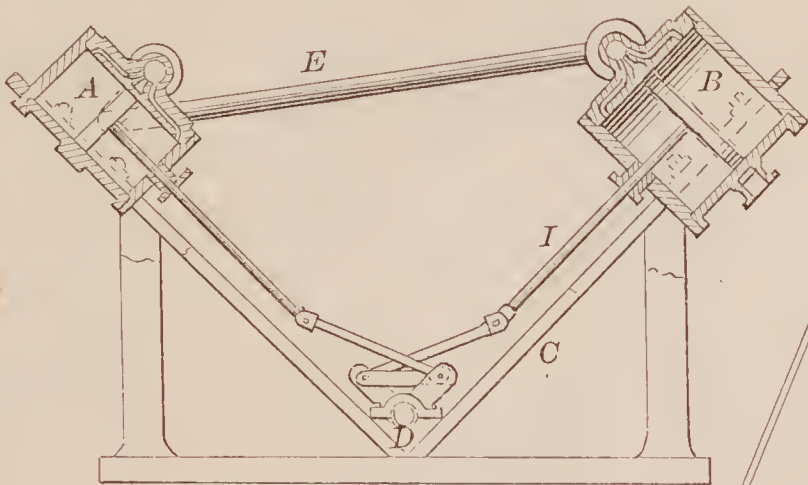
66973—J. L. Lay— Steam Engine.
