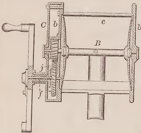
71344—J. Vom Hofe—Fishing Reel.
