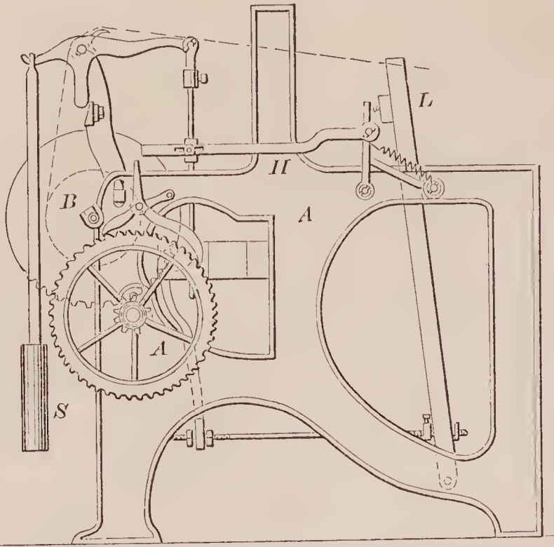
72236—H. L. Smith— Corn Harvester.
