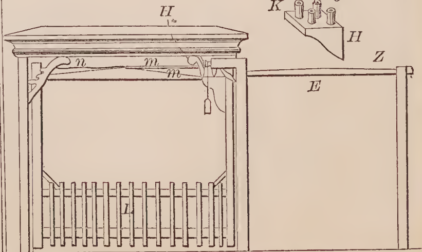
72495—H. Hunt— Gate.
