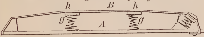
72398—P. C. Ingersoll—Spring Bed Slat.
