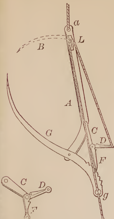
68873—L. Haverstick— Horse Hay Fork.
