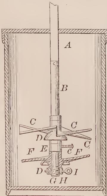
68560—J. E. Finley—Churn.
