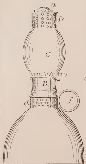
70931—M. B. Wright—Lantern.
