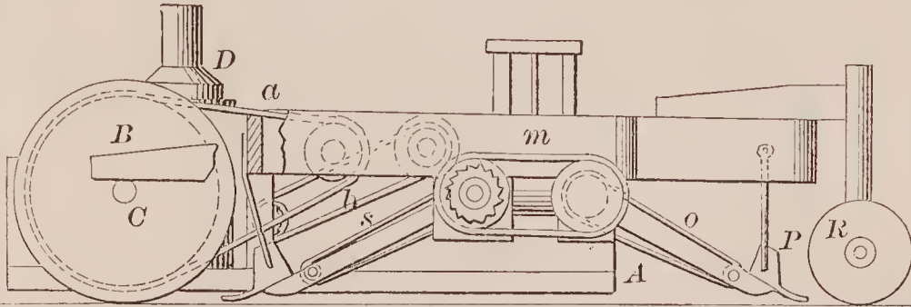
72336—B. T. Stowell—Excavator.
