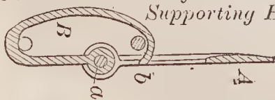
67681—J. H. Snyder—Hame Clasp.
