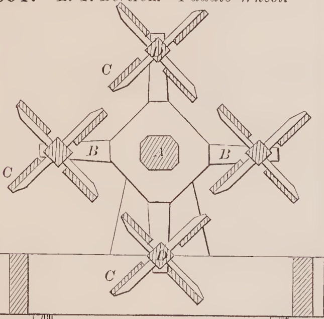
70947—E. T. Bostrom—Paddle Wheel.
