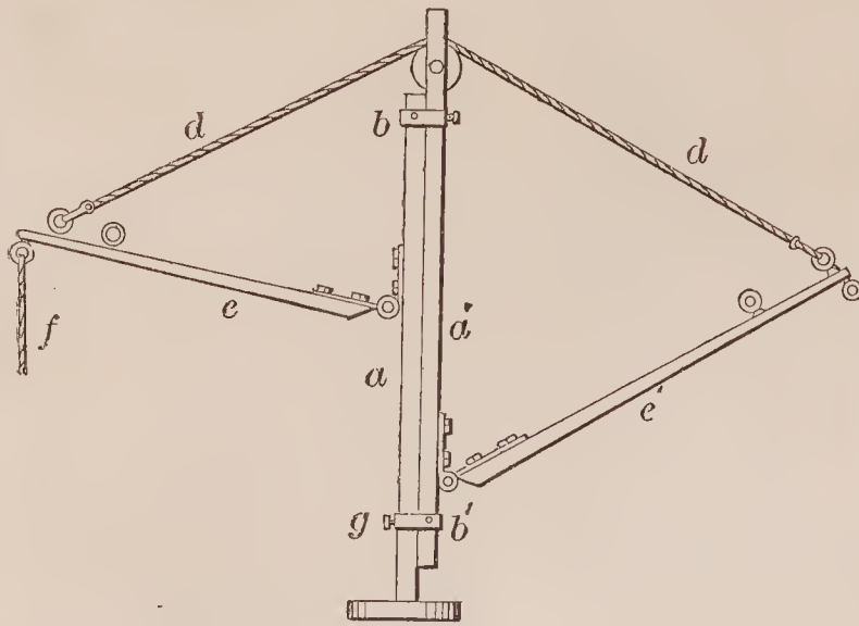
69378—E. H. & D. R. W. Williams—Excavating Machine.
