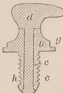
69306—W. P. Bateman— Carriage Button.
