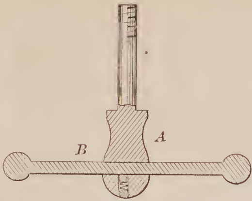
72327—H. K. & T. W. Porter—Vise.
