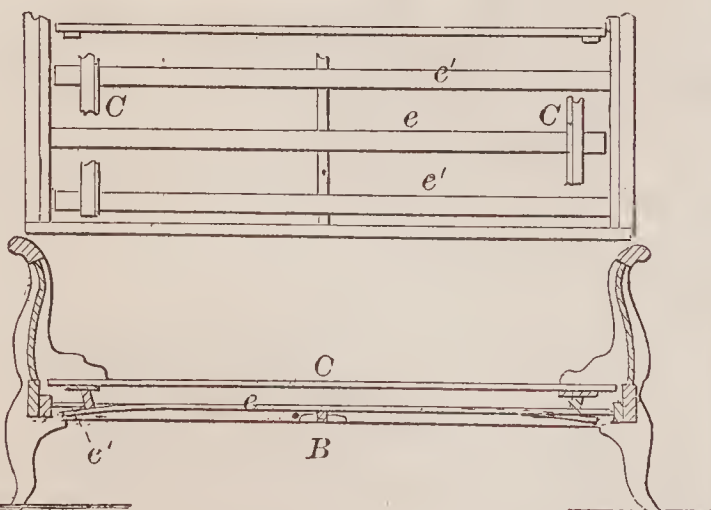
67521—H. A. & A. Follett— Bed Bottom.
