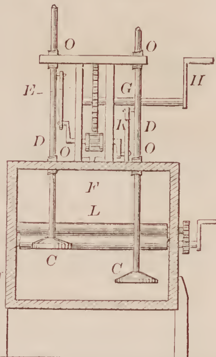
72281—T. Q. Frost—Washing Machine.
