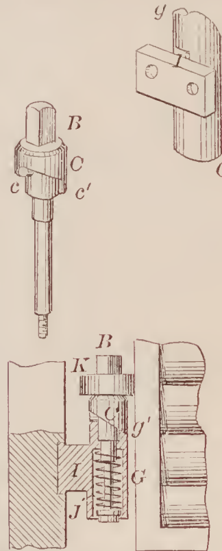
70922—A. S. Villec— Clamp for Harness Frames.
