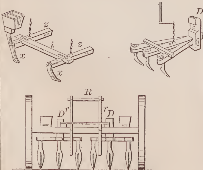
68056—R. N. Ely—Cultivator.
