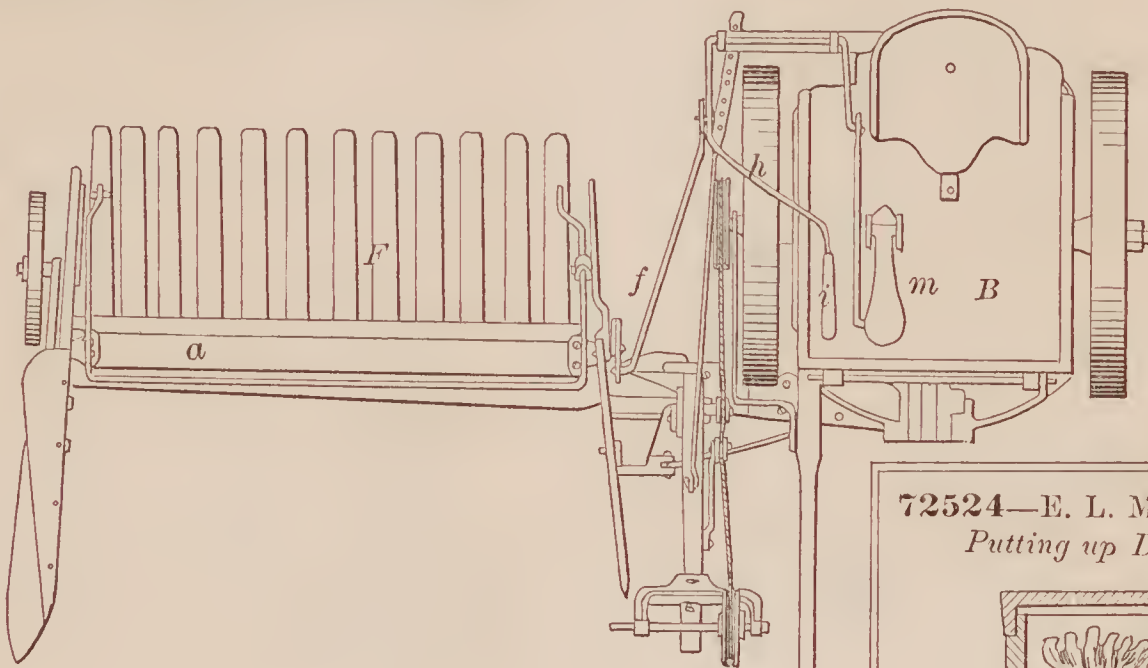
72523—J. Miller— Harvester Dropper.
