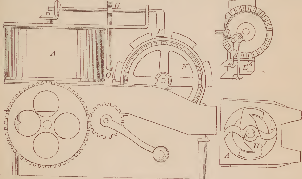
68894—J. M. Moyer—Brick Machine.
