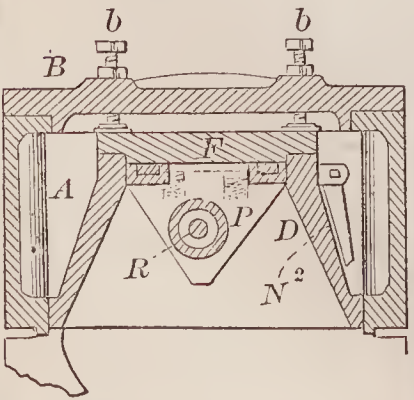
67302—G. H. Hoagland—Slide Valve.
