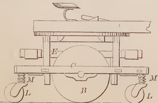
70739—E. F. Olds—Land Roller.
