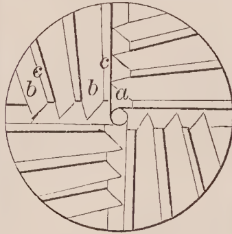
72259—J. R. Adams—Coffee Mill.
