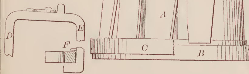
70739—E. F. Olds—Land Roller.
