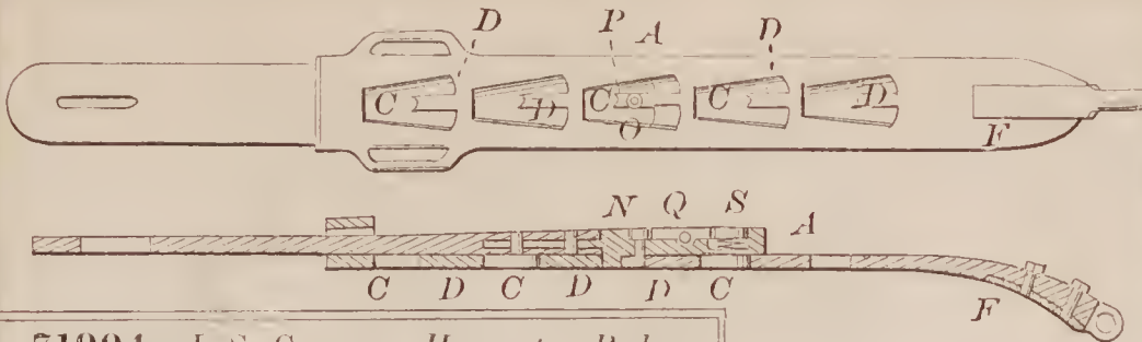
71994—J. S. Crump—Harvester Rake.
