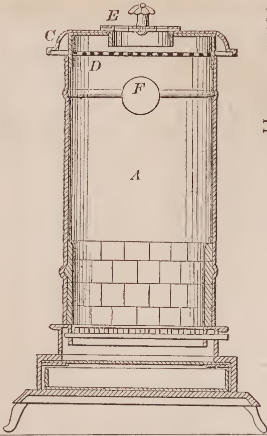
69246—J. H. Quackenbush—Washing Machine.
