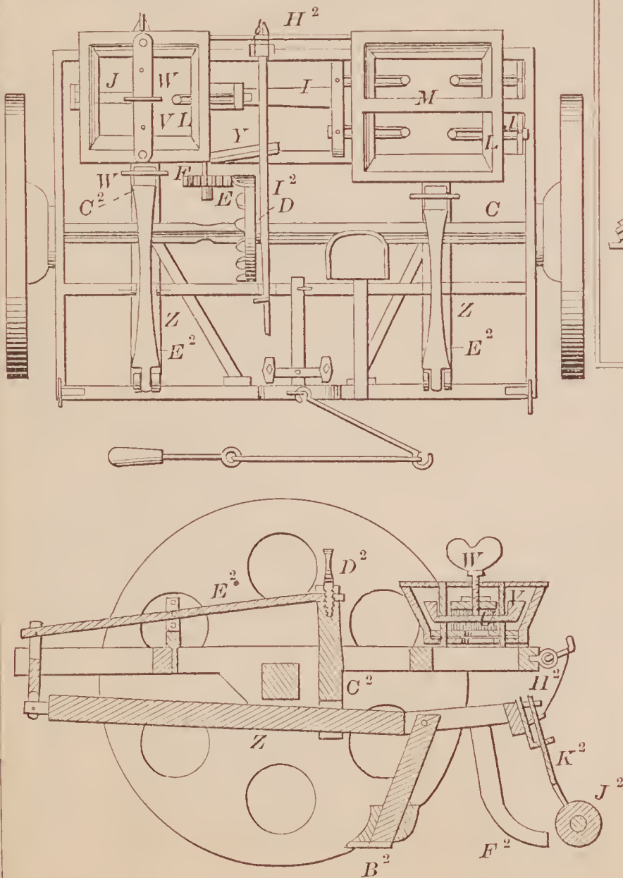
72472—J. K. Frantz—Seed Planter.
