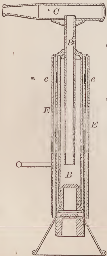
69578—N. Page, Jr.—Pump.
