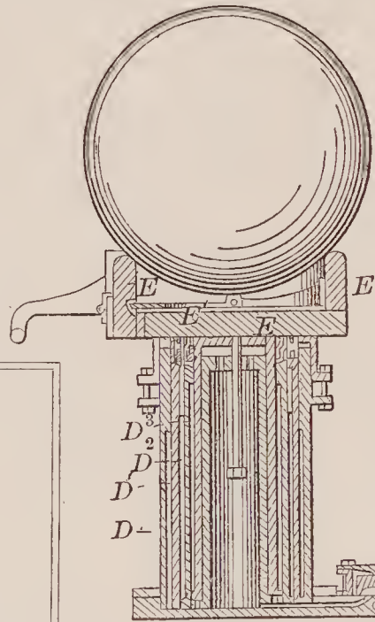
71593—K. Ebermeyr—Melodeon.
