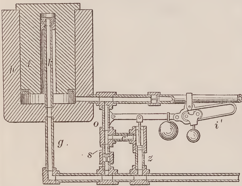
67719—J. T. Burr— Hydraulic Press.
