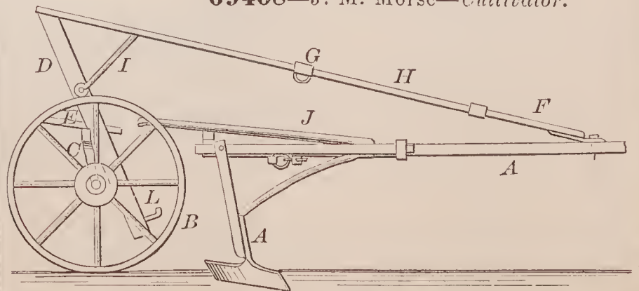
69468 —J. M. Morse— Cultivator.
