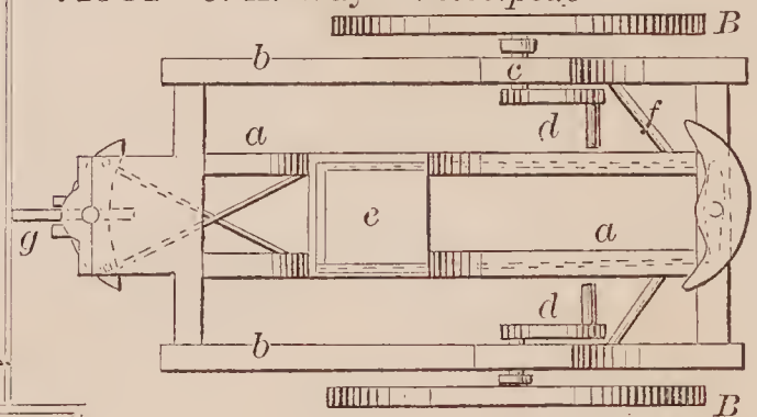
71561—C. A. Way— Velocipede
