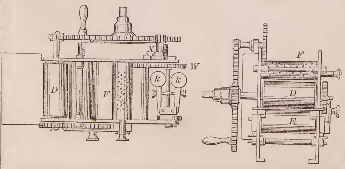
71103—J. M. Willbur—Printing Apparatus.
