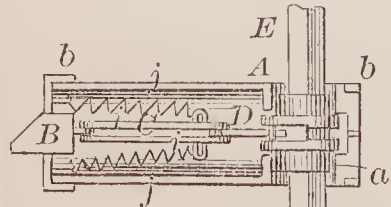
67795—G. H. Palmer— Mortise Knob Latch.
