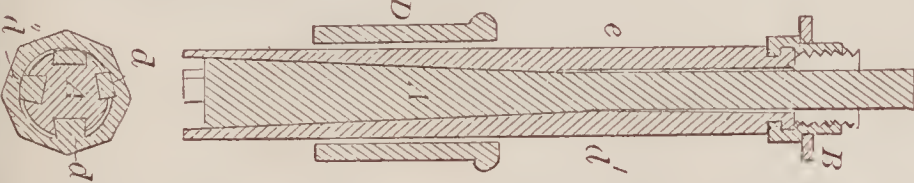
67711—C. C. Blodgett—Horse Hay Fork.
