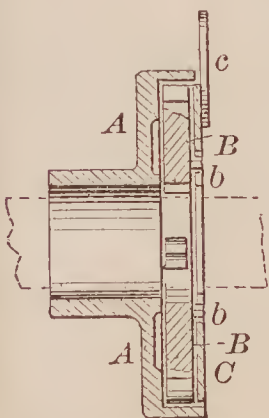
69184—W. T. Cole— Chuck.
