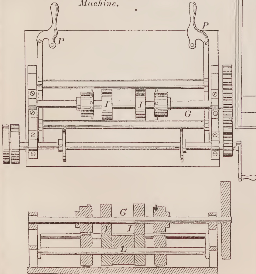
69991—J. H. Haskell—Leather Punching Machine.
