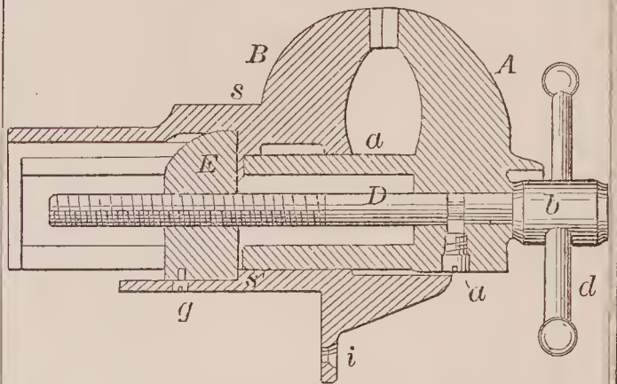
69361—J. H. Murray— Vise.
