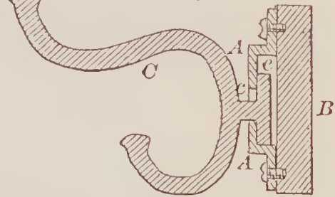
69587—S. S. Putnam— Clothes Hook.
