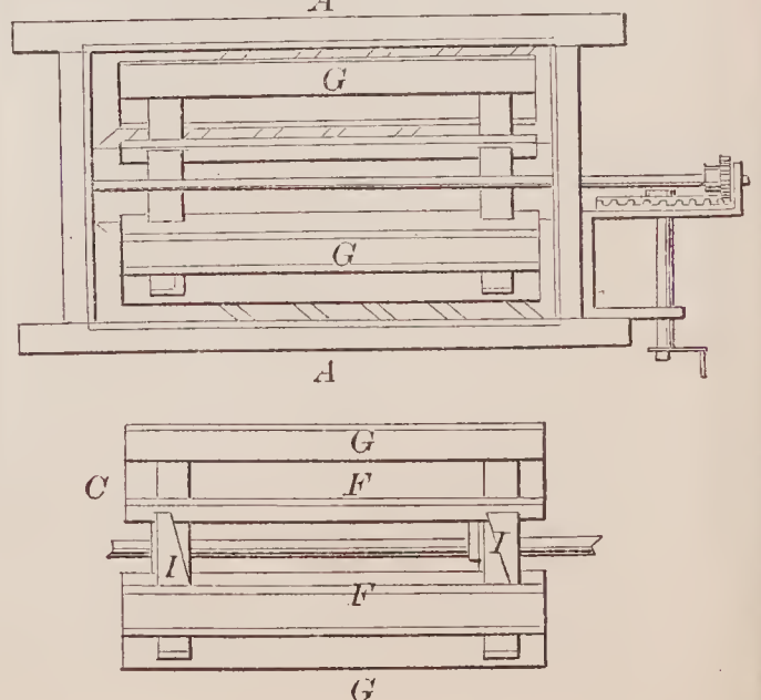
69855—I. H. Spelman— Churn.
