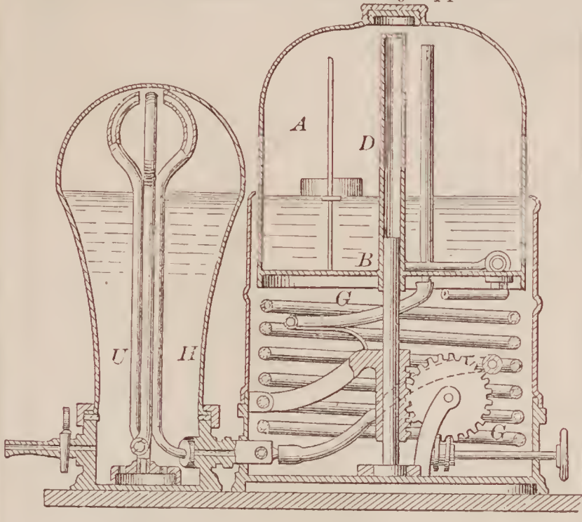
68231—G. H. Peacock—Carbureting Apparatus.
