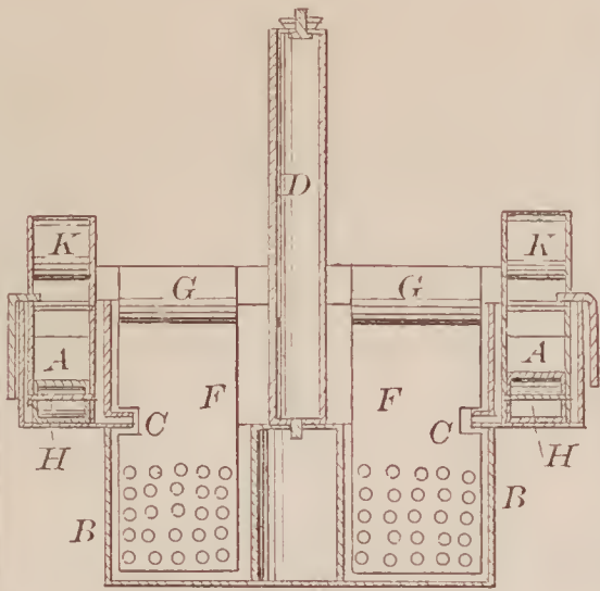
68175—G. B. Field— Amalgamator.
