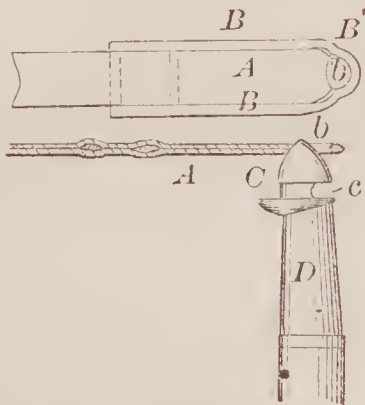
67967—G. W. Fink— Trace Fastener.
