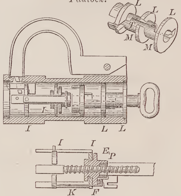
69645—B., J., S. B & A. H. Elbert— Padlock.
