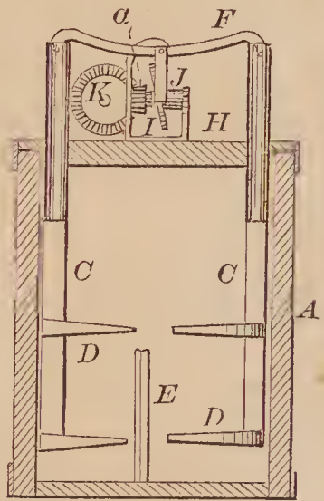
72588—H. B. Barber— Churn.
