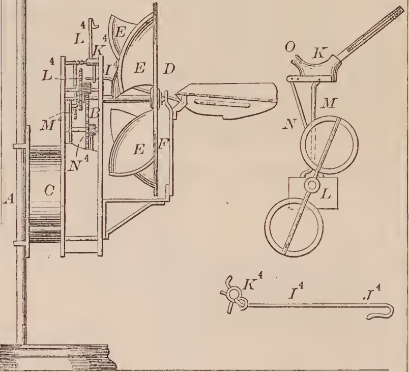
68483—J. & A. Bloom—House Fan.
