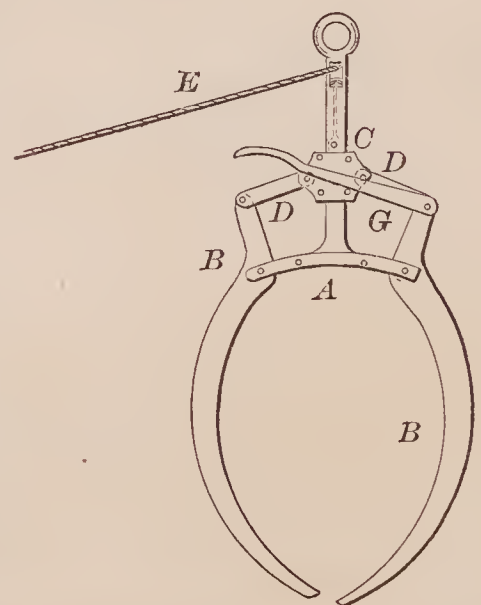
72567—L. N. Tinkham— Horse Hay Fork.
