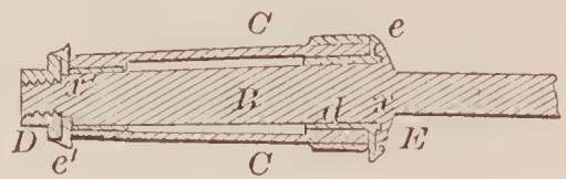
69350—S. D. Littlefield— Axle
