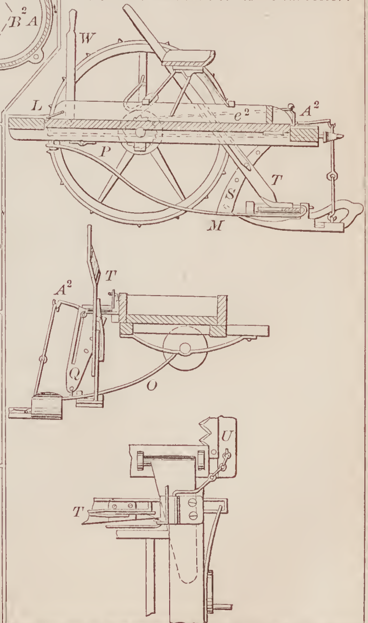
70001—M. A. Keller— Harvester.
