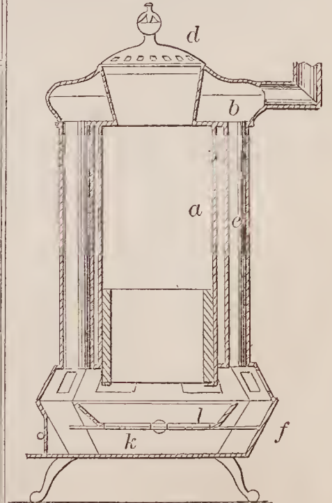
67283—C. H. Frost—Base Burning Stove.
