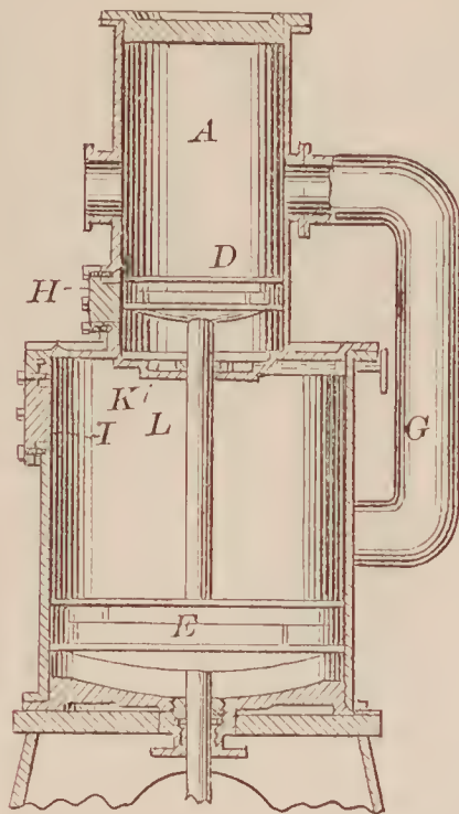
66971—J. L. Lay— Steam Engine.
