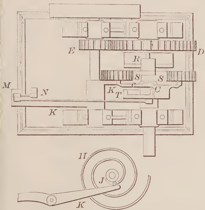
71162—J. Hall— Toy Pistol.
