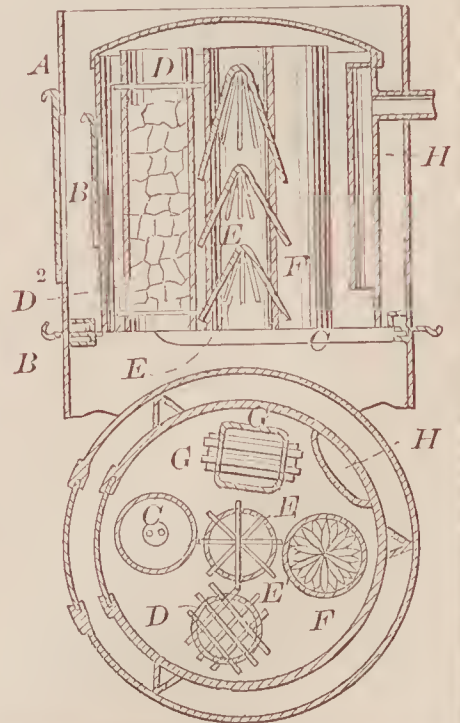
66862—M. S. Marshall—Gas Stove.
