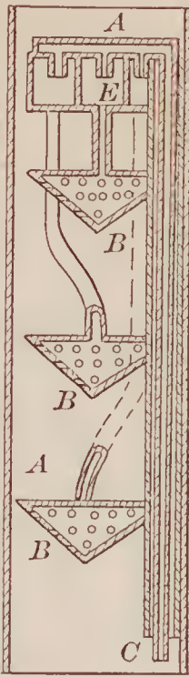
70389—E. H. Ashcroft— Condenser.
