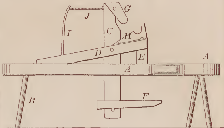
68272—D. Williams—Corn Husker.
