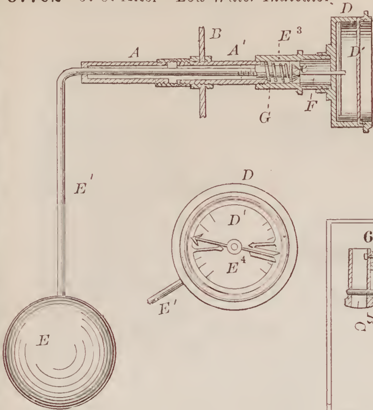
67702—J. O. Alter—Low Water Indicator.
