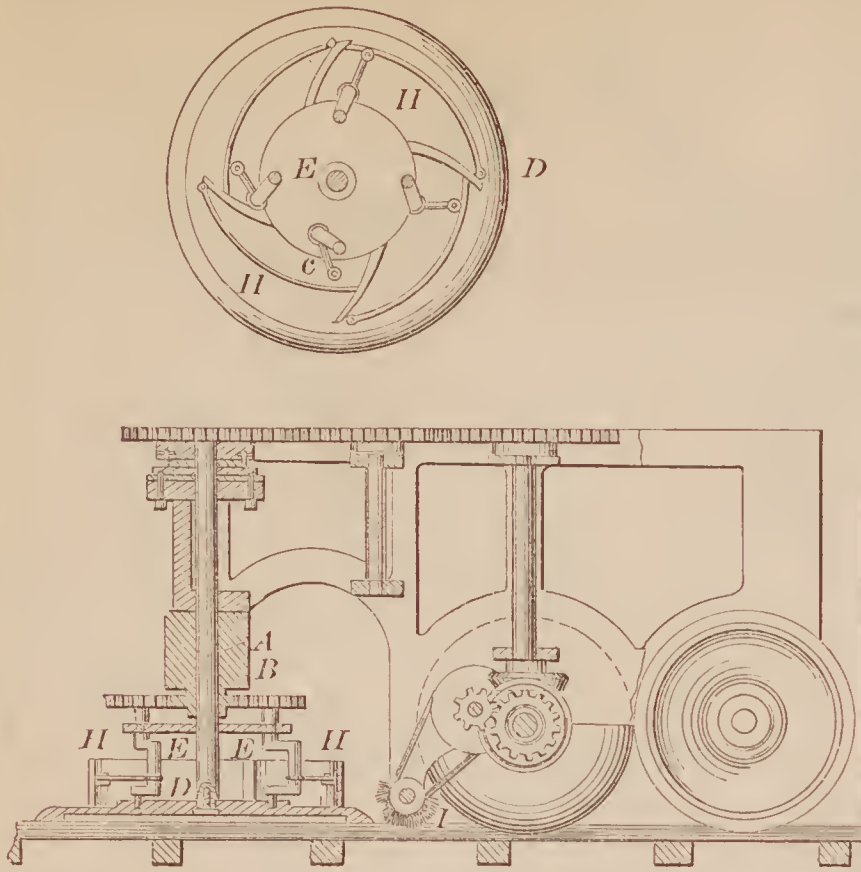
72439—E Abbiati—Track Clearer.
