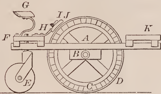
69175—G. R. Burt—Land Roller.
