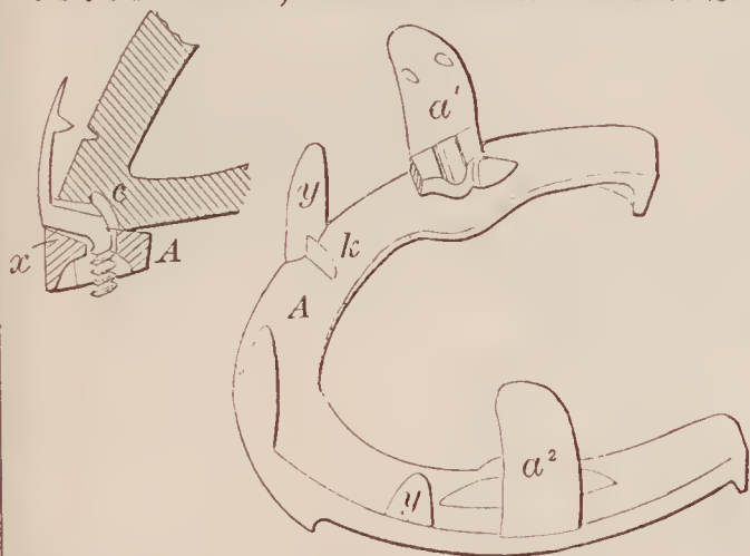
70783—Behel, Perrine & Buell—Horse Shoe.
