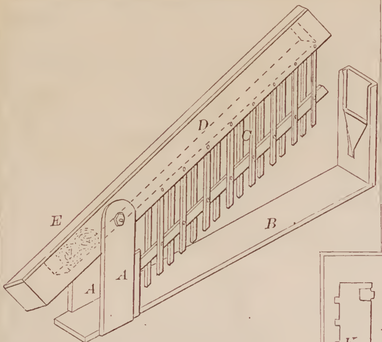
68687—J. Beck—Ticket Punch
