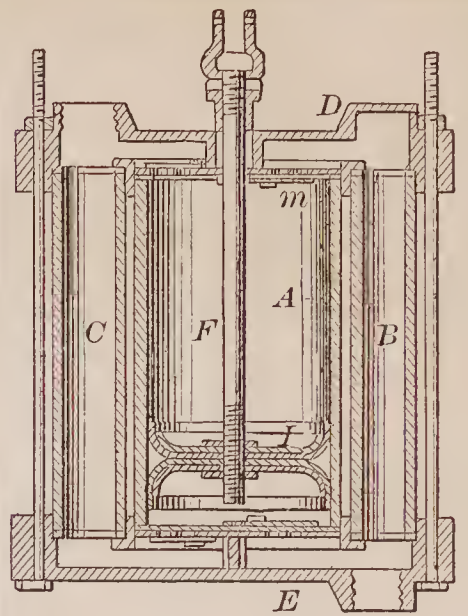
70379—H. Tyler— Pump.
