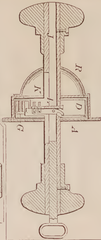
72347—J. Wertsbaenger—Locking Knob Latch.
