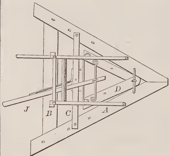
72623—J. T. Frankeberger—Harrow.
