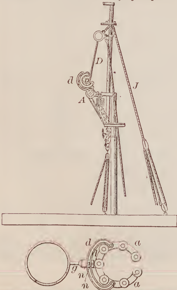
67546—F. Höök—Eor Reefing Top Sails.
