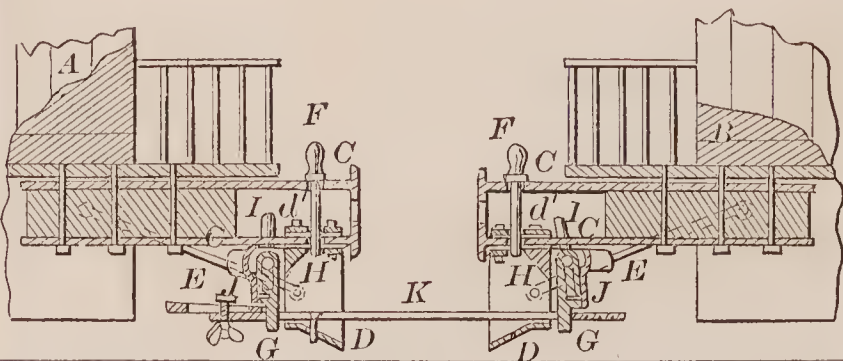
72203—M. G. Imbach—Car Ventilator.
