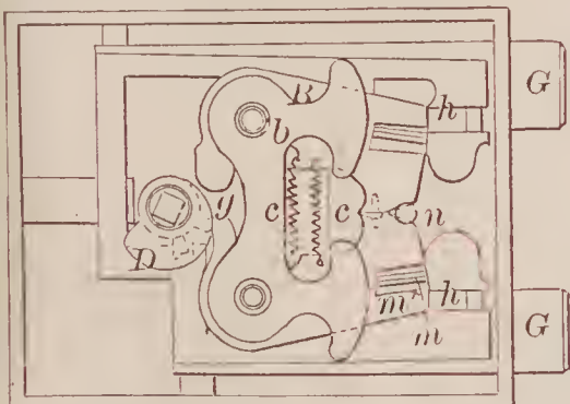
68334—Allen & Brady— Door Lock.
