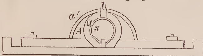
70397—M. Blakey— Skelping Die.
