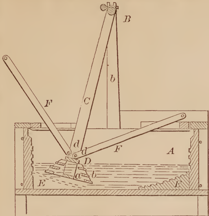
72816—H. G. Dayton—Spirit Still.
