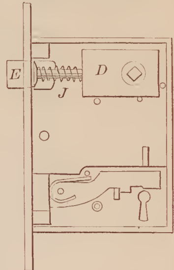
72946—R. L. Webb—Reversible Latch.
