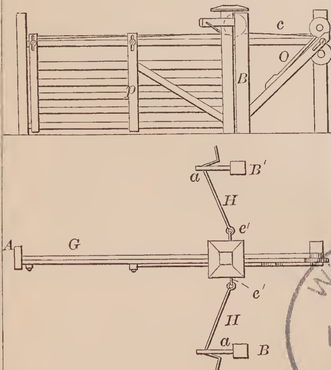
72957—I. N. Young—Gate.
