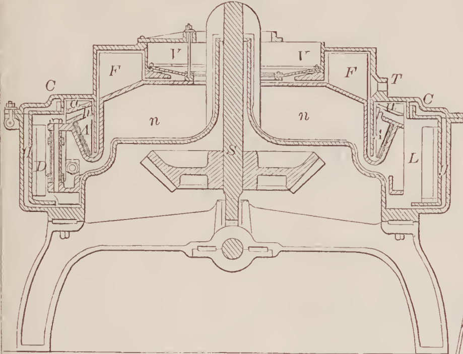
69564—F. G. Hesse— Amalgamator.
