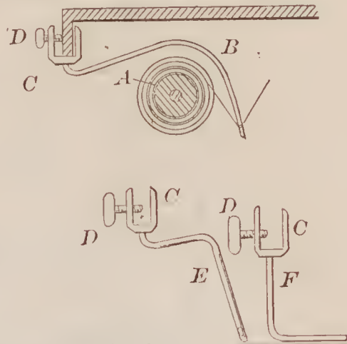
67525—H. S. Frost— Door Spring.
