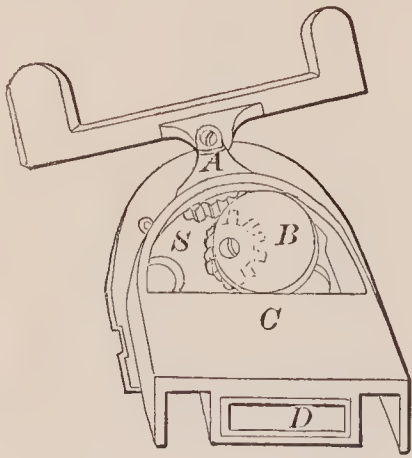
71829—H. Willard—Horse Hay Fork.
