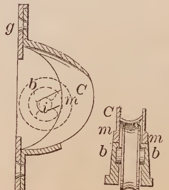
68868—O. S. Garretson—Window Pulley.
