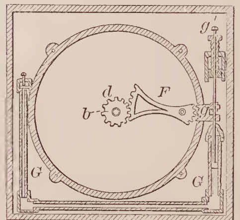
72084—J. T. Buckley—Automatic Register.
