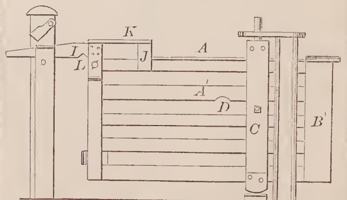
66852—E. Kemper—Gate.
