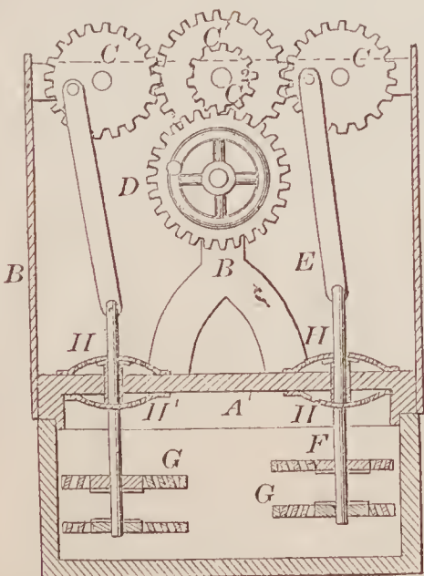
69653—E. L. Gilman— Churn.
