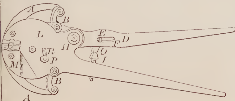
69962—J. Blackinton— Bolt Trimmer.
