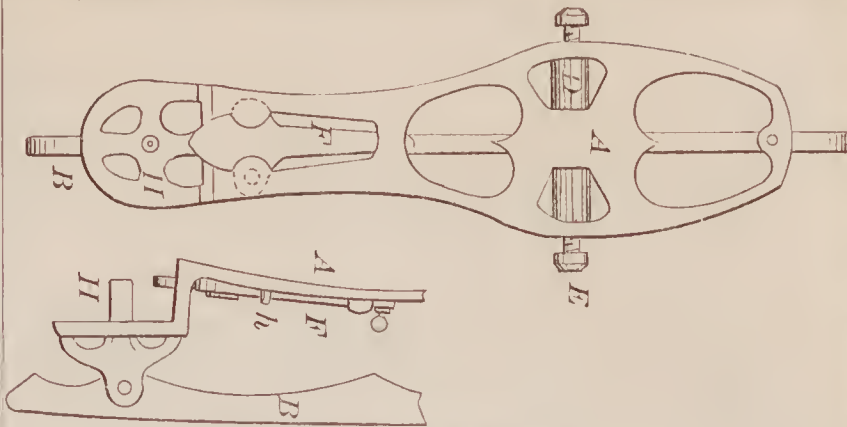
67799—J. W. Post— Skate.
