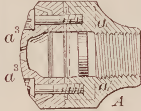
72348—J. M. Wheeler—Steam Jet.
