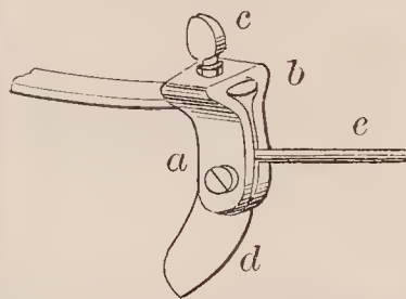
66869—J. E. Morgan— Harrow.
