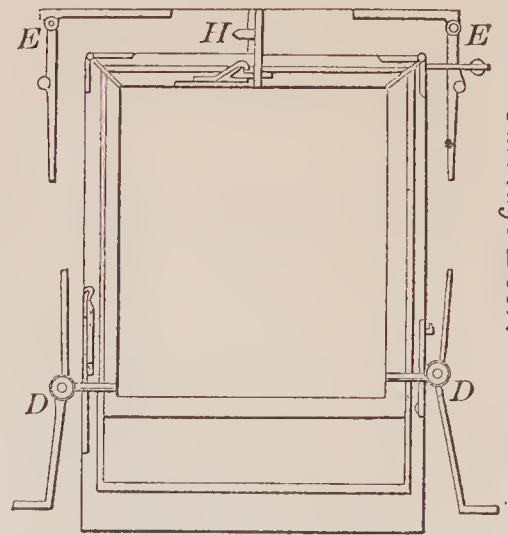
69641—Devillard & Postwieler— Carriage Door.
