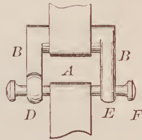
67777—L. Littlejohn— Cotton Bale Tie.
