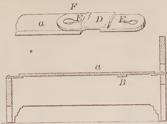
69632—H. M. Conklin—Bed Bottom.
