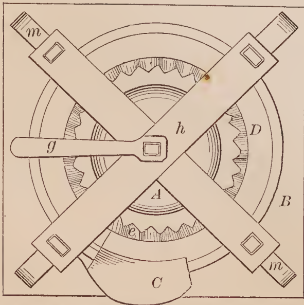
72388—S. Gissinger—For Squeezing Puddled Iron.
