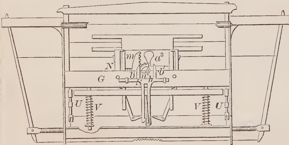
69711—L. Seofield—Loom.
