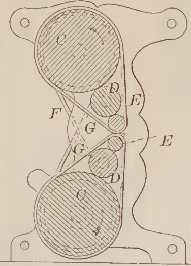
67773— J. W. Kokemuller— Cotton Gin.
