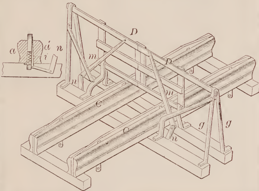
70828—E. K. Gardner— Railroad Gate.
