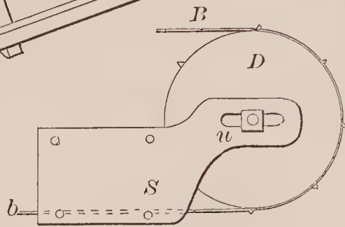
70883—E. & J. S. B. Norton— Dish Washer.
