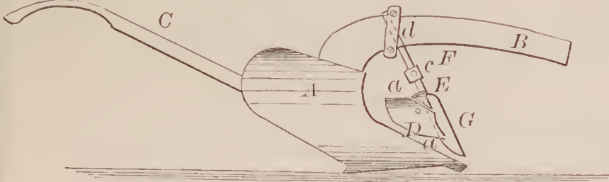
68152—J. S. Beals—Plow.
