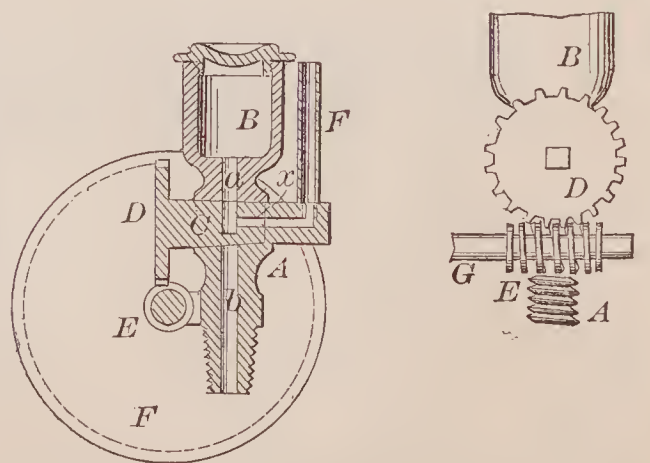
68057—J. G. Edgell—Lubricator for Shafting.
