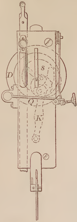
68835—C. F. Bosworth— Sewing Machine.
