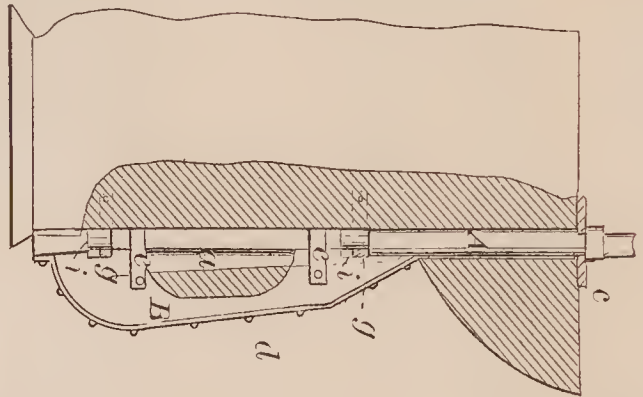
67066—T. W. Murray— Rudder.
