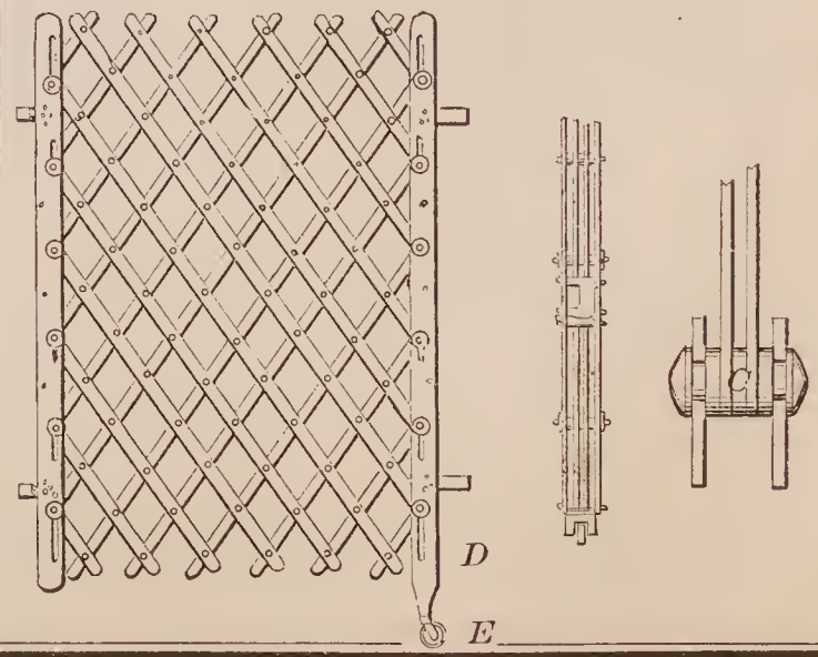
67143—C. S. Snead—Extension Gate.
