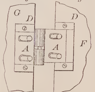
67904—J. G. Ralph— Adjustable Hinge.
