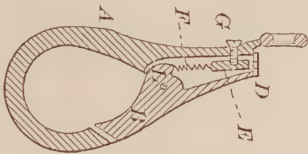
68781—H. S. North— Snap Hook.
