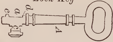
68338—A. G. Batchelder—Lock Key
