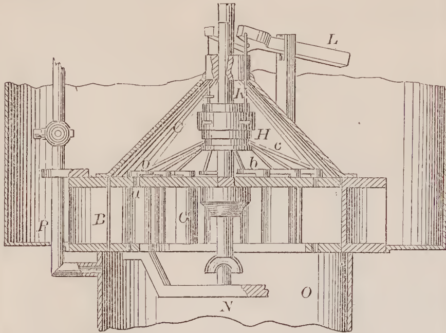
67994—O. W. Ludlow—Water Wheel.
