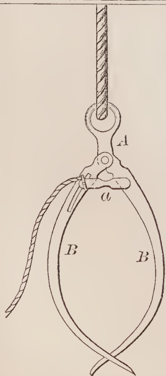
69857—B. F. Stewart— Horse Hay Fork.
