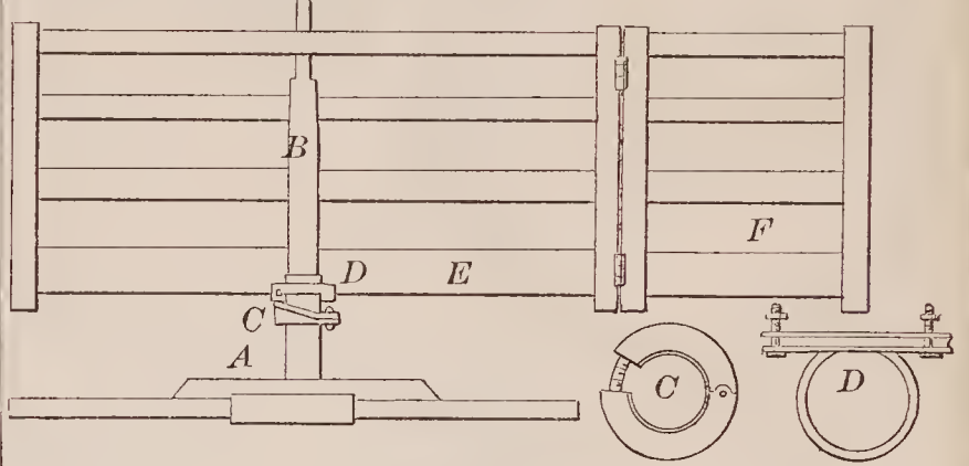
70548—O. Graham—Farm Gate.
