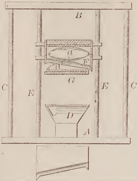
67964—C. L. Eggert— Churn.
