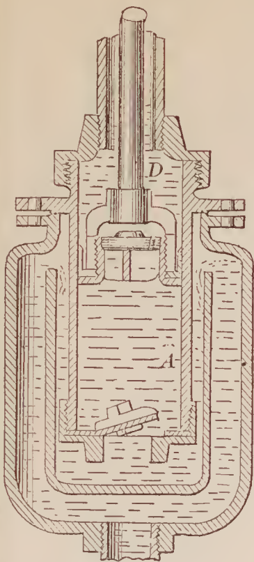
70733—J. H. & T. J. McGowan—Pump.
