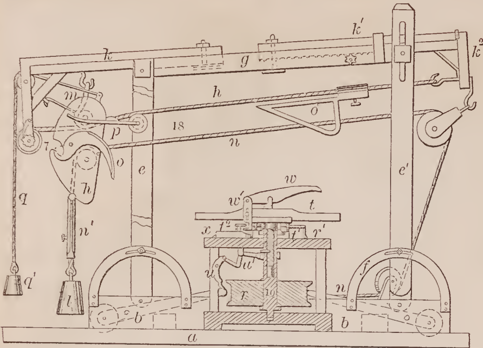
69257—E. U. & W. L. Scoville—Hoisting Apparatus.
