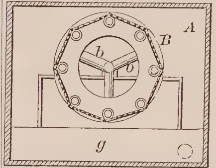
72254—J. E. Winants—For Melting Crude Turpentine.
