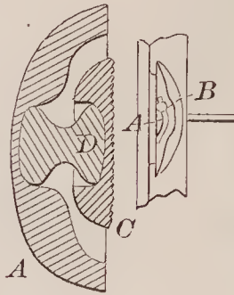
67606— S. E. Strickland— Sash Fastener.
