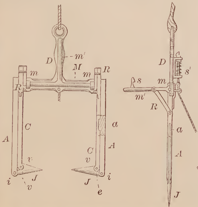
72837—J. Gilmore—Horse Hay Fork.
