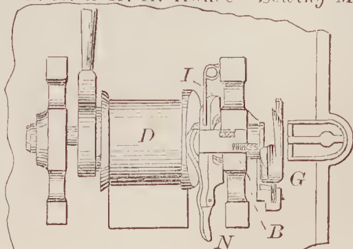
67652—J. A. & H. A. House—Sewing Machine.
