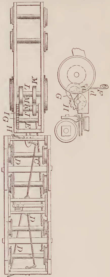
69892—J. L. Barnes— Car Brake.
