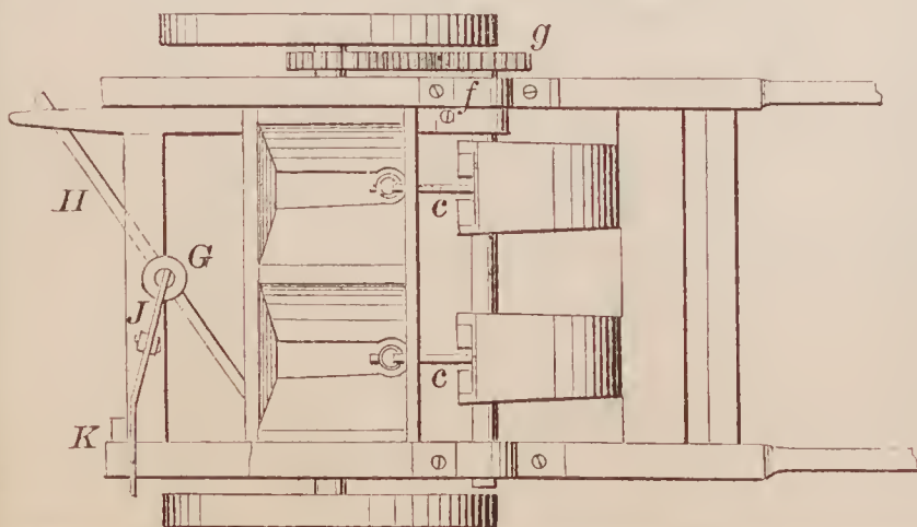
70786—Bendix & Dietsch—Potato Planter
