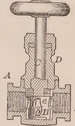
72529—G. Murray— Valve.
