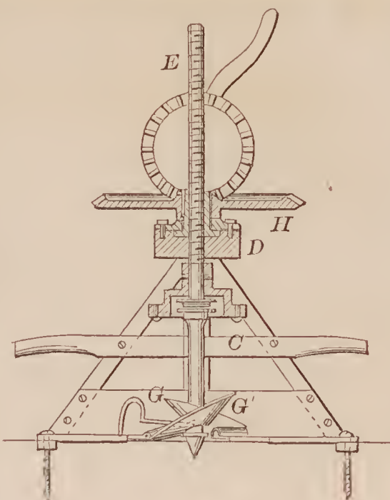
72497—W. R. Des—For Boring Post Holes
