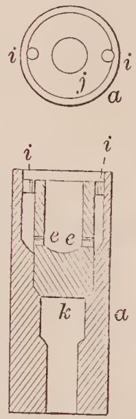
72531—G. H. Noble— Spindle Step.
