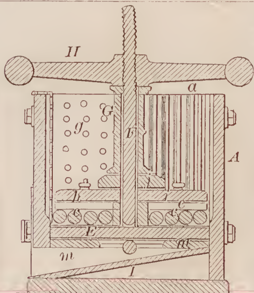
70468—A. L. Rand—Wine Press.
