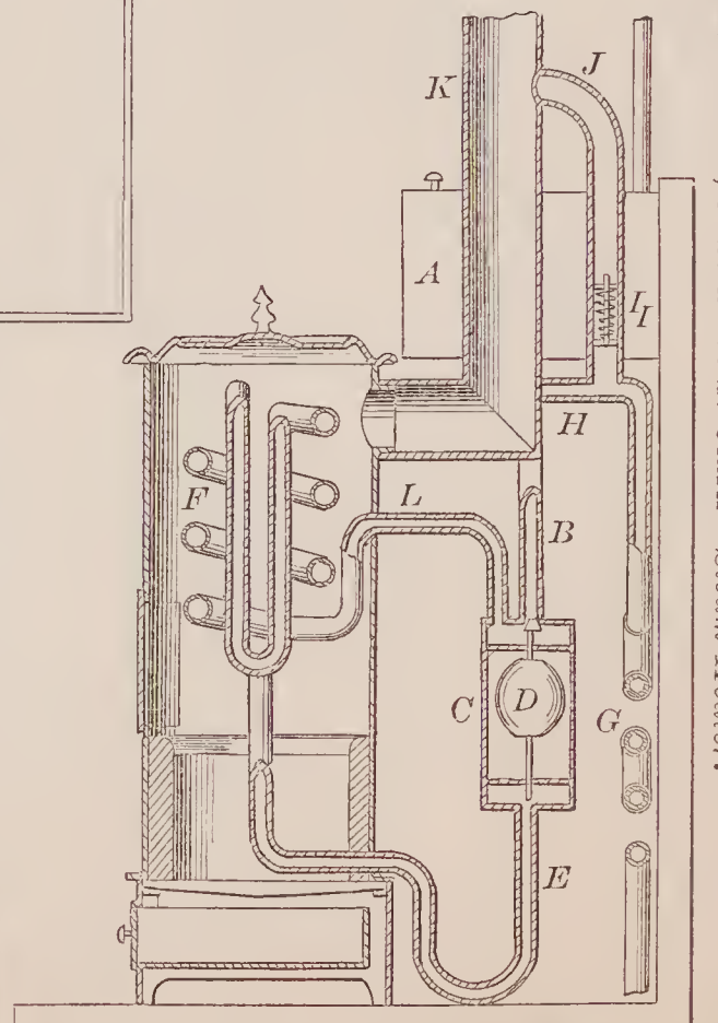
69542—E. B., J. S. & W. S. Clark—Steam Heater.
