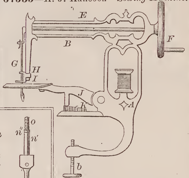
67535—H. J. Hancock—Sewing Machine.
