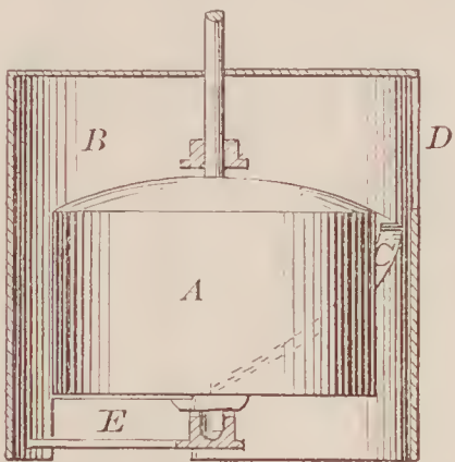
69459—H. McElDowney—For Ventilating Millstones.
