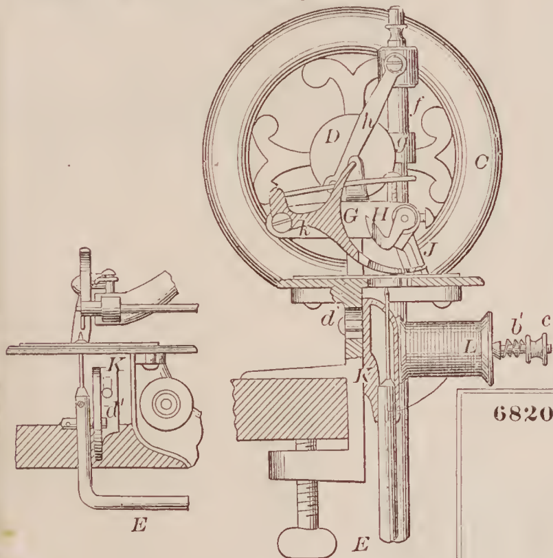
68196—W. S. Hill—Sewing Machine.
