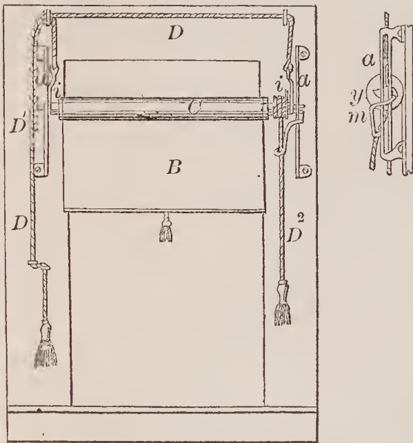
67337—D. G. Morgan—Window Curtain.
