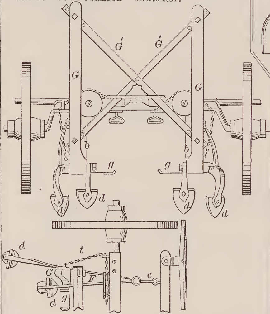
71623—J. P. Johnson— Cultivator.
