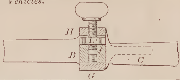
69403—J. G. Buzzell—Carriage Wheel.
