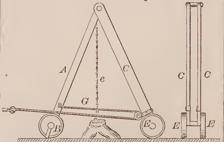
68228—I. H. Palmer—Stump Extractor.
