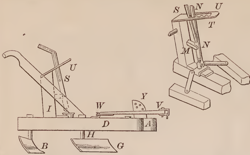
68392—J. P. Stanton— Potato Plow.
