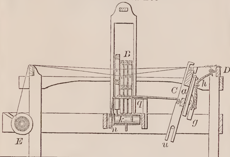
71087—T. H. Tibbles—Hand Loo
