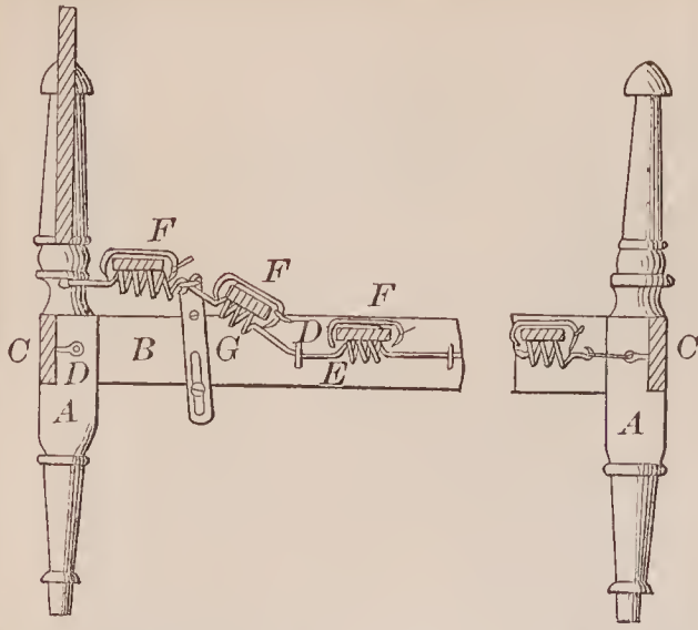
68499—J. S. Grant— Bed Bottom.
