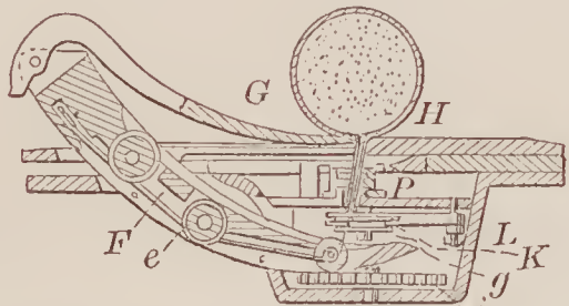
67393—A. M. Wright— Bag Fastener.
