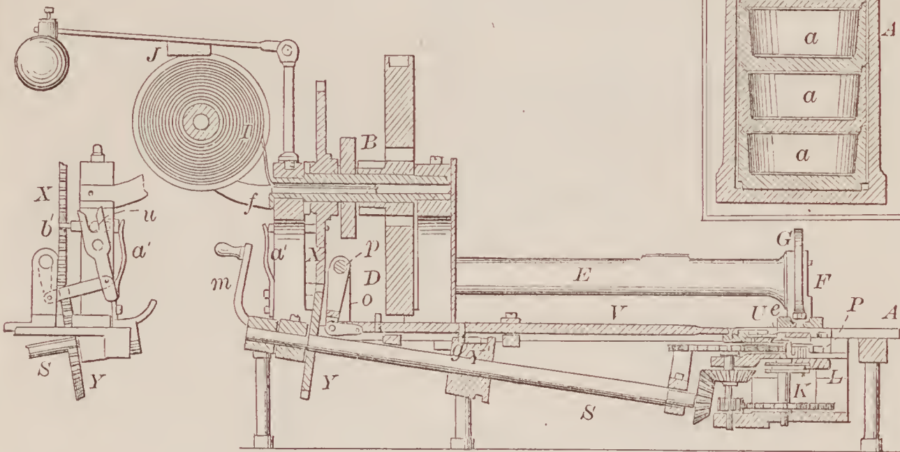
67389—G. Warner— Grain Binder.
