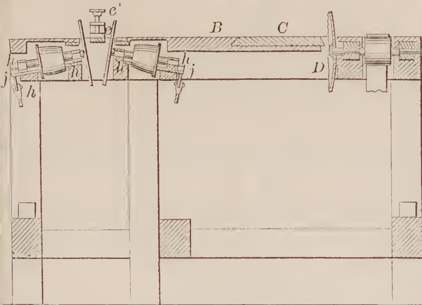
71276—F. O. Clark—Stave Machine.
