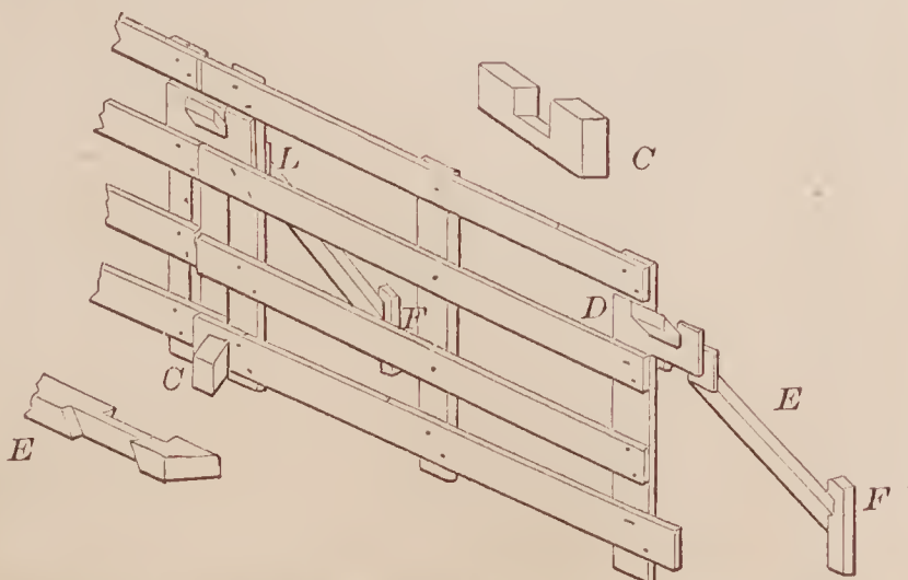
68116—A. M. Nichol—Fence.
