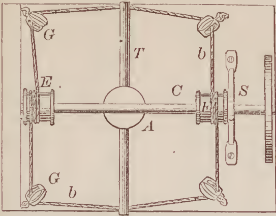
69564—F. G. Hesse— Amalgamator.
