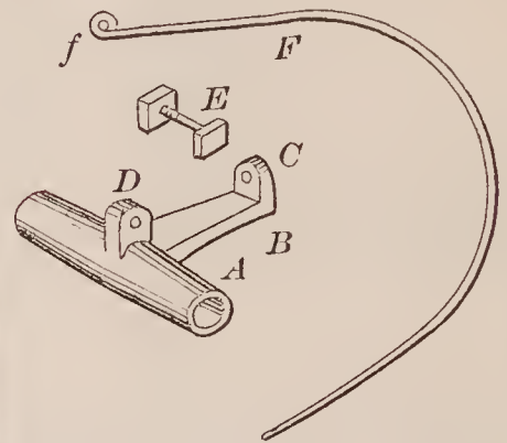
70643—H. K. Stoner—Horse Rake.
