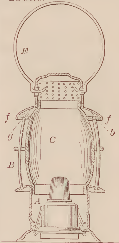
66902—C. F. Spencer— Lantern.
