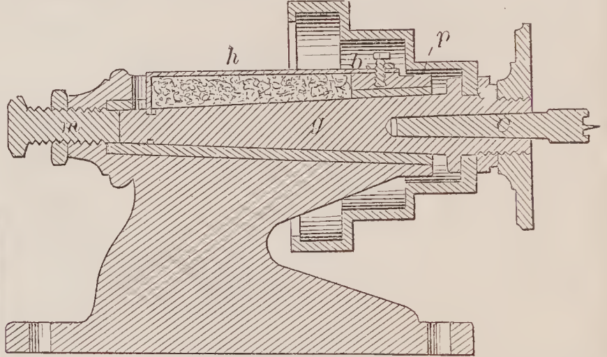
67676—J. Richards—Turning Lathe.
