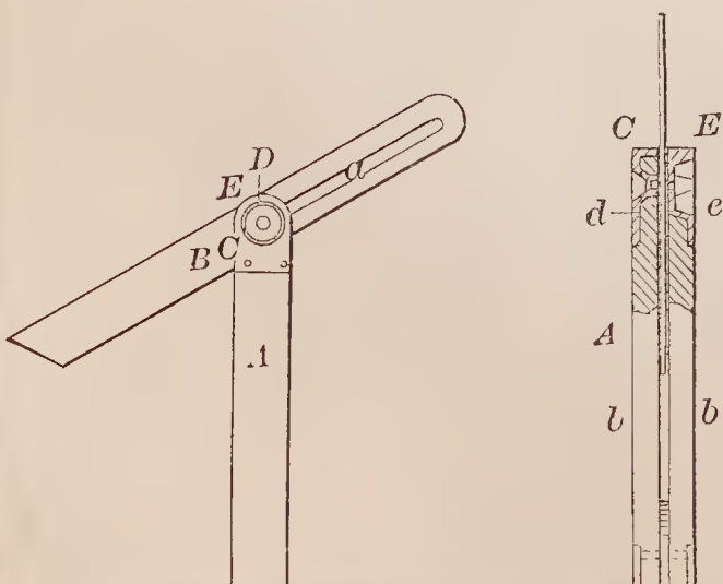
70570—L. D. Howard—Bevel.
