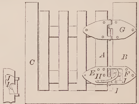
70762—G. L. Templeton— Gate.
