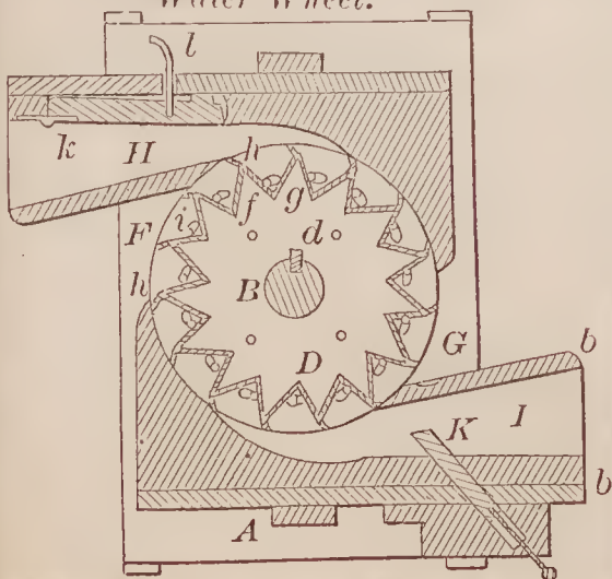
69169—L. W. & R. A. Blood— Water Wheel.
