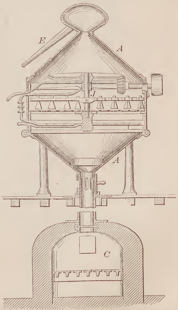
69534—W. Blakey— Malt Kiln.
