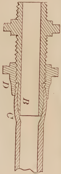
68348—J. R. Buchanan—Hose Coupling
