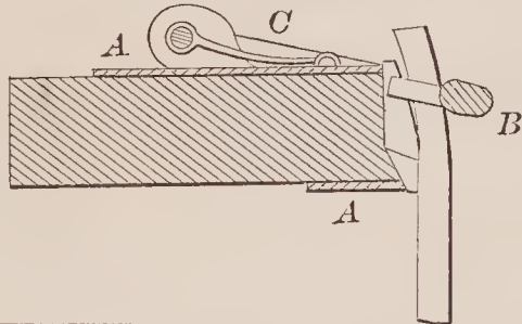
71295—E. H. & E. B. Goelet— Seeding Machine.
