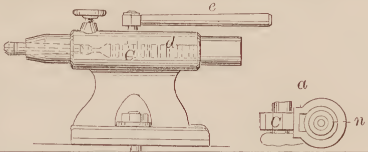
66889—O. L. Robinson—Cherry Stoner.
