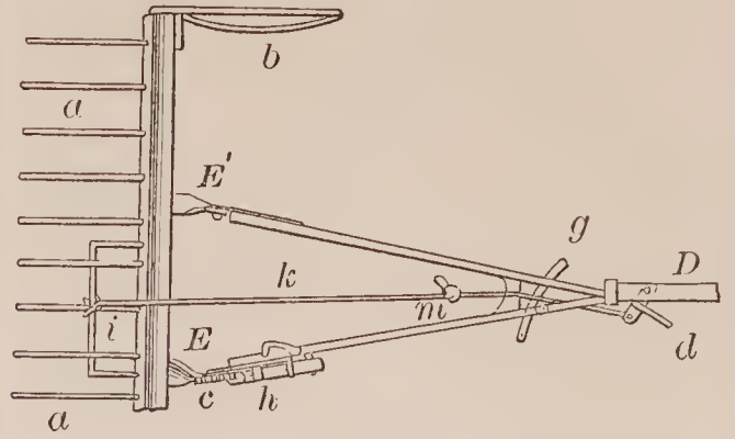
68500—J. S. Grant— Horse Rake.
