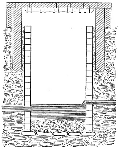
Fig. 140. Silt basin.
