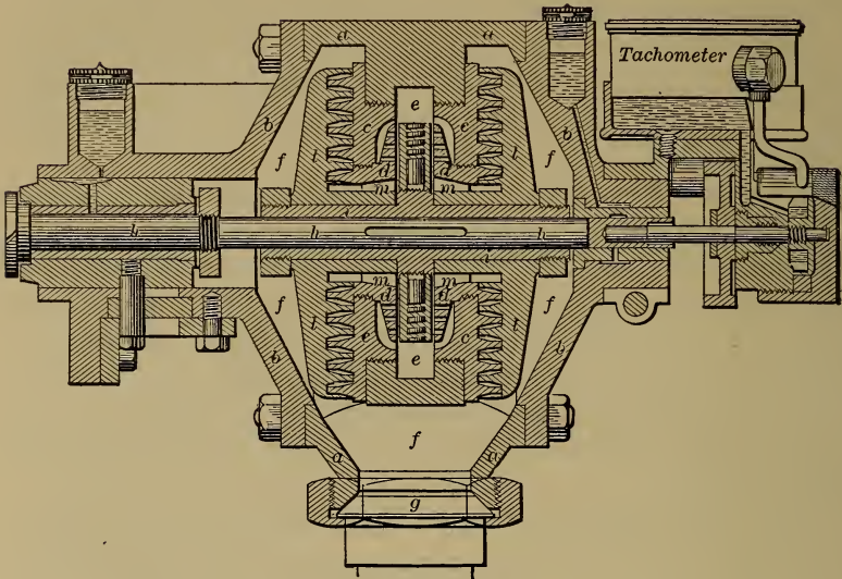
FIG. 43.—DOW TURBINE.
