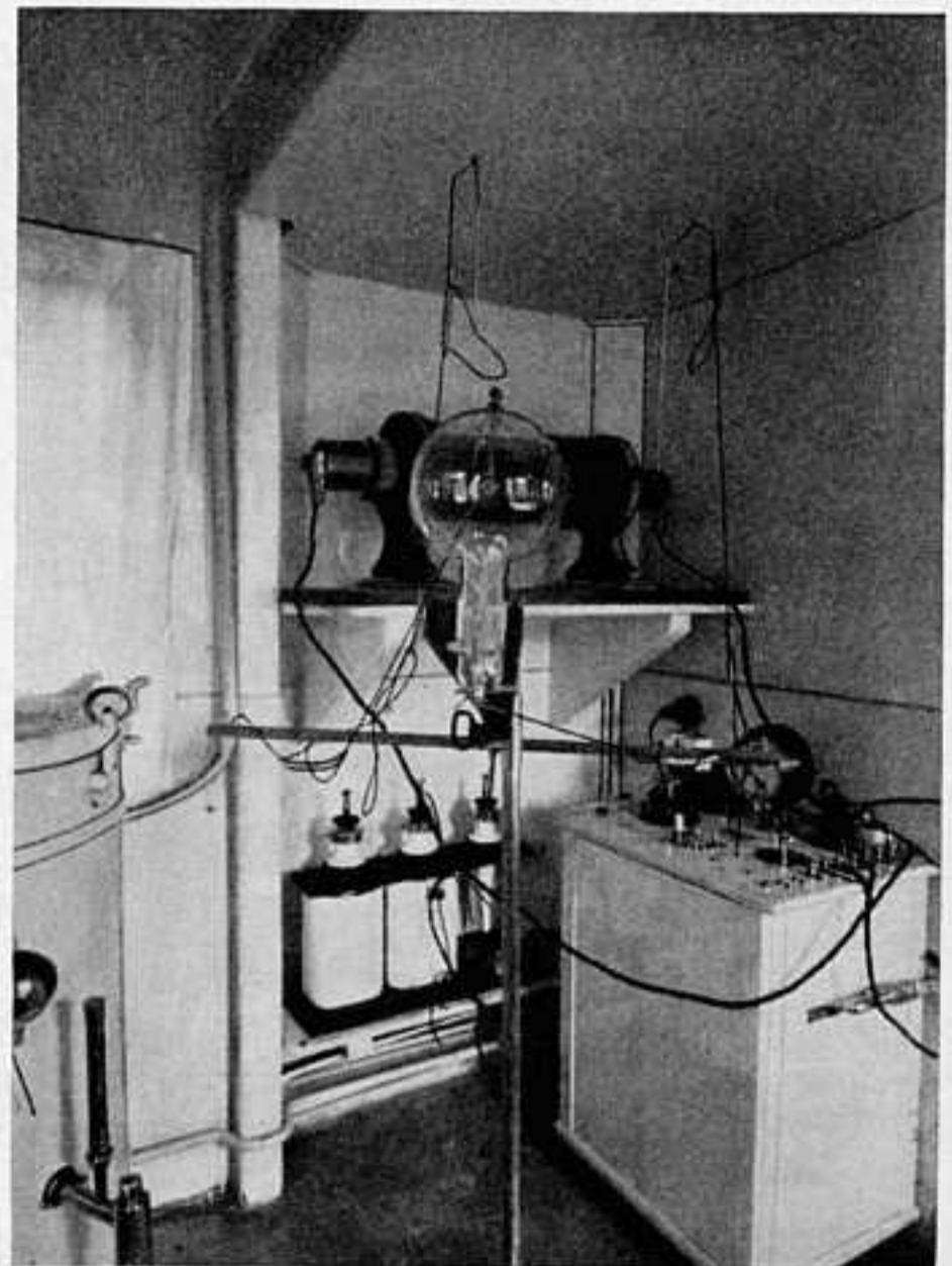
ОПЕРАЦІОННОЕ ОТДѢЛЕНІЕ ВЪ ВАГОНѢ САНИТАРНАГО ПОѢЗДА. АППАРАТЪ РЕНТГЕНА.
