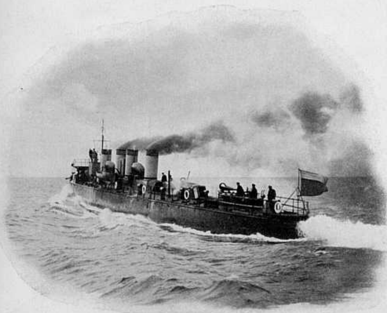
МИНОНОСЕЦЪ «БРАВЫЙ». ФОТ. Н. Н. АПОСТОЛИ. ВСЯКІЯ КОПИ ВОСПРЕЩАЮТСЯ.
