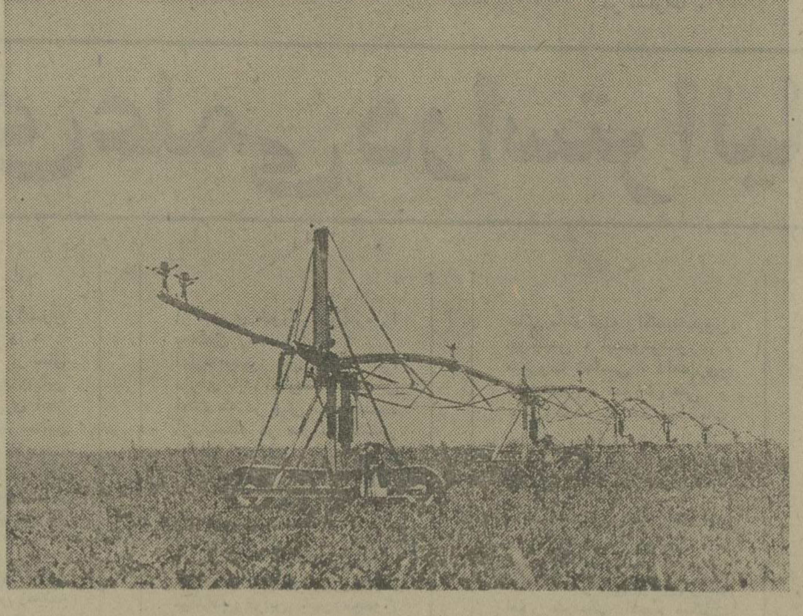
دستگاه آبیاری اتوماتیک‌سیار بهترین نتیجه را در کشاورزی با حداکثر صرفه‌جویی تضمین میکند.
