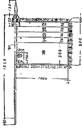
(別圖第一) 騎兵團軍旗 尺寸以公釐爲標準
