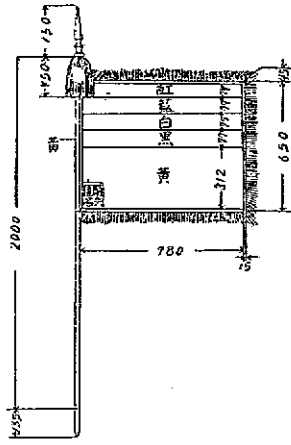
(別圖第一) 騎兵團軍旗 尺寸以公釐爲標準
