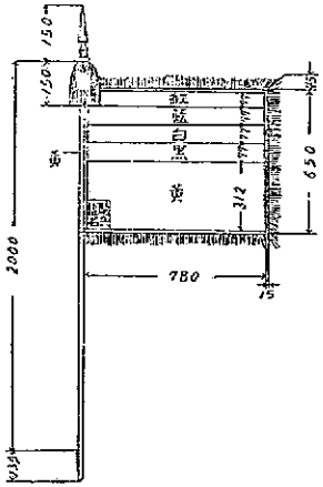
(別圖第一) 騎兵團軍旗 寸法耗
