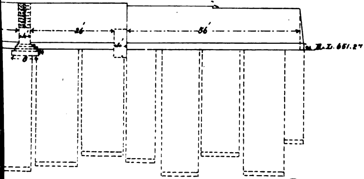
Elevation
