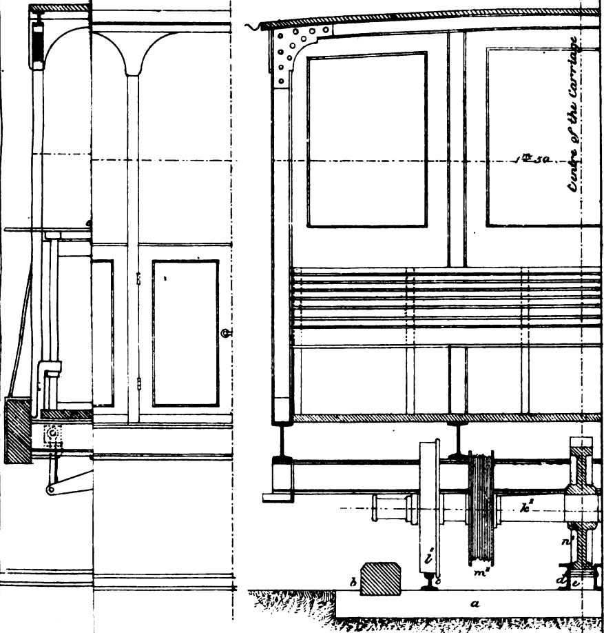
Fig. 19. Transverse Section
