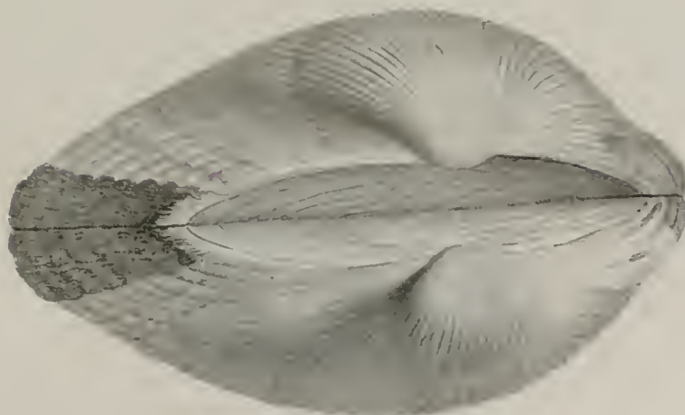
L. 23. americana Noh
