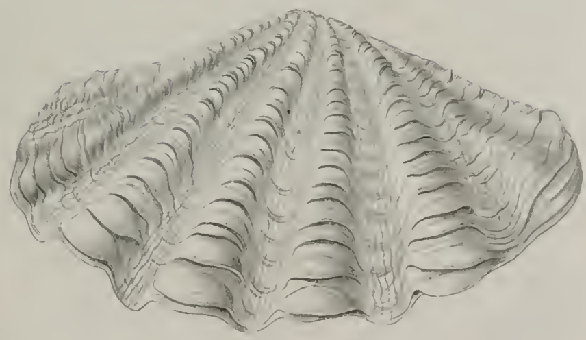
Fig. 1. Cardium Formasimanum Nob Fig. 2. Trochana longatissima . Nob
