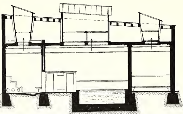
197. Folkskolebad på Östermalm, genomskärning.
