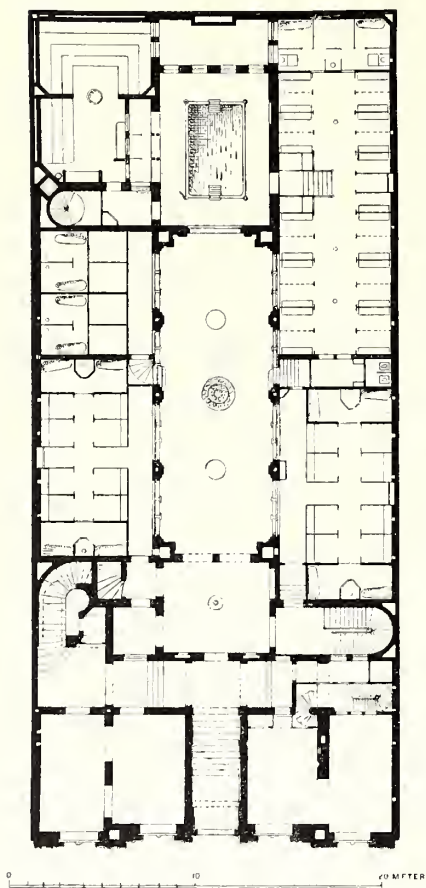
194. Sturebadet, plan af bottenvåningen.
