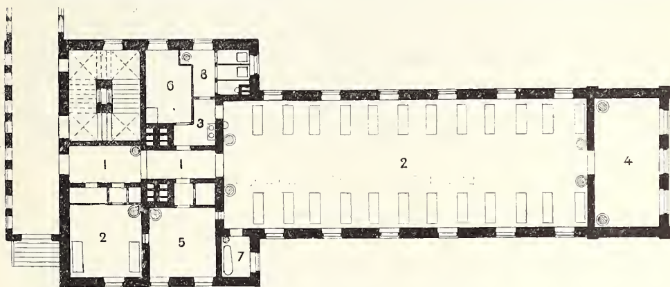
211. Sabbatsbergs sjukhus, sjukpaviljong.
