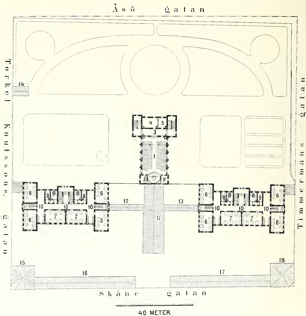
249. Plan af södra fattighuset, våningen 1 tr. upp.
