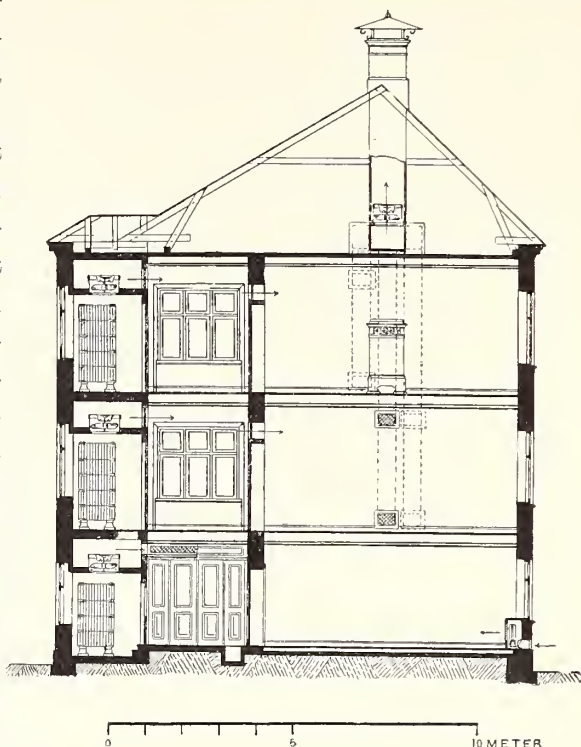
222. Maria sjukhus, uppvärmning och ventilation.
