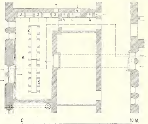
220. Sjukhuset Sankt Göran, ventilation och uppvärmning.
