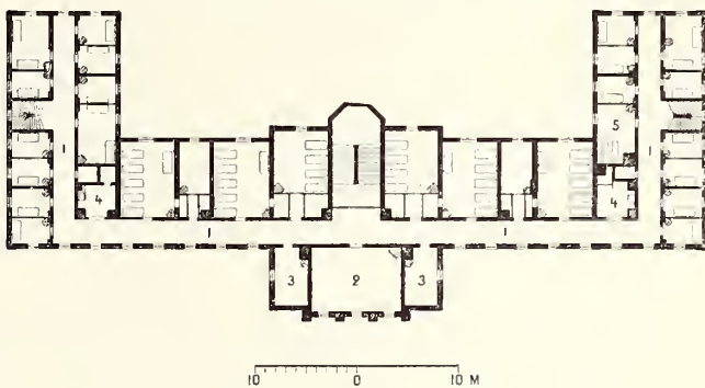
237. Stockholms sjukhem, plan af våningen 1 tr. upp.
