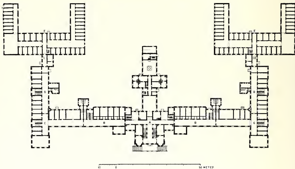
235. Stockholms hospital Konradsberg, plan af bottenvåningen.
