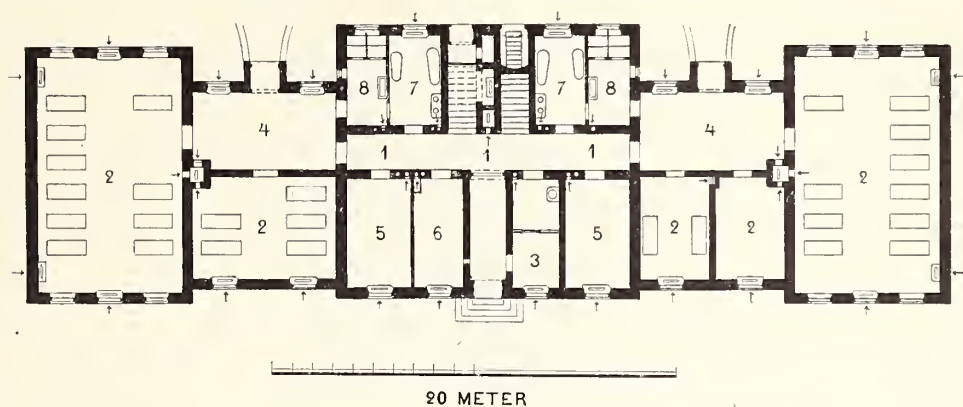
226. Epidemijukhuset, plan af sjukpaviljong.
