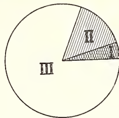
7. Rumförhållandet hos Mälarens 3 östra bäcken.
