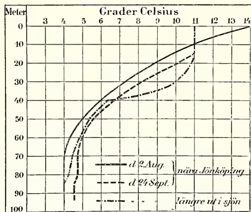
20. Temperaturkurvor för södra Vättern 1895.
