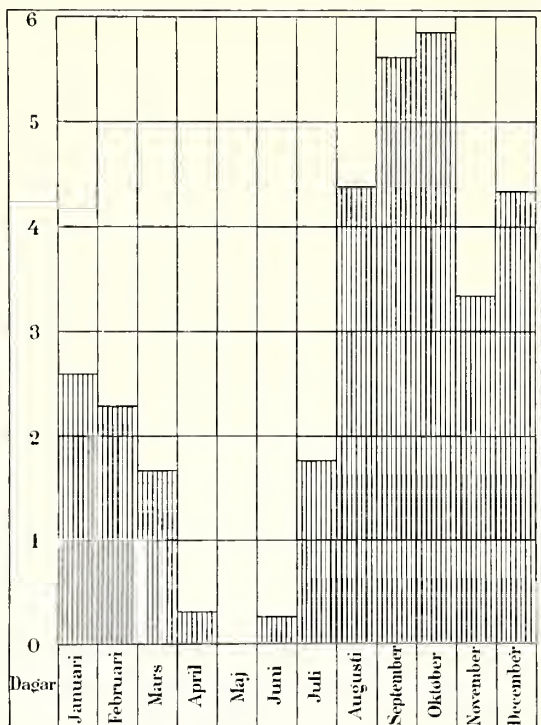
14. Medeltalet uppsjödagar per månad.
