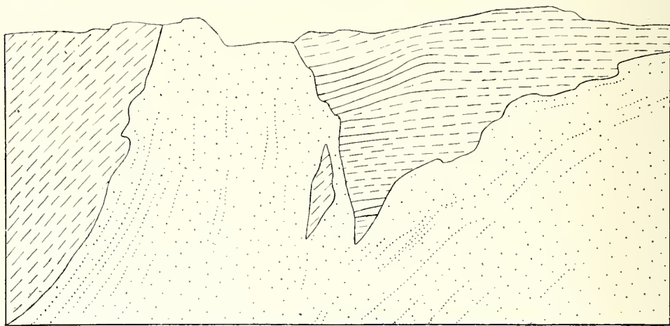
2. Granitgång i gneis vid Vegagatan, tecknad efter fotografi. Graniten är prickad, gneisen streckad, bergväggens höjd 4 m.
