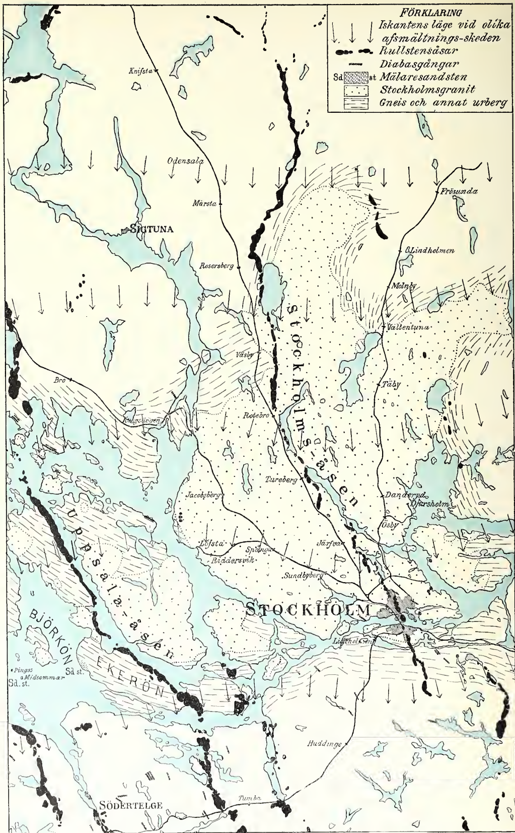
1. Karta öfver Stockholmstraktens berggrund och rullstensåsar.
