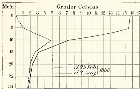
21. Temperaturkurvor vid Beckholmen 1888.
