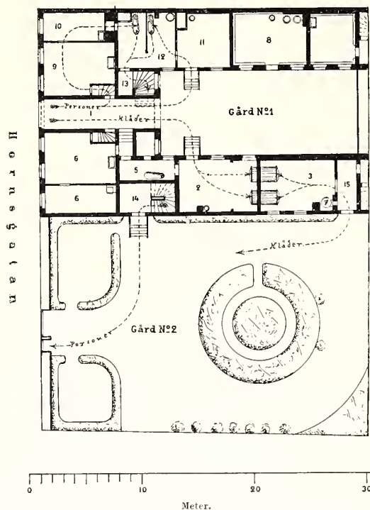
187. Plan af stadens desinfektionsanstalt.
