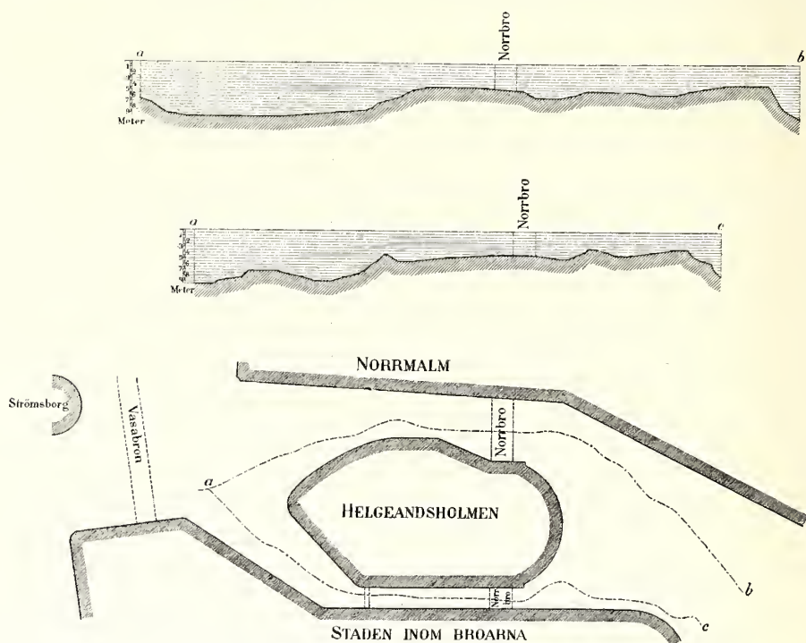
8. Profiler af Norrströms båda grenar, i djupaste rännan.
