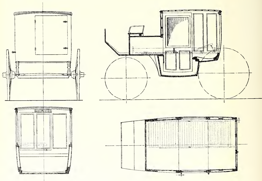
189. Sjuktransportvagn med rörlig sjukbår.
