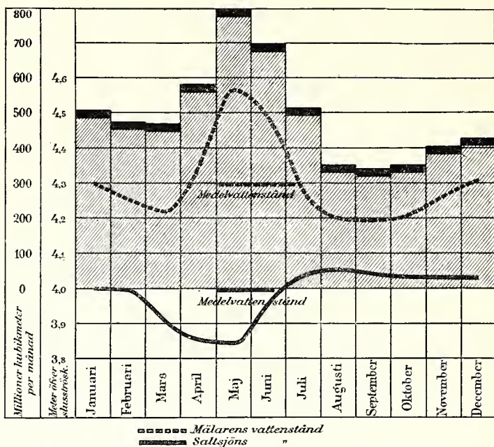
11. Månadsmedia för Mälarens och Saltsjöns vattenstånd samt medelkvantiteten uttrinnande vatten per månad.
