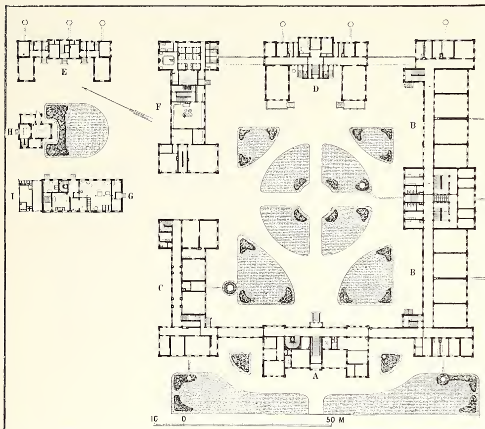
239. Plan af Stora barnhuset.
