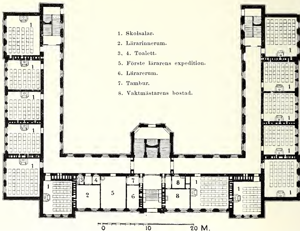
127. Plan af bottenvåningen i Maria folkskola, Ringvägen.
