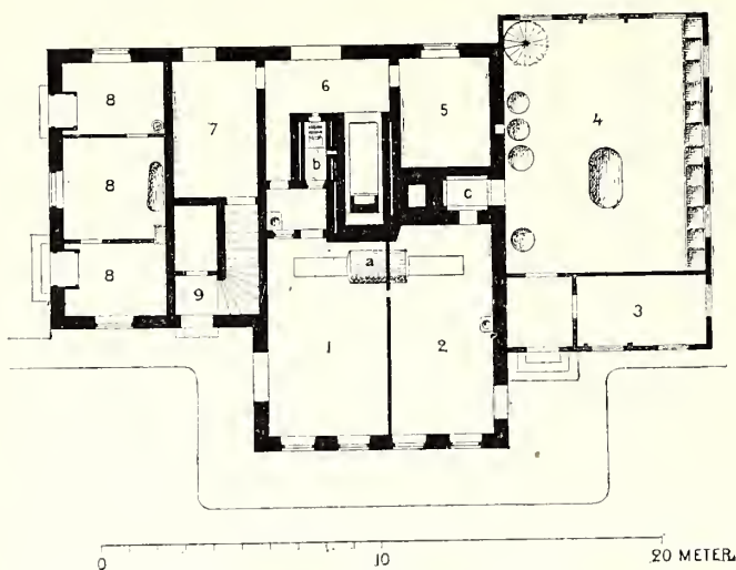
231. Epidemisjukhuset, desinfektions- och tvätthuset.
