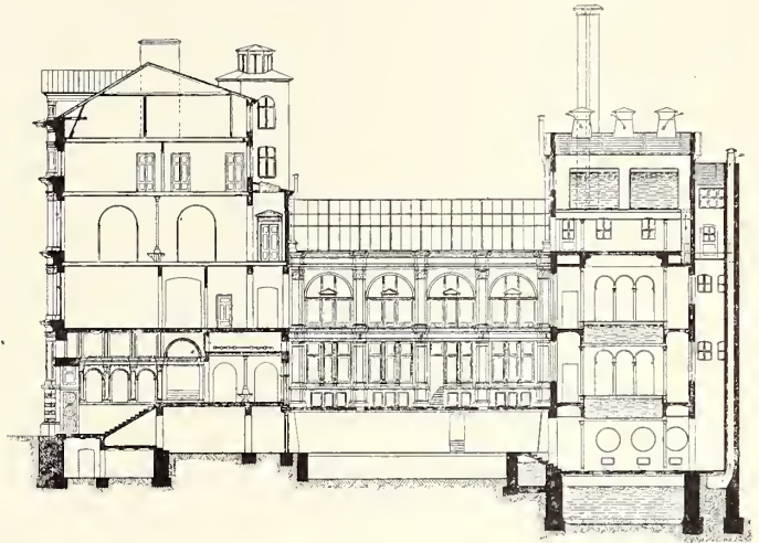
193. Sturebadet, längdgenomsnitt af byggnaden.
