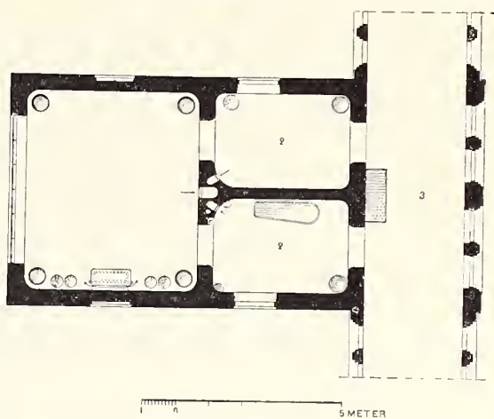
214. Sabbatsbergs sjukhus, plan af operationshuset.
