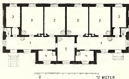
217. Sabbatsbergs sjukhus, isoleringspaviljong.
