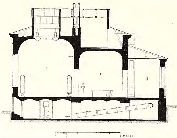
215. Sabbatsbergs sjukhus, genomskäring af operationshuset.
