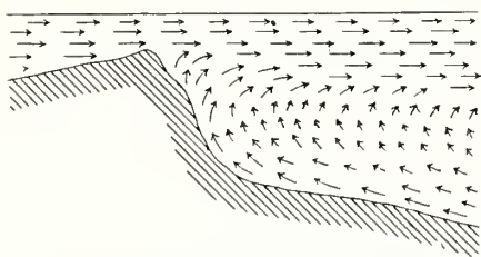
15. Förloppet vid tvänne vattenlagers reaktionsverkan på hvarandra.
