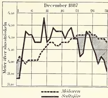
12. Mälarens och Saltsjöns vattenstånd hvarje dag kl. 8 i dec. 1887.
