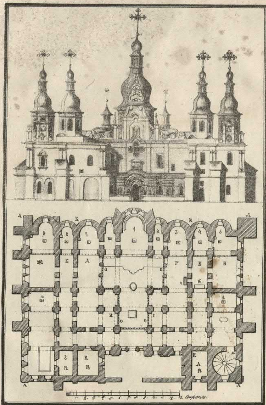
Планъ и Фасады Софійскаго Собора въ Кіевѣ.
