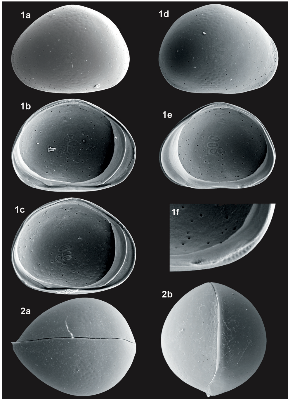
Cyclocypris laevis (O.F.MÜLLER, 1776) – Magdala (31) aHo 1a - LVa (L 0,47), 1b - LVi (L 0,49), 1c - LVi (L 0,49), 1d - RVa (L 0,48), 1e - RVi (L 0,48), 1f - RVi (Ausschnitt posteroventral L 0,17).
