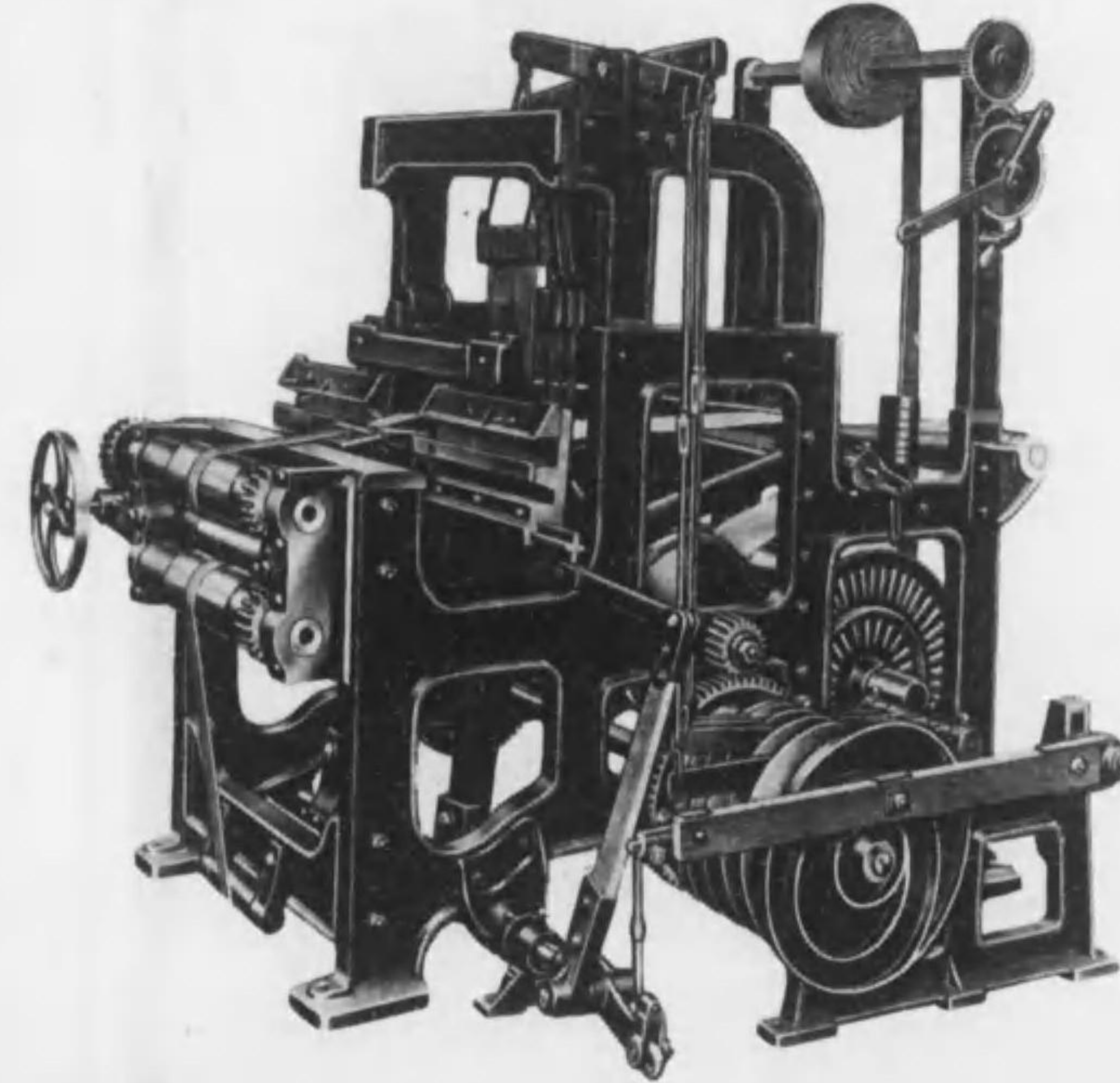
HP型ホースパイプ織機
