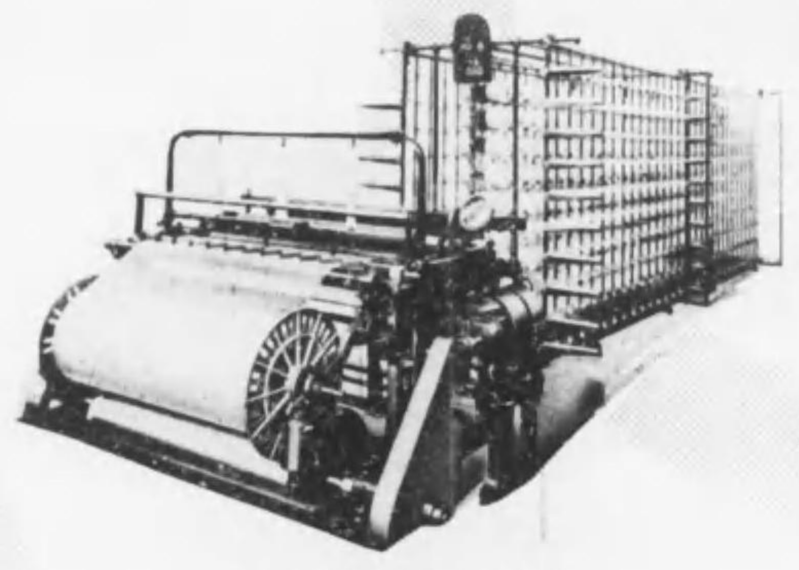
超高速度整經機
