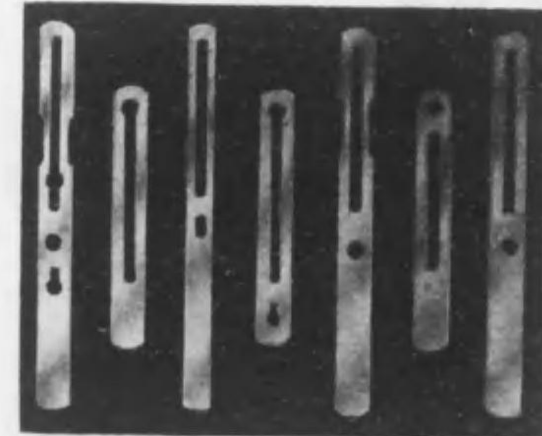
ドロツバー(經糸切斷停止裝置用)
