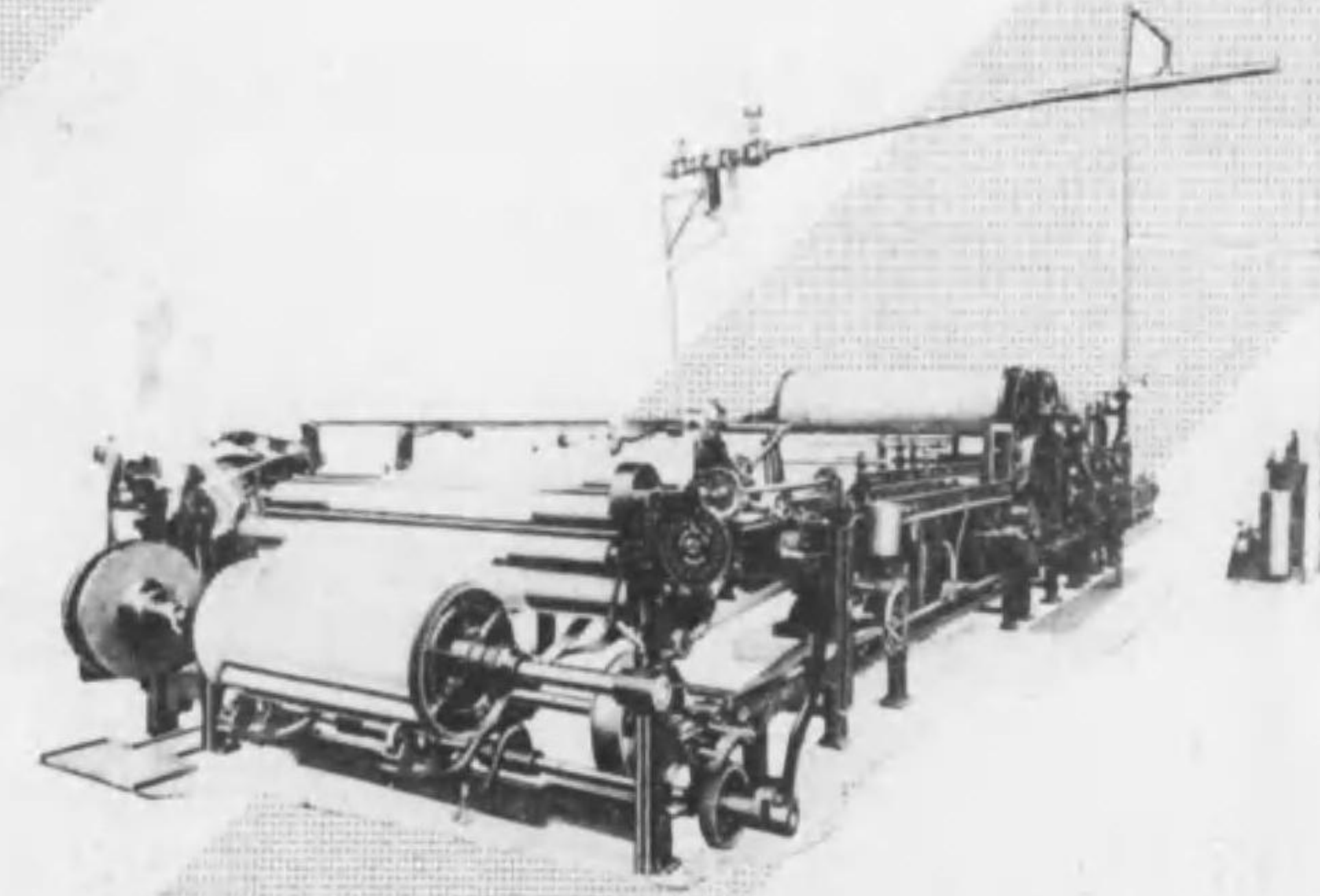
人絹・光棉糸糊附乾燥機
