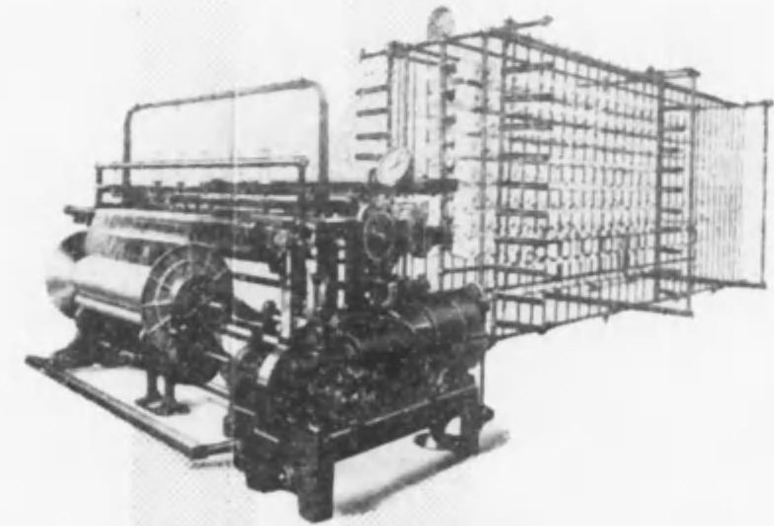
高速度人絹整經機
