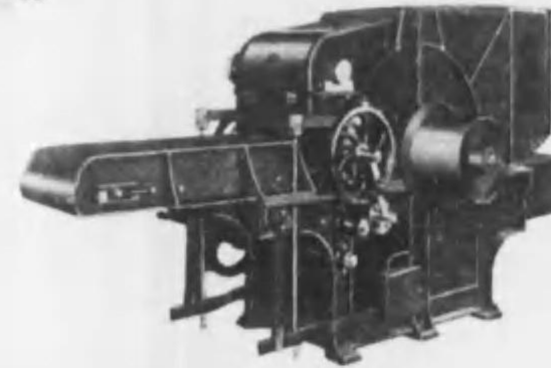
ラッグ マシン
