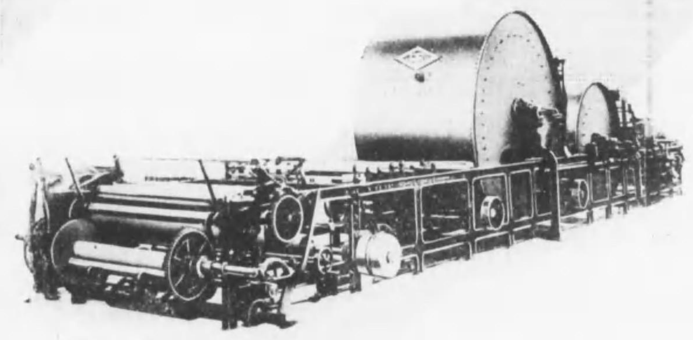
高能率スラッシャー經糸糊附乾燥機
