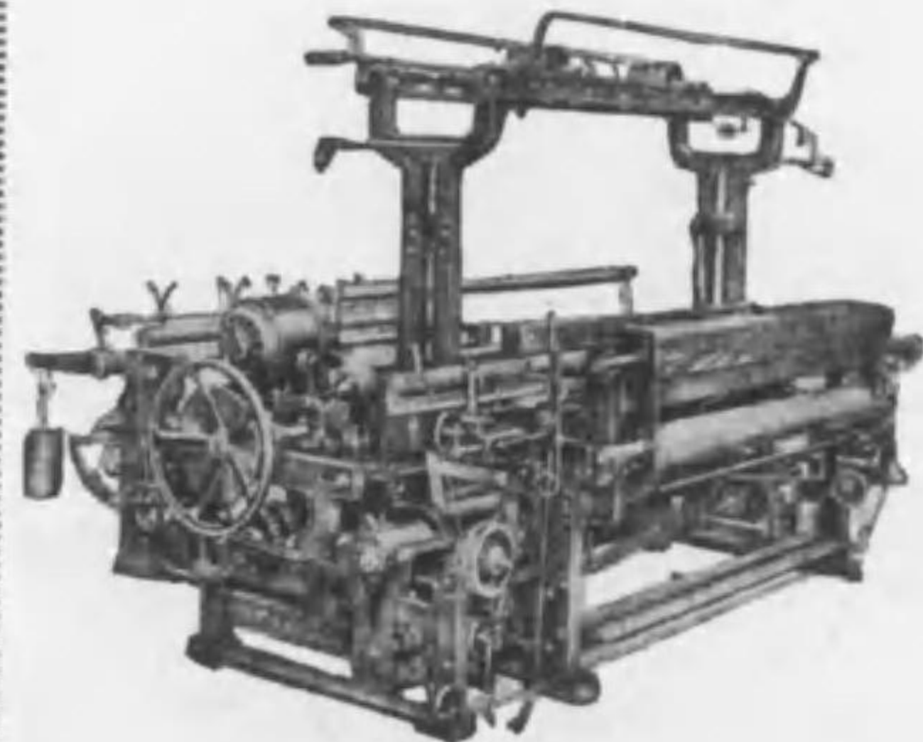
最新型二重天鷲絨織機
