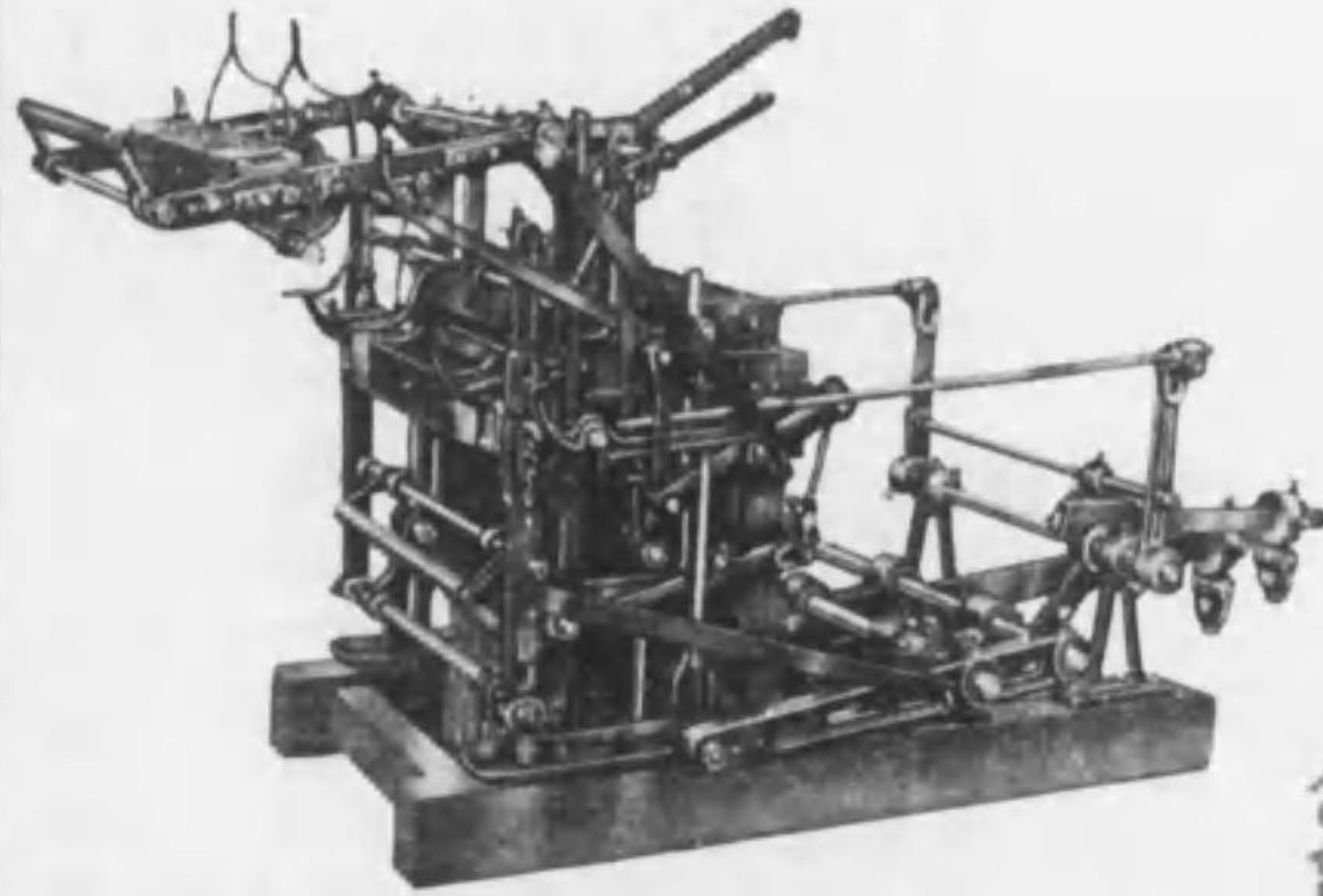
特許ダブルシリンダー ジャカード機
