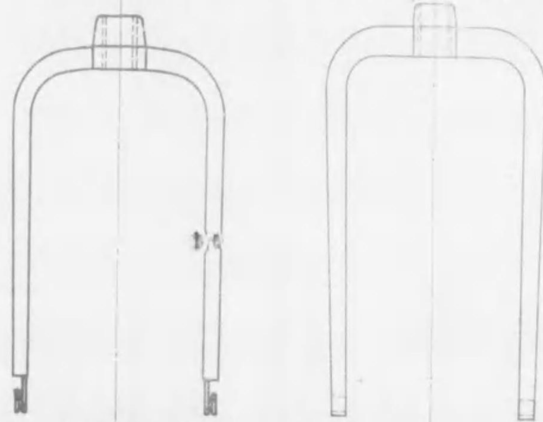
麻紡績用精紡機フライヤー 麻糸用フライヤー
