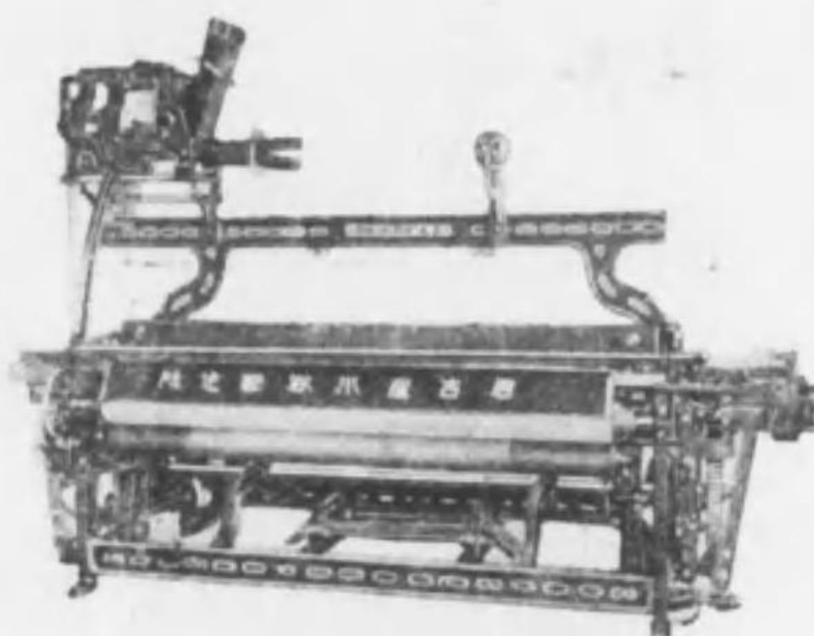
四中下ビー付織機
