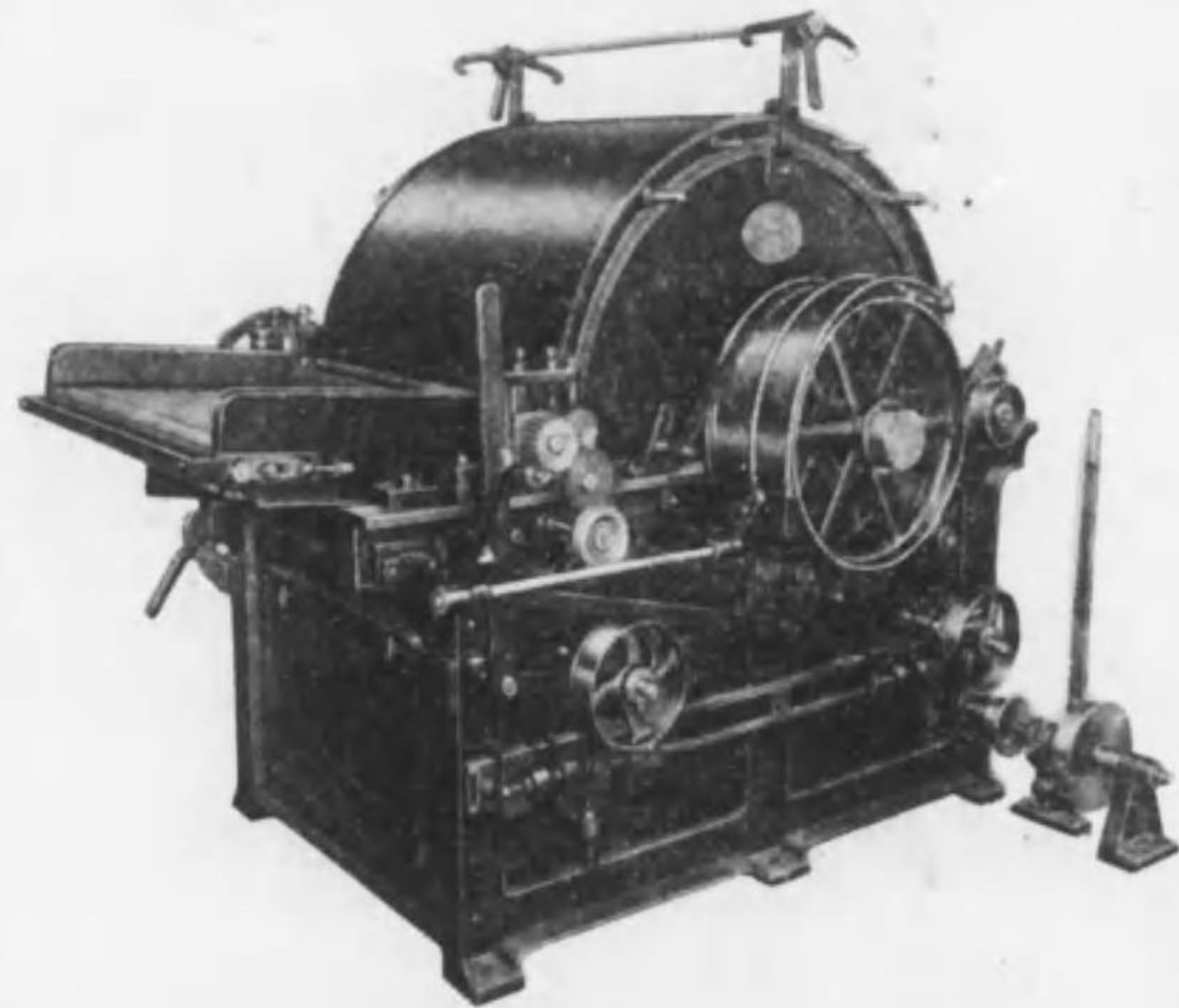
解 繭 機
