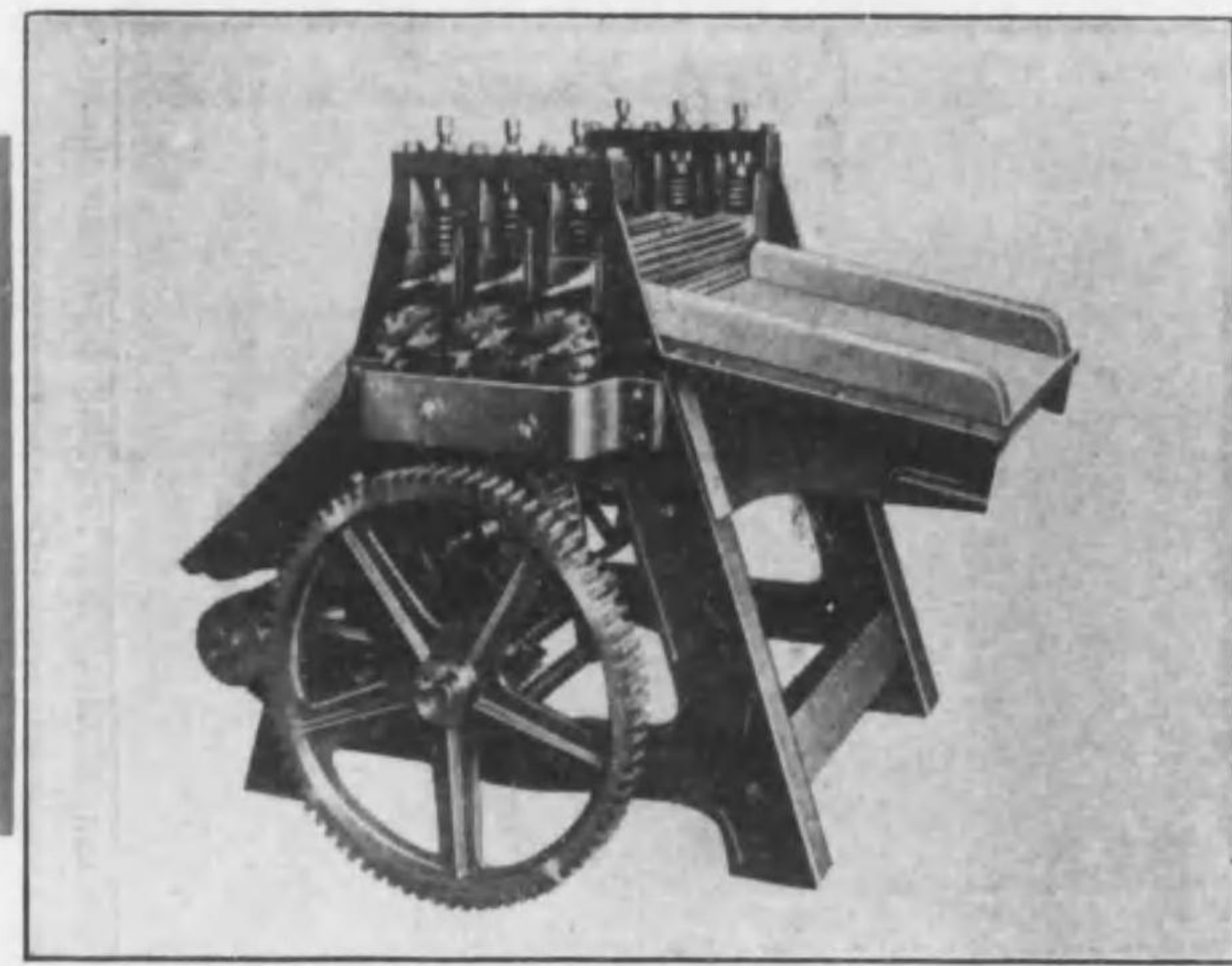
軟 織 機
