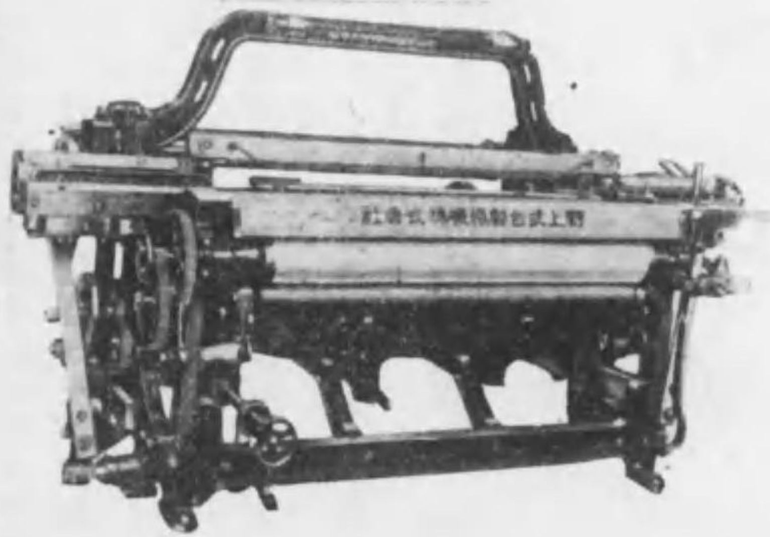
下打平織機
