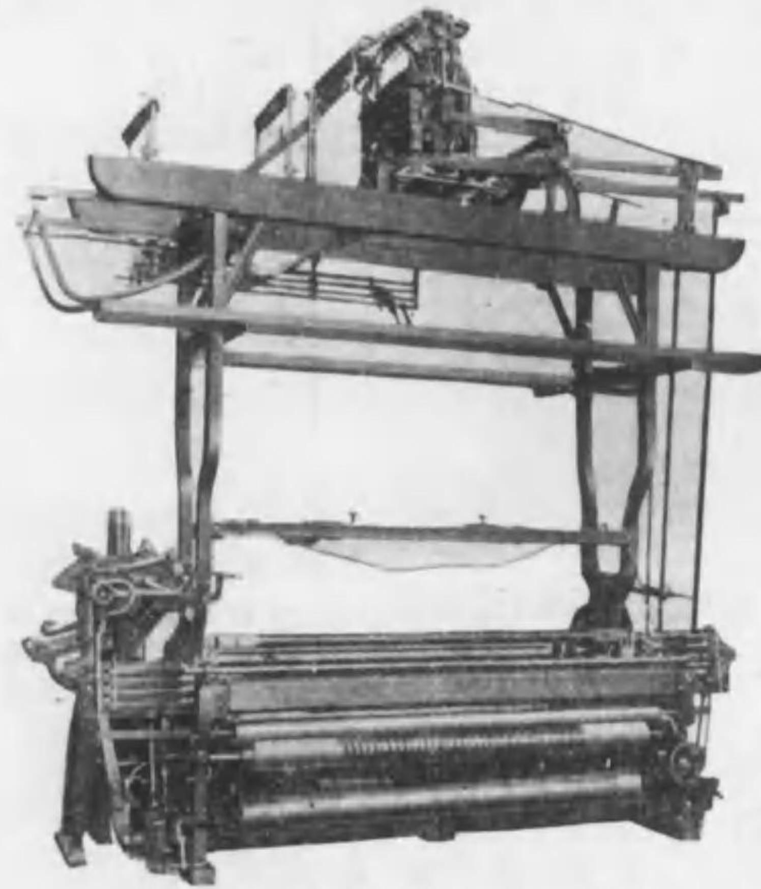
兩口式上下一方ダブルシリンダージャカード機
