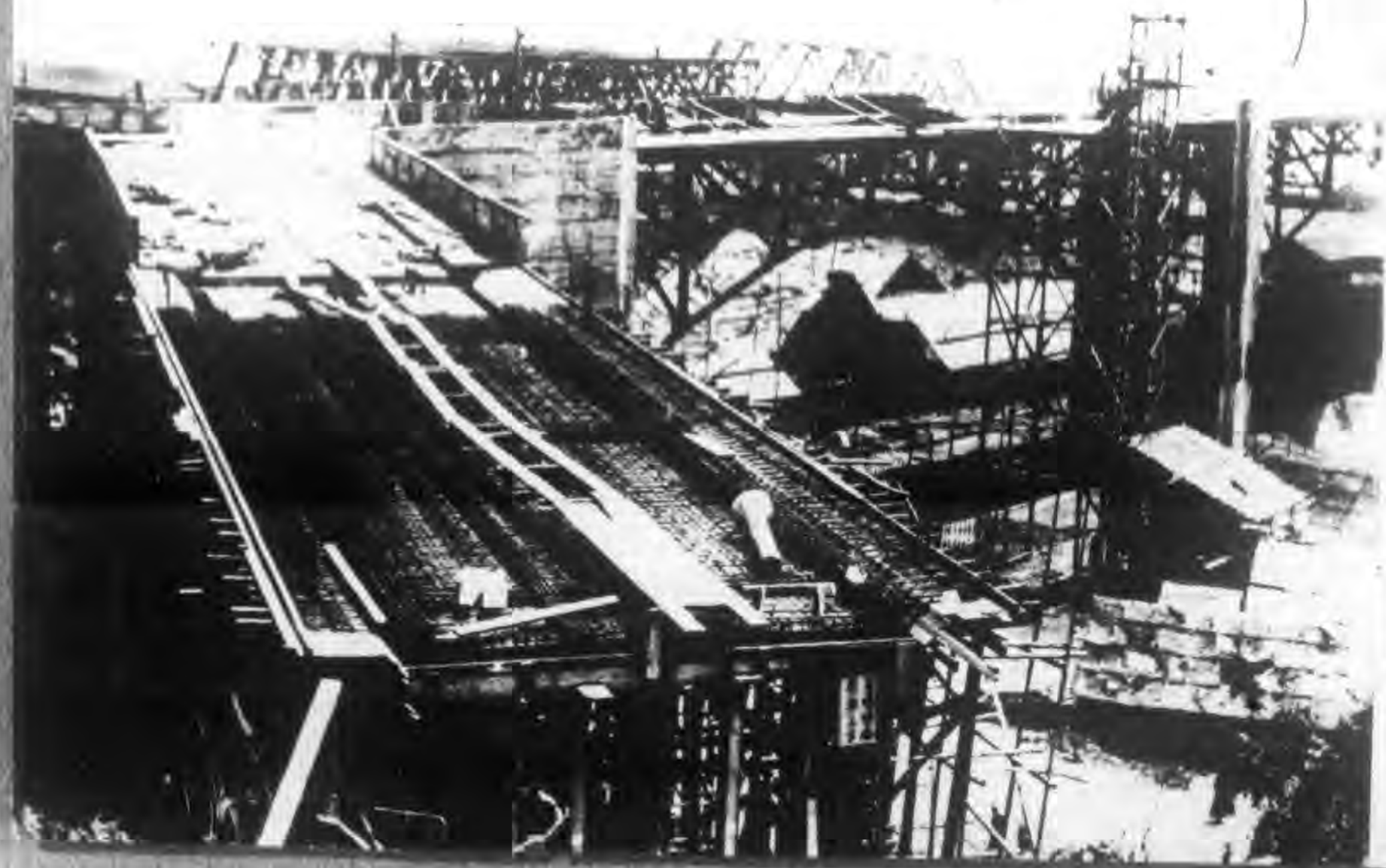
約一百呎。北岸的六墩，墩外設拱橋及混凝土橋梁，作公路引橋之用，下層鐵路則於橋墩起用墊土建築與兩岸之鐵路接軌，圖為該橋最近工程情形。 (吳寶基攝誌)
