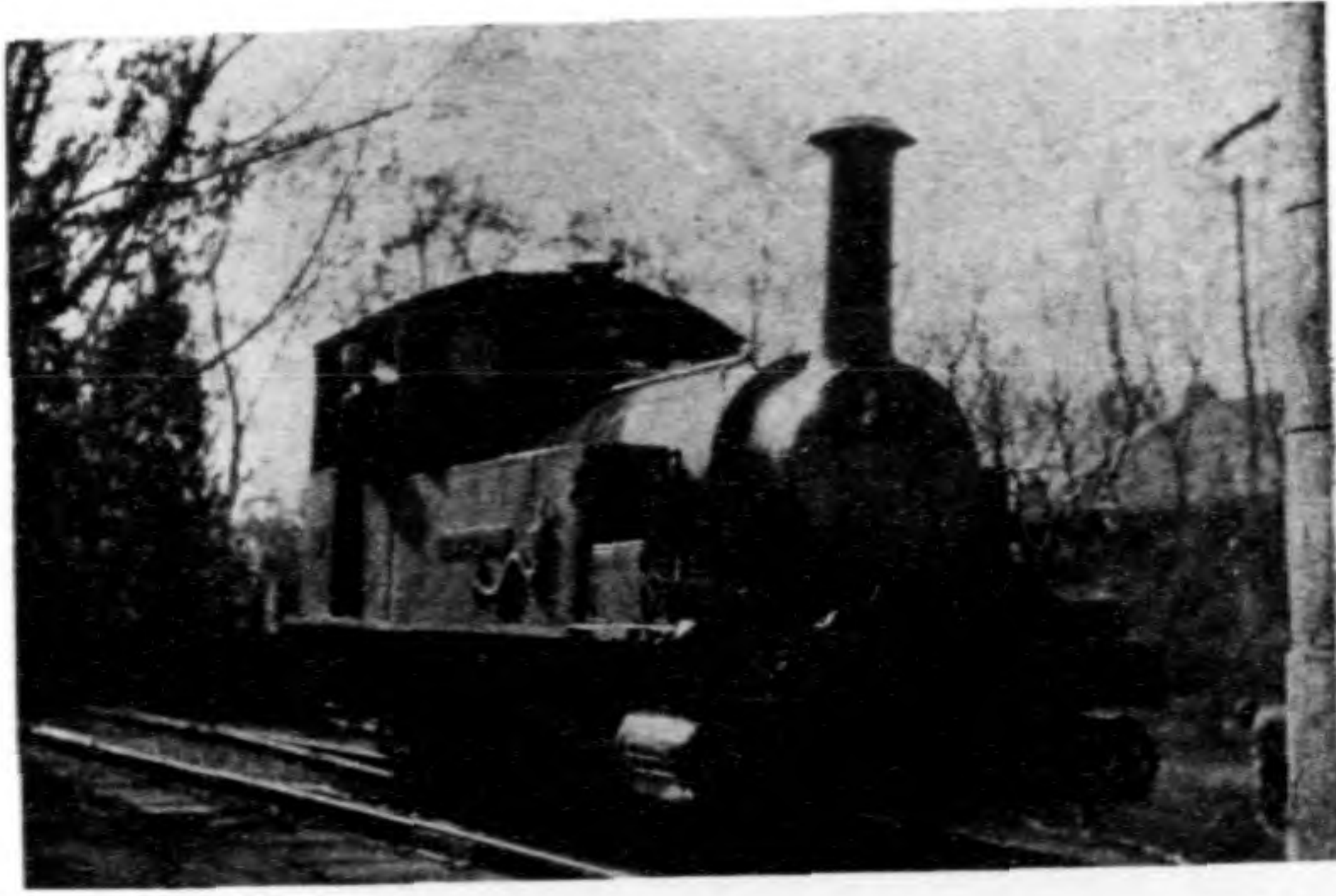
中國第一機車
