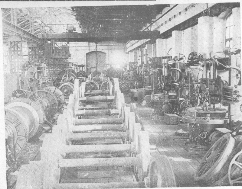
哈爾濱鐵路總 工廠車輪場
