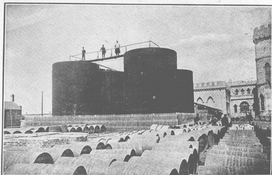
伯羅金高田酒廠 存放酒精油槽
