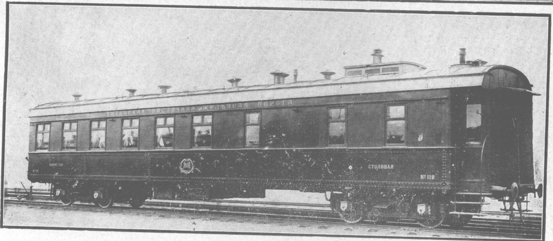
東省鐵路飯車
