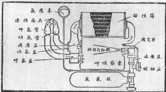
連有壓縮氧之面具
