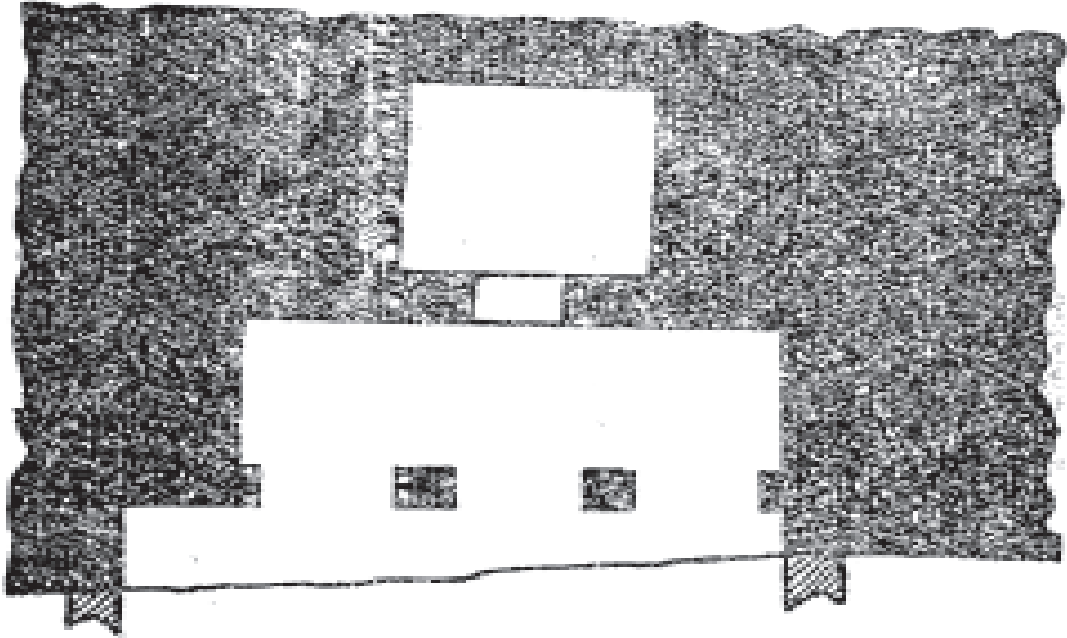
மேலைச்சேரி குகைக்கோயில் தரையமைப்பு
