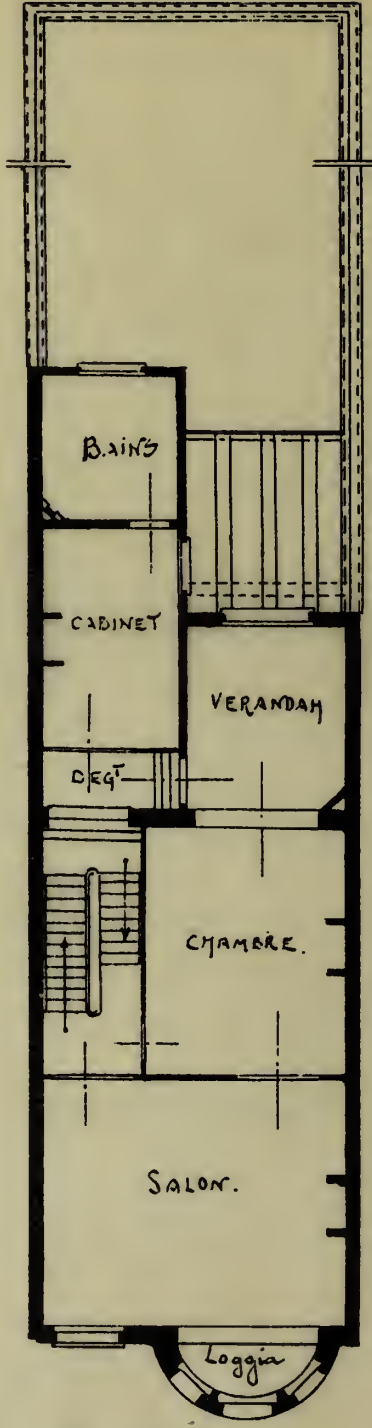
PREMIER ETAGE.
