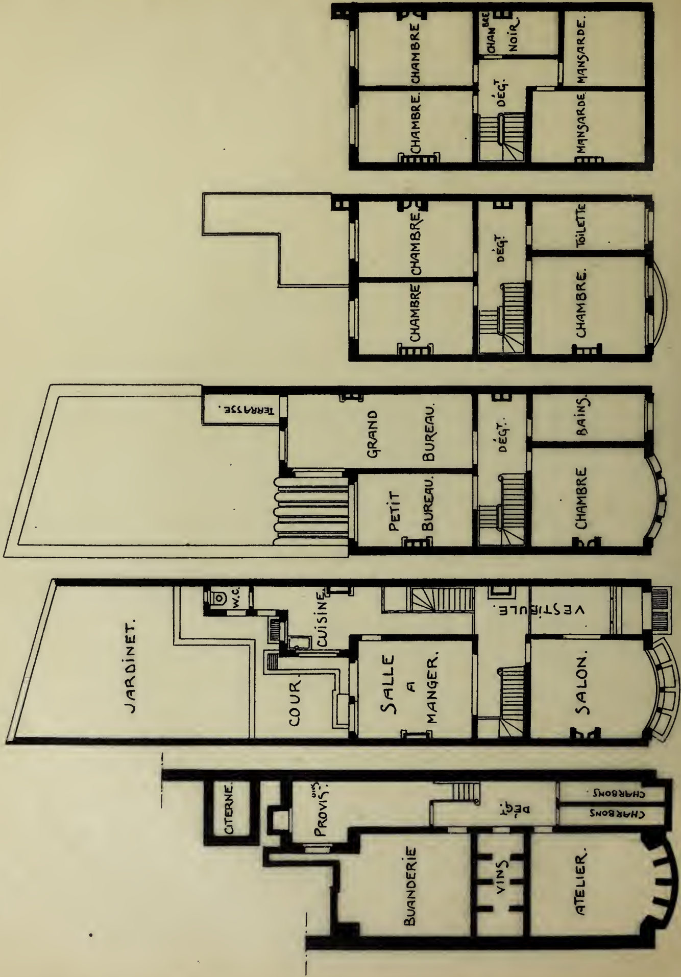
REZ DE CHÉE. PREMIER ETAGE. SECOND ETAGE. COMBLES.
