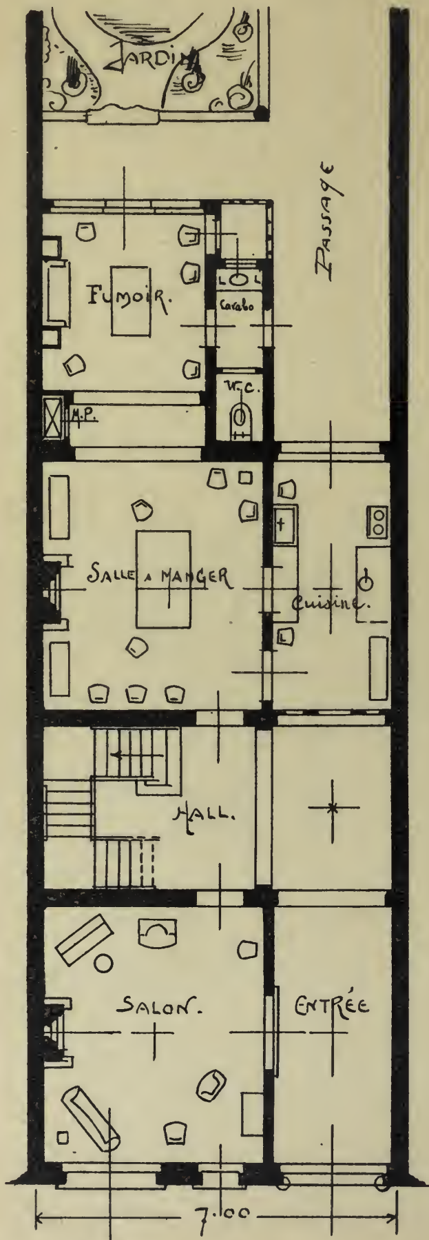
REZ-DE-CHAUSSÉE.
