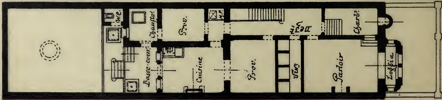
Souterrains
