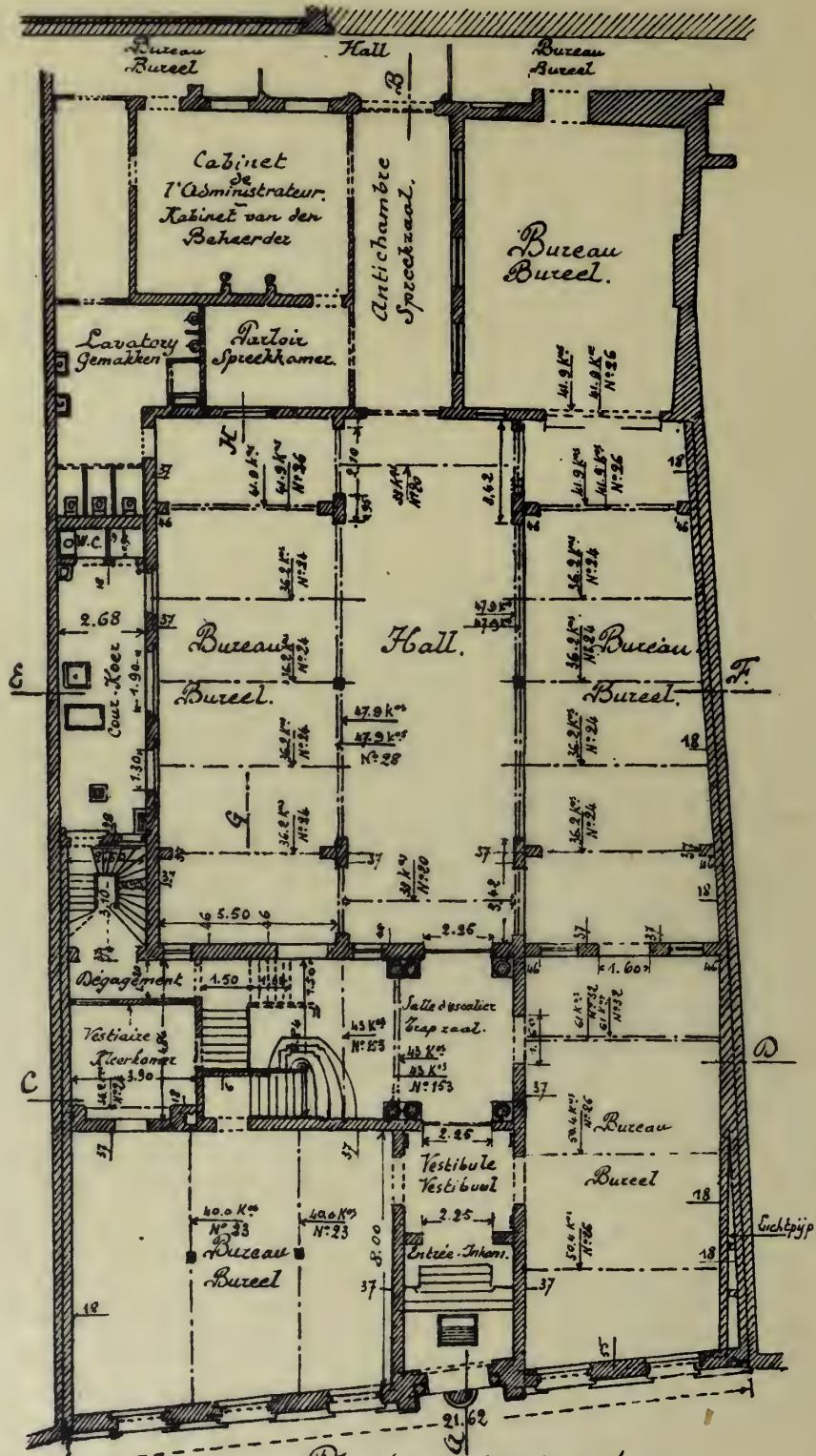
— Plan du rez-de-chaussée — — Plan van gelijkvloers. —
