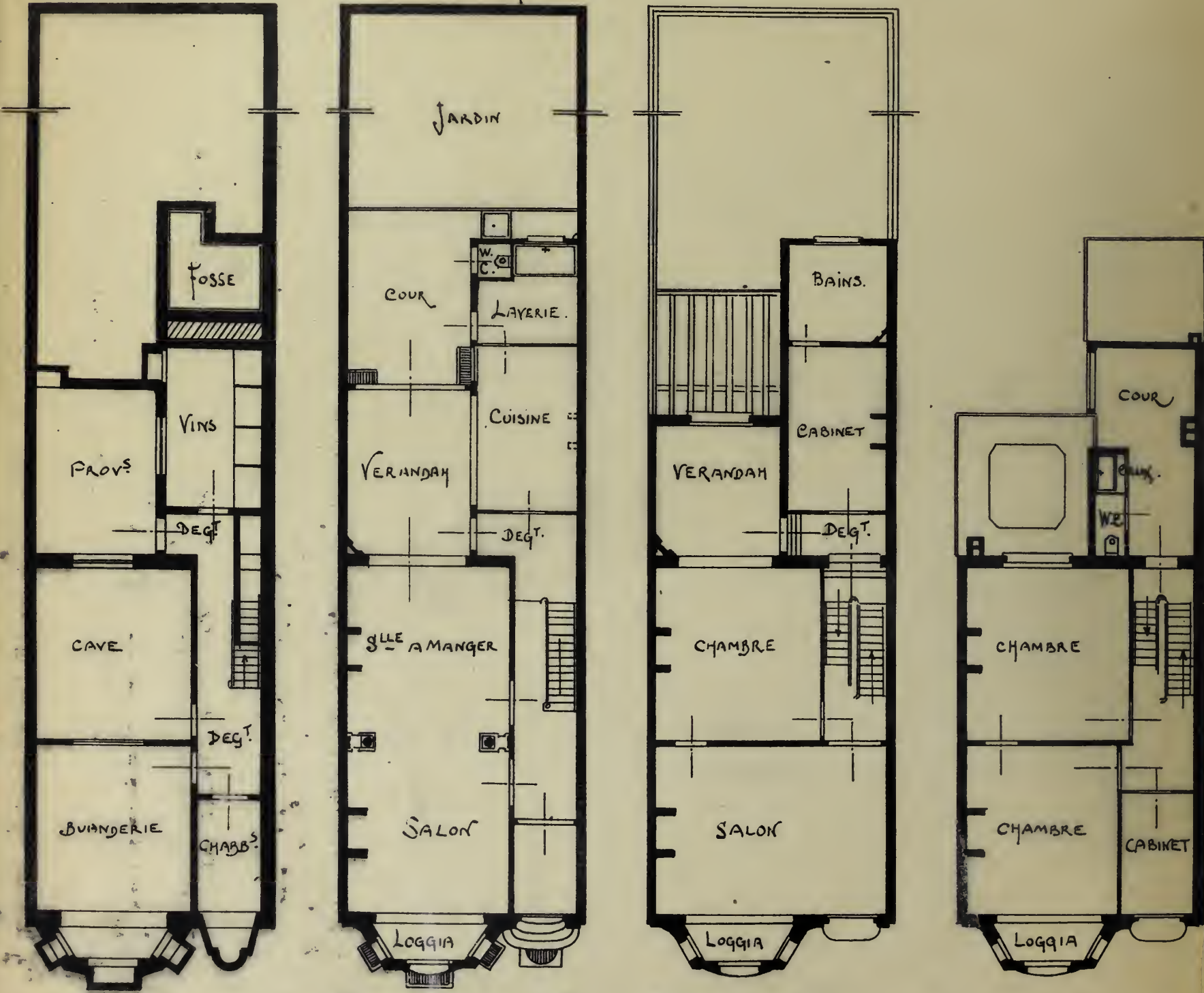
REZ-DE-CHAUSÉE
