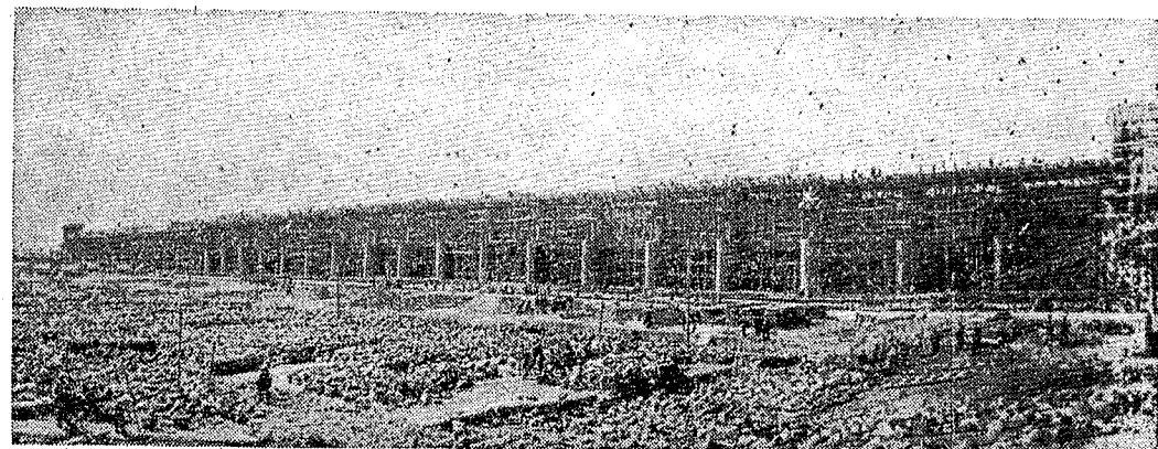
治淮主要工程之一的射陽湖灌溉工程正在加緊施工。這座灌溉工程在江蘇省里下河地區射陽湖的大壩，按照設計，開全長40多公里，35孔。這座大壩將比原計劃提前1個月在5月底完工。灌溉工程修成後，可使里下河地區和海鹽區1,400萬畝土地免遭旱澇，並且可以免除一定程度的暴雨災害。圖為正在施工中的射陽湖灌溉工程。
