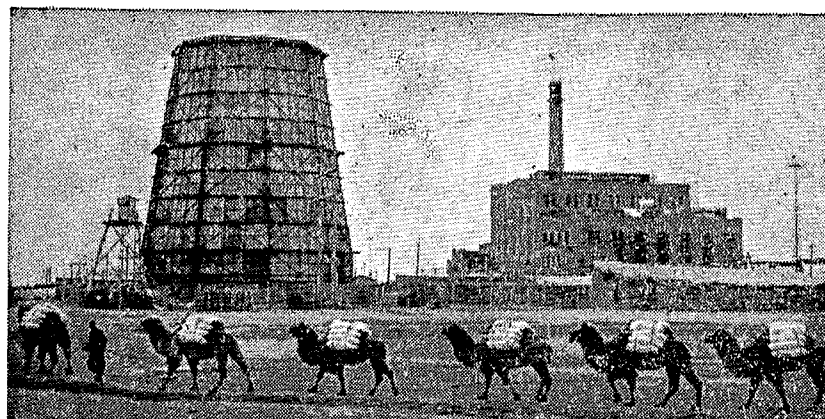
包頭發電廠的擴建工程在3月底提前一個月完成了全部安裝工程約75%，原來計劃在5月1日投入生產的一部新發電機已提前在4月10日發電。廠房的擴建部分全部投入生產後，發電能力將比原有電力增加3倍。這是擴建中的包頭發電廠外景。
