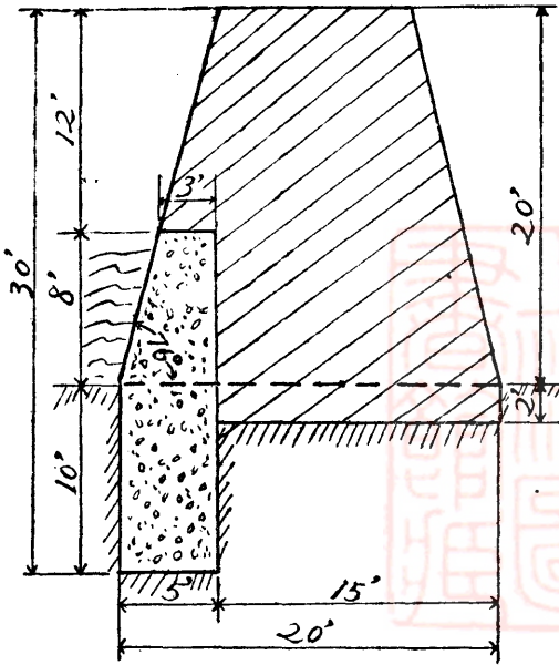
石壩切面圖 比例尺 1"=10'
