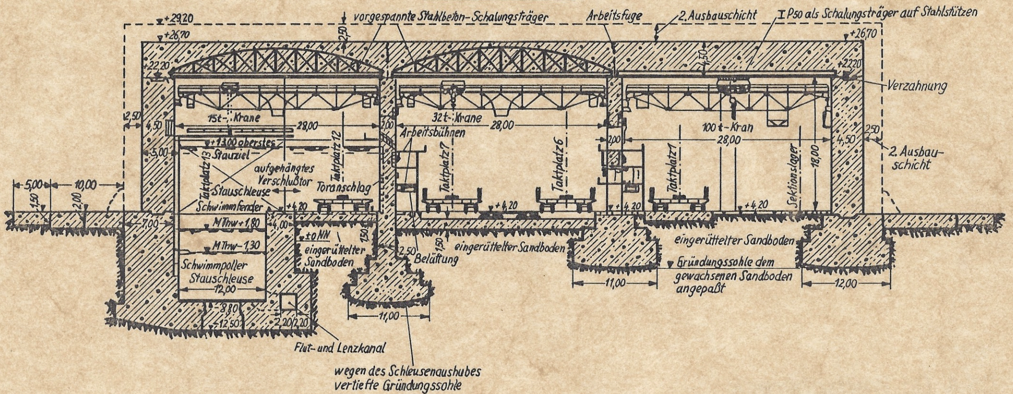
Schnitt A-B 0 5 10 15 20 m
