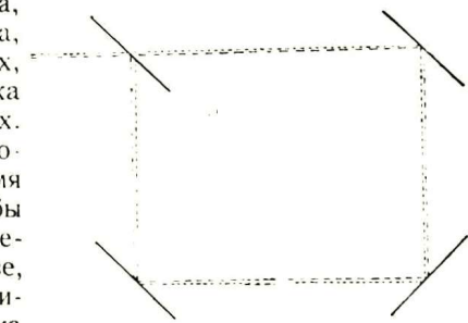
Расположение зеркал в опыте Майкельсона. Черт. 1.
