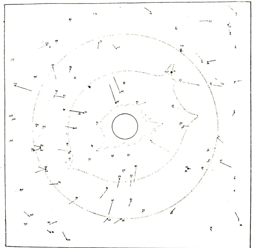
Масштаб карты. Смещение звезд, наблюдавшееся во время полного затмения 1922 г. Масштаб смещения звезд. Черт. 2.
