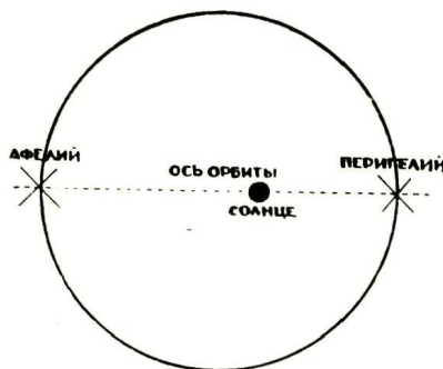
Орбита Меркурия вокруг Солнца. Черт. 4.
