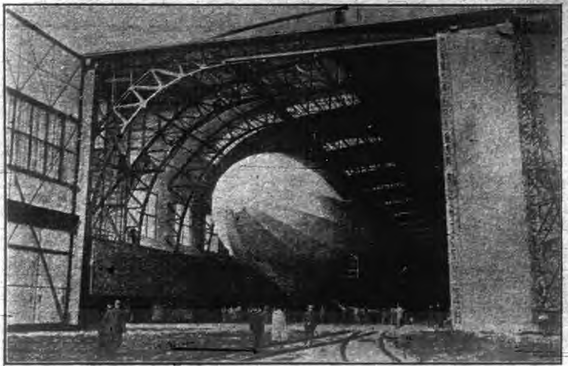
德國皮藏徐柏林飛艇之房屋
