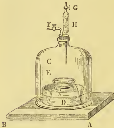
Fig. 16. — Appareil de Schloësing, modifié par Deville. — AB, plaque de verre ; D, cristallisoir ; E, capsule ; H, pipette ; G, robinet.
