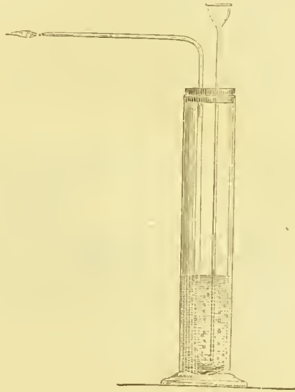
Fig. 8. — Appareil de Marsh, modifié par Chevallier.
