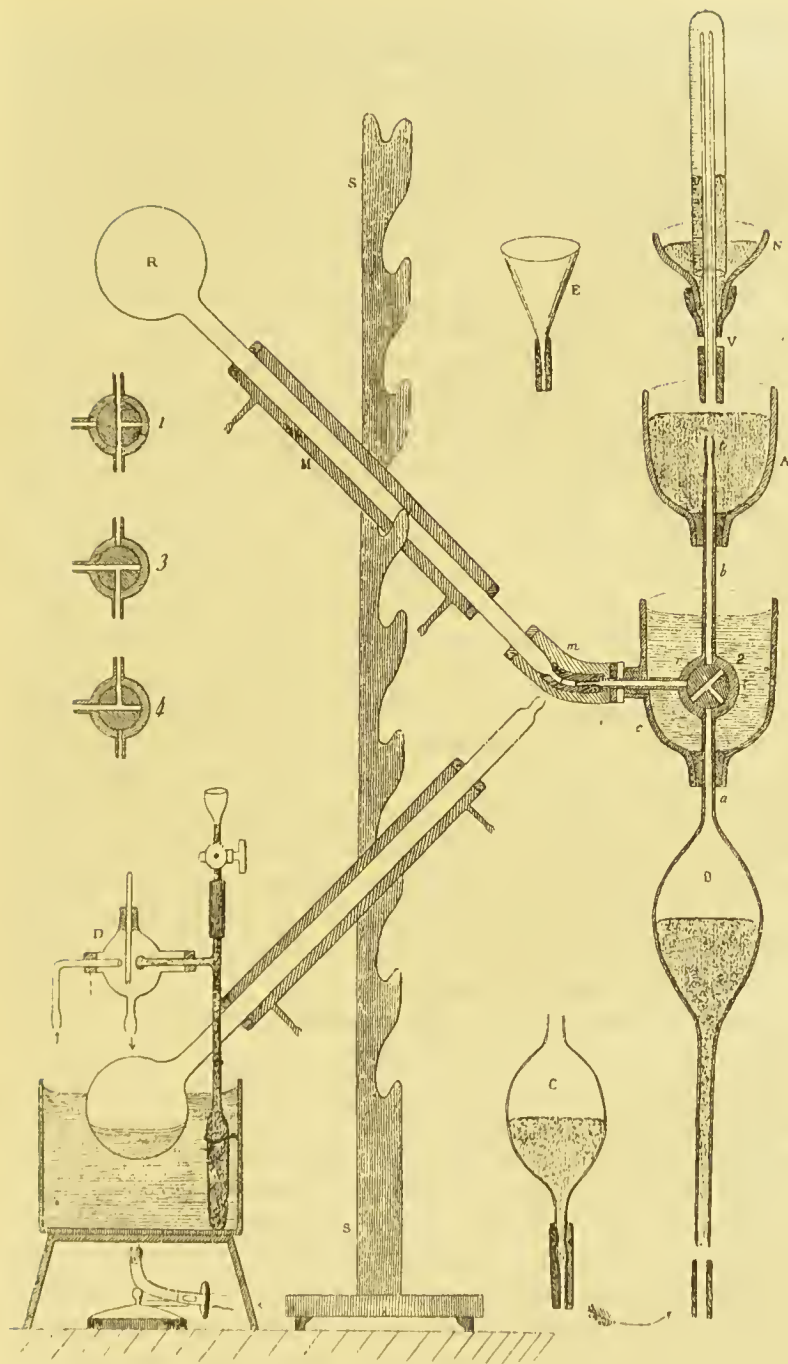
Fig. 28. — Pompe à mercure (Gréhan).
