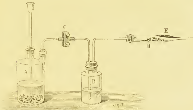
Fig. 12. — Appareil de Fresenius et Babo.
