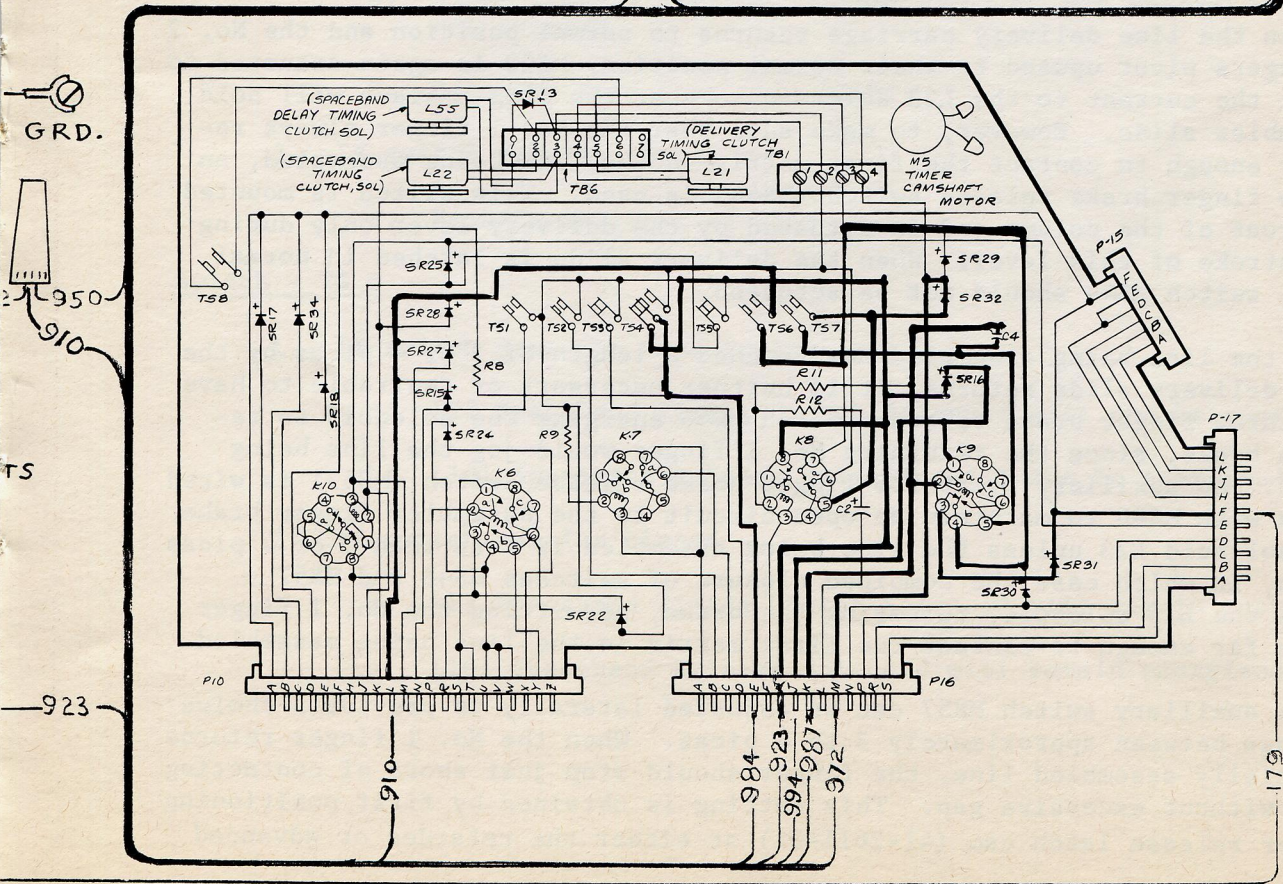
WIRING DIAGRAM FIG. 20
