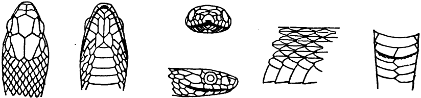
FIG. 269. STORENIA OCCIPITOMACULATA STORER. X 2.
