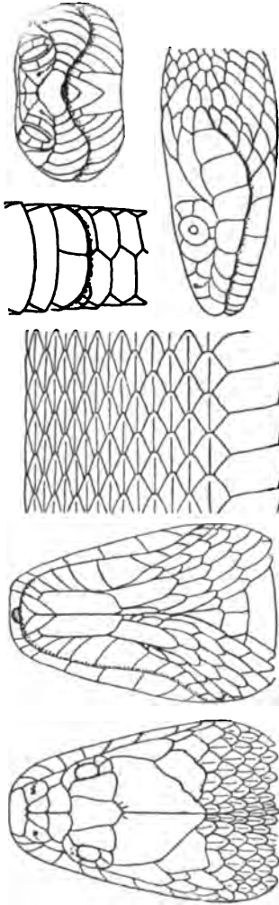
FIG. 248. NATRIX CYCLOPIUM DUMÉRIEL AND BIBRON.
