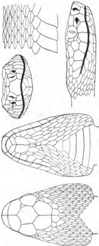
FIG. 325. ANCISTRODON PISCIVORUS LACEPÈDE. X. 66 Cat. No. 8946, U.S.N.M.
