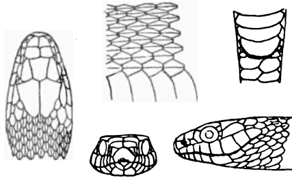
Fig. 285. EUTÆNIA INFERNALIS VIDUA COPE. = 1.
