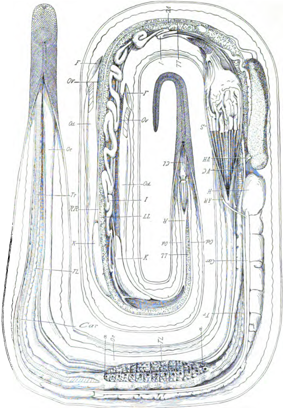
VISCERA OF CHERSYDRUS GRANULATUS MERREM.
