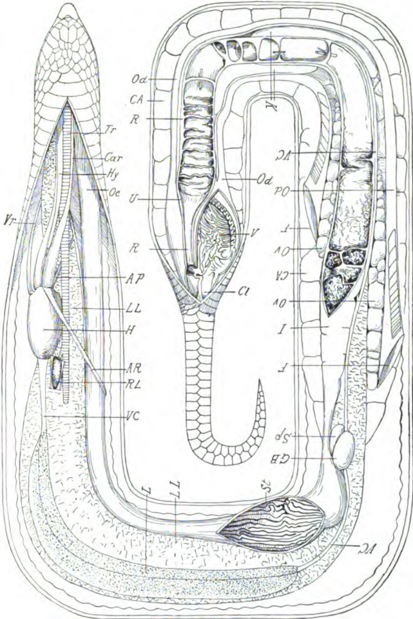
VISCERA OF HETERODON PLATYRHINUS LATREILLE.
