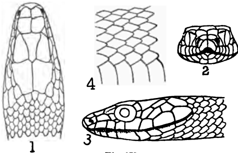
Fig. 179. ZAMENIS AURIGULUS COPE. = 1.
