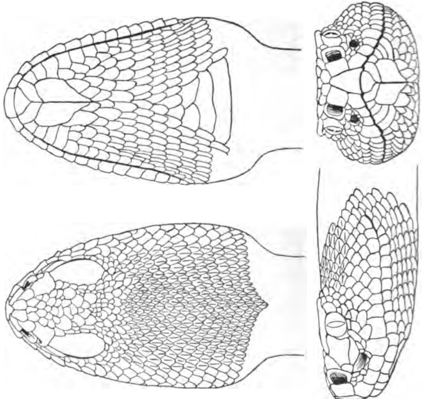
Fig. 383. CROTALUS ADAMANTEUS ADAMANTEUS BEAUVOIS. = 1.
