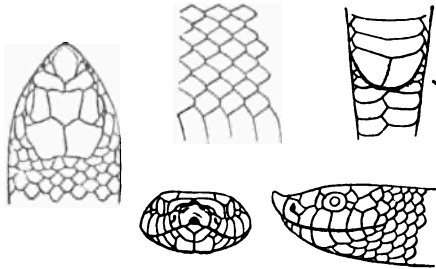
Fig. 241. GYALOPIUM CANUM COPE.
