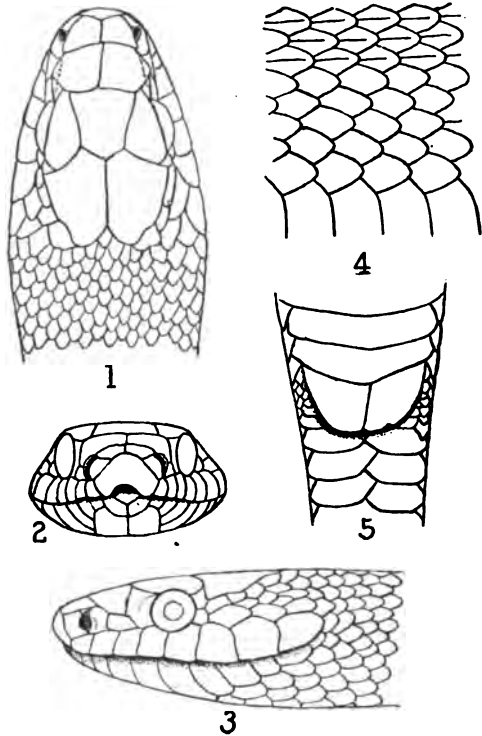
Fig. 194. COLUBER OBSOLETUS SAYI.
