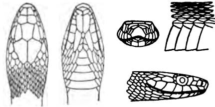
Fig. 298. EUTÆNIA SIRTALIS GRAMINEA COPE.
