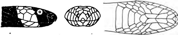
Fig. 322. ELAPS FULVUS LINNÆUS. = 1.
