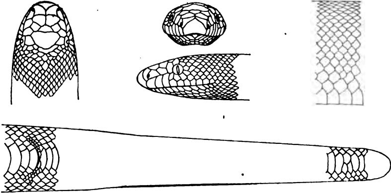
Fig. 149. CHARINA BOTTÆ BLAINVILLE. × 1.5. Summer Lake, Oregon. E. D. Cope.
