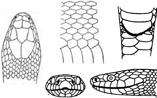
Fig. 223. OPHIBOLUS CALLIGASTER SAY. = 1. St. Louis, Missouri. Cat. No. 1629, U. S. N. M.
