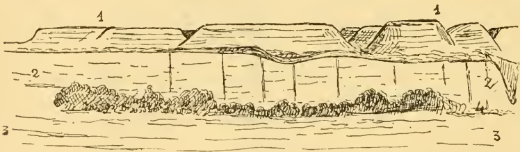
Fig. 3. a —Panorama de las terreras y de los páramos, visto desde La Campiña.
