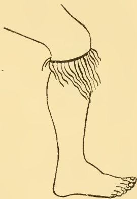
Fig. 3. a —El «Ponor» de Timor, según un dibujo de Riedel.
