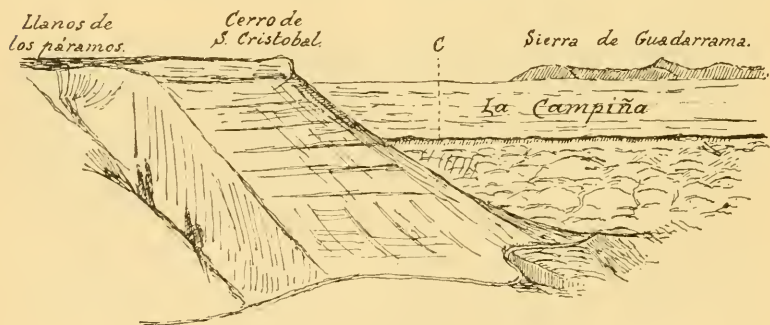
Fig. 6. a —Panorama desde la ladera N. W. del páramo del Sotillo, para que se vean la posición de estos tres escalones: páramos, terraza cuaternaria y La Campiña. C, Borde de la terraza (760 m.) á 40 m. sobre el Henares. Cumbre del Cerro de San Cristóbal (932 m.). Apunte del natural.
