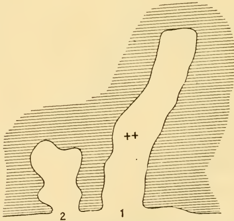
Fig. 5. a —1, cueva de San Jorge en Niéva de Cameros.—2, cueva innominada, del mismo lugar.— ++, sitio donde se hallaron huesos y cerámica.
