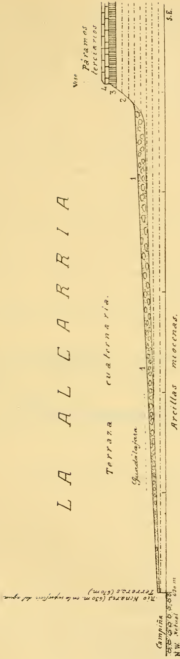
Fig. 2. a —Corte transversal, de N. W. á S. E., de La Campiña á los paramos terciarios de La Alcarria.
