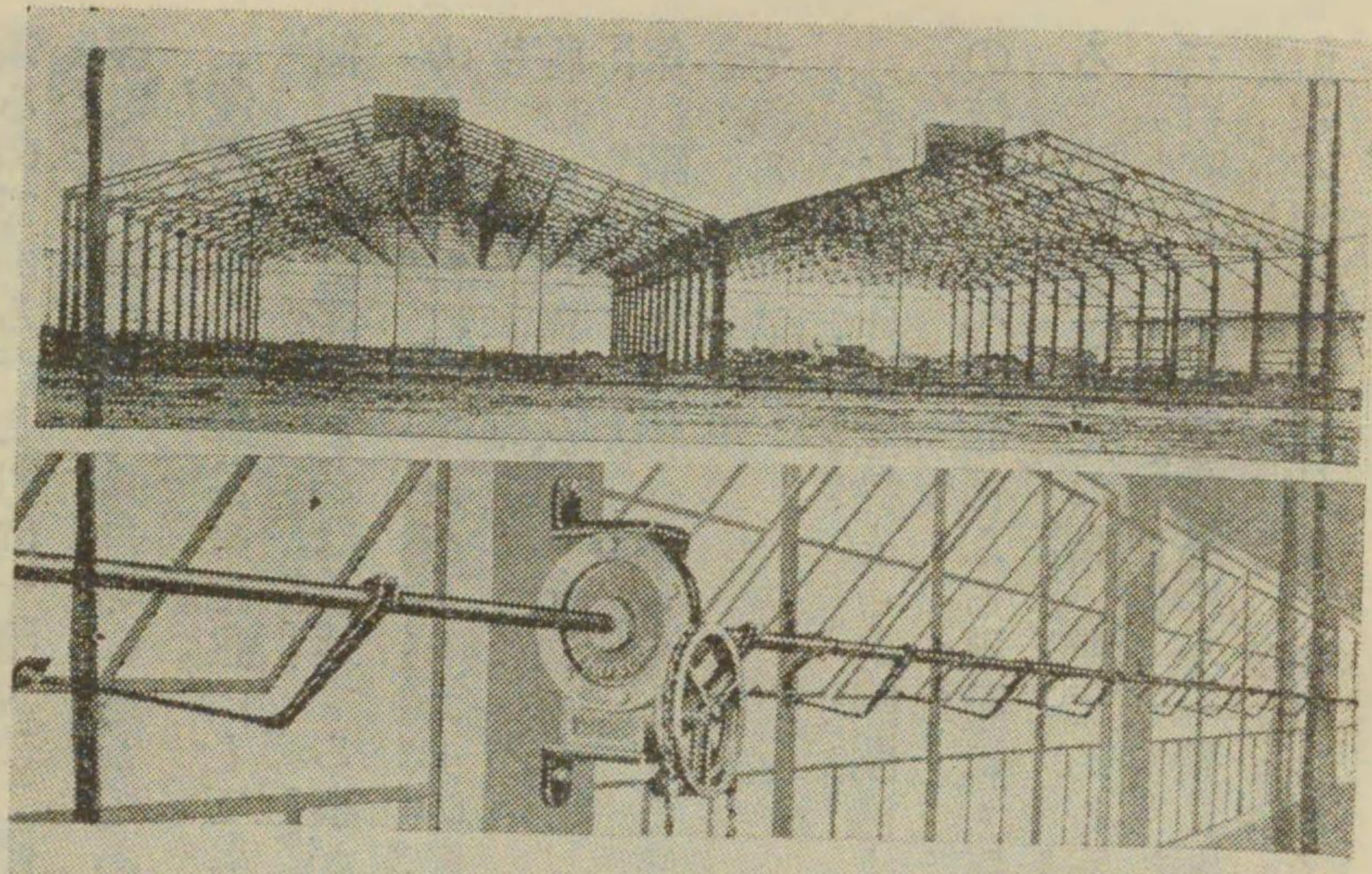
鋼製建物の骨組とみ連続密接の閉開装置
