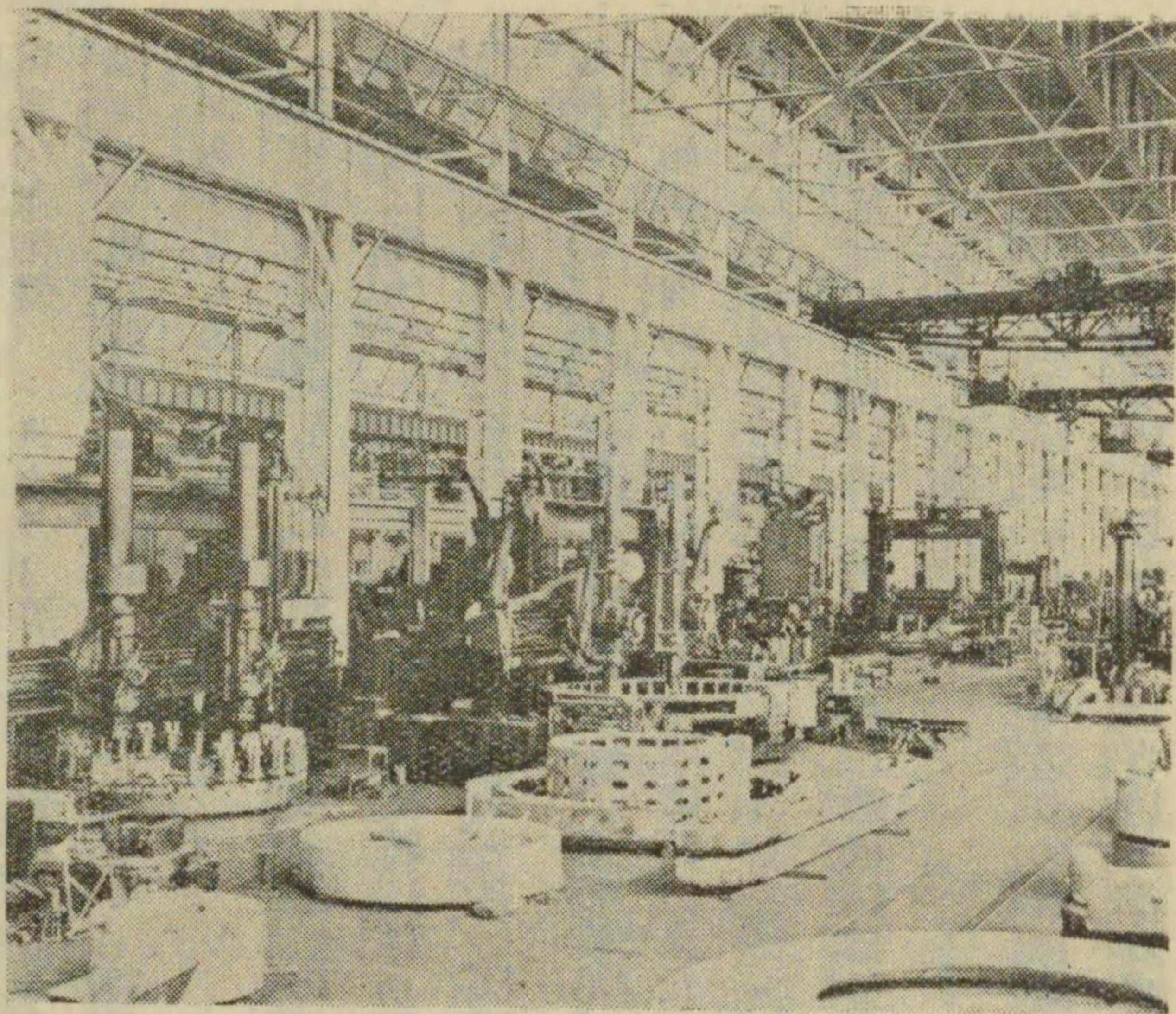
廻轉機工場の一
