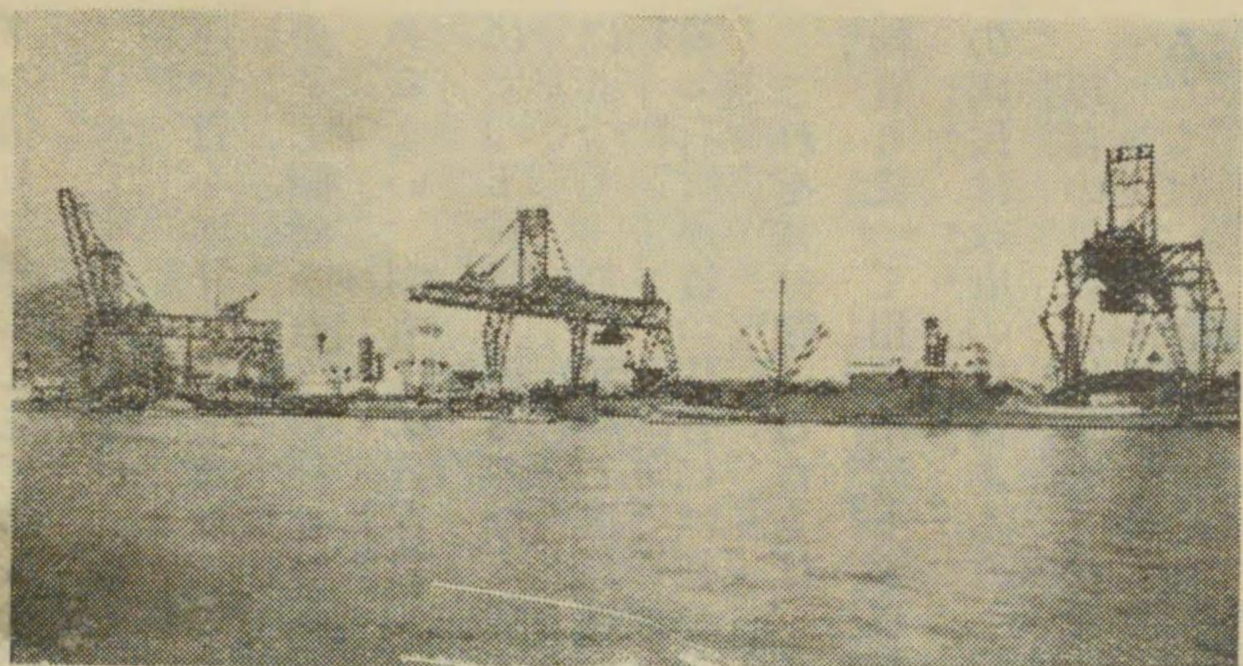
上海より見たる鶴見工業地帯の一部三井埠頭の設備
