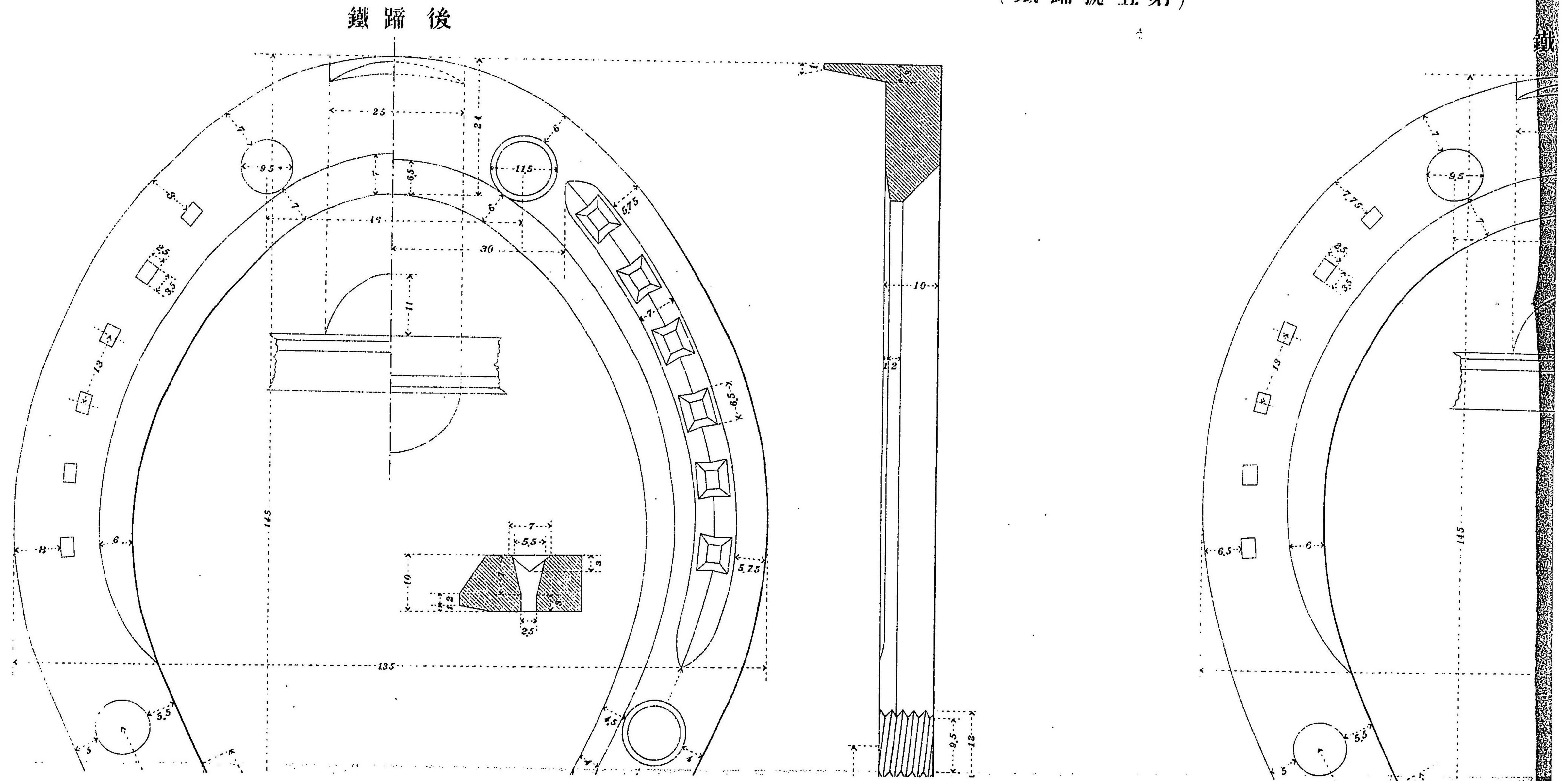
圖 二 第 (鐵 蹄 上 水) 五 其 (鐵 蹄 號 五 第)
