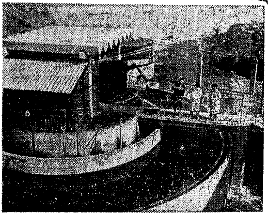
湘潭纺织印染厂成立专门班子进行实验，认真研究解决生产中排出的大量污水。图为该厂的污水净化人员在提取污水进行分析。
