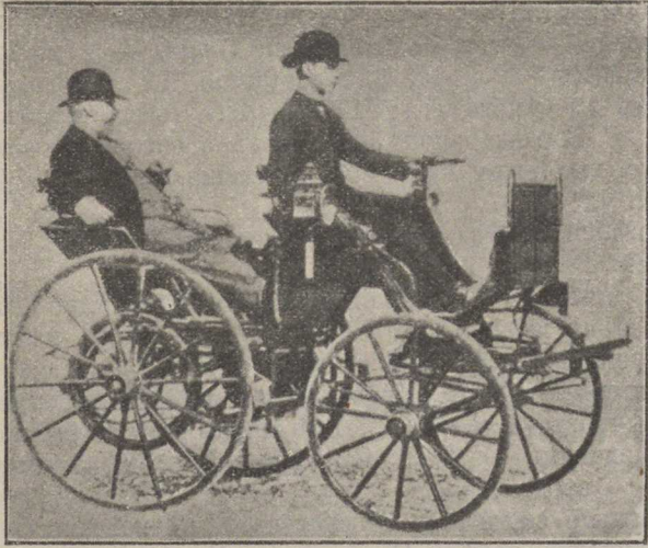
Первый автомобиль съ бензиновымъ моторомъ Даймлера.
