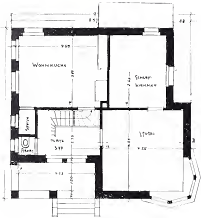
Erdgeschoß.
