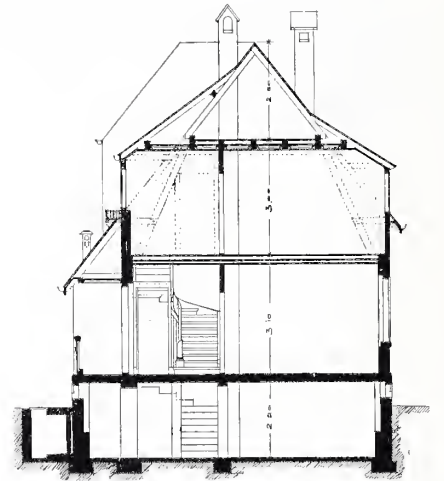
Schnitt.
