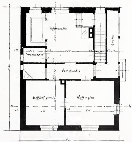
Erdgeschoß.
