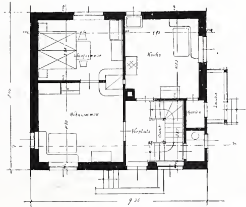
Grundriß-Erdgeschoß.
