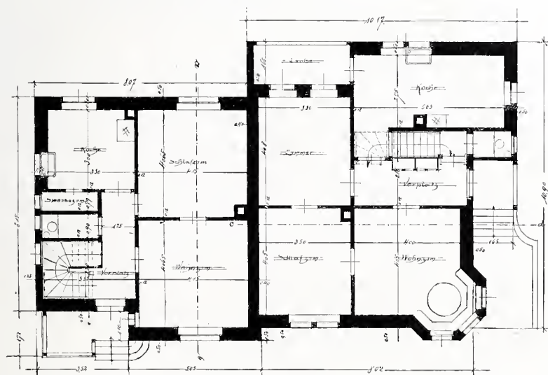
Erdgeschoß.
