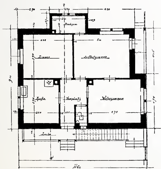
Erdgeschoß.
