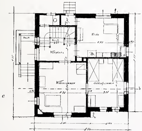
Erdgeschoß.
