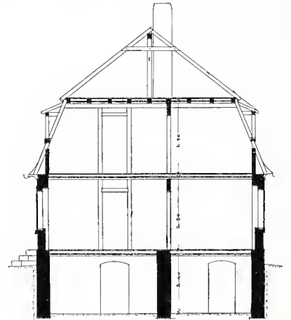
Schnitt.
