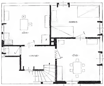
Obergeschoss.
