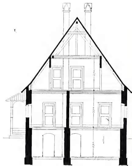
Querschnitt.
