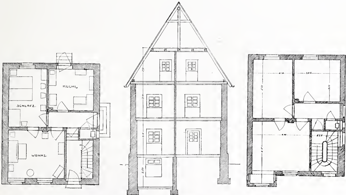
Querschnitt.
