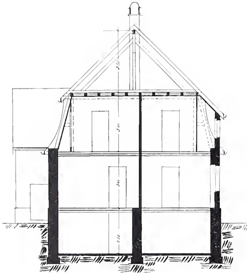
Querschnitt.
