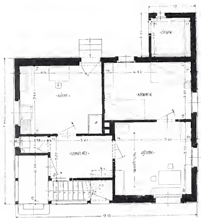
M. 1:200
