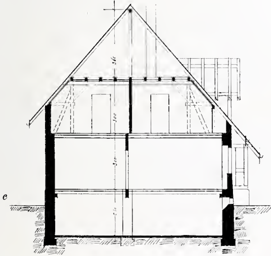
Querschnitt.
