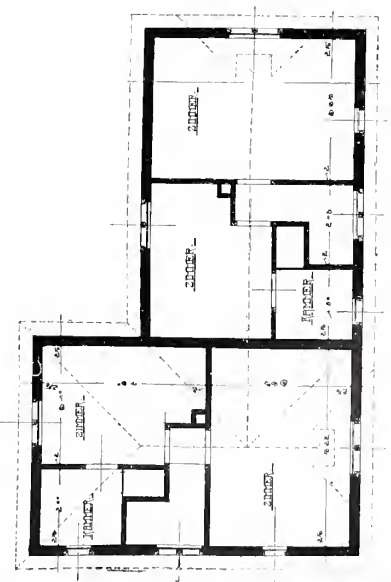
Obergeschoss.
