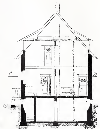
Querschnitt.
