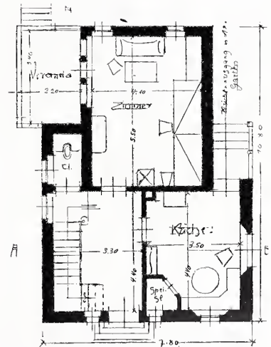
M. 1:200
