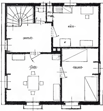
Obergeschoß.
