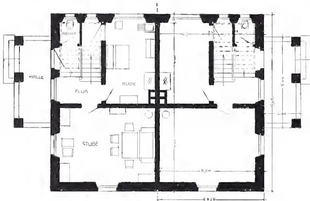
Erdgeschoß.
