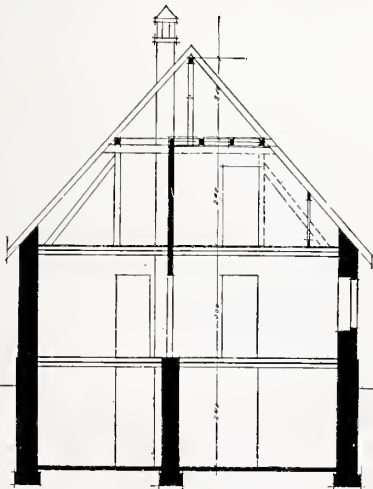
Querschnitt.
