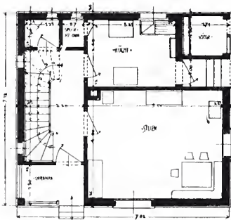
Obergeschoß.
