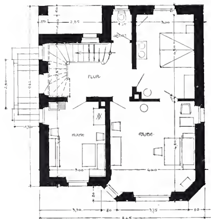
Erdgeschoß.
