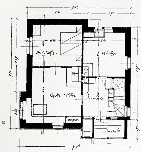
Erdgeschoß.
