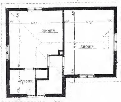
Obergeschoß.
