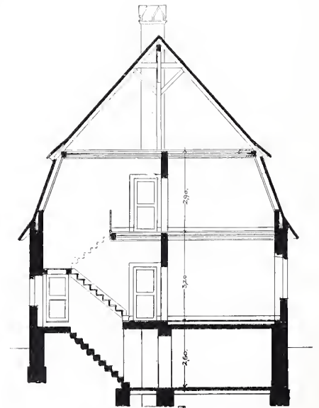
Querschnitt.
