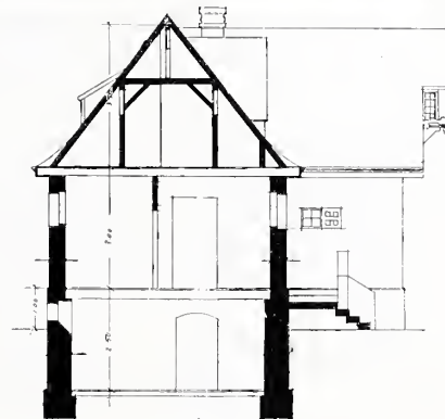
Schnitt.
