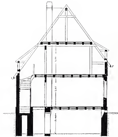
Schnitt.
