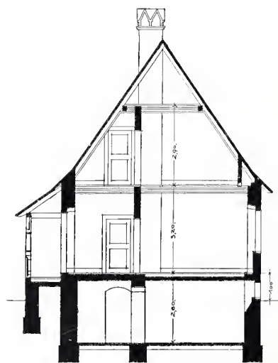
Querschnitt.
