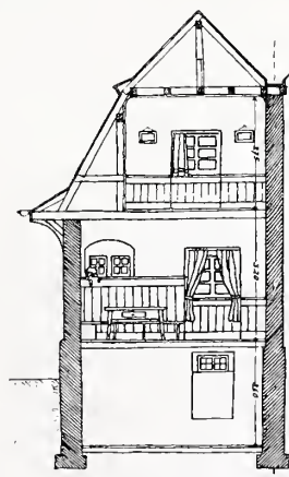
Querschnitt.
