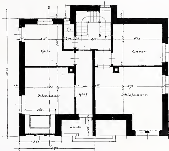
M. 1 : 200
