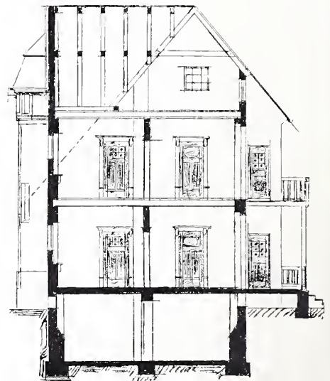
Querschnitt.
