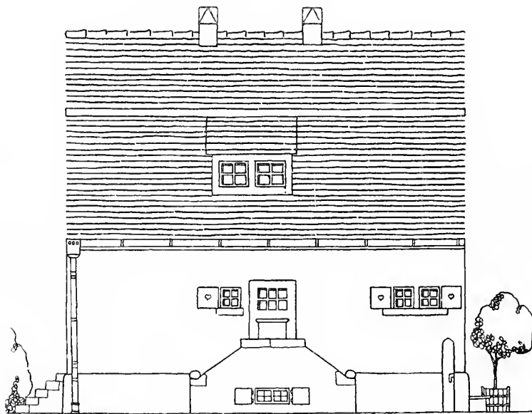
Seitenansicht.
