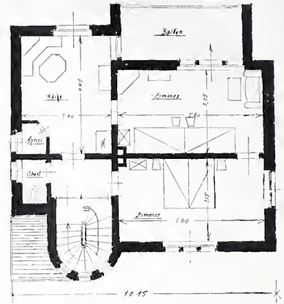
Obergeschoss.
