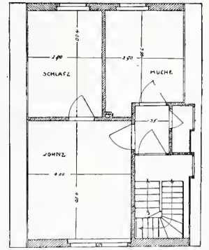
Obergeschoss.
