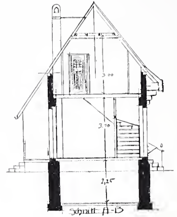
Querschnitt.
