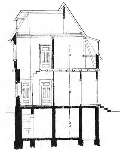
Schnitt.
