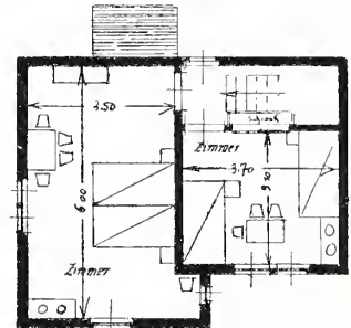
Obergeschoß.
