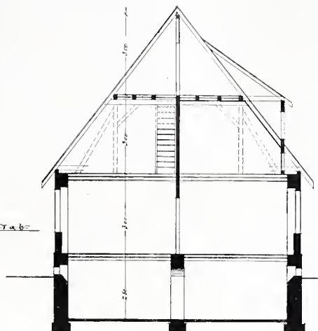
Schnitt des linken Hauses.
