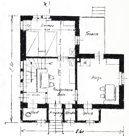
Erdgeschoß.
