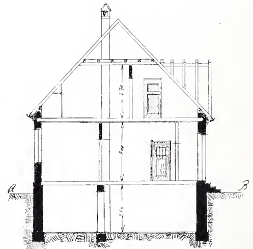
M. 1:200 Querschnitt.
