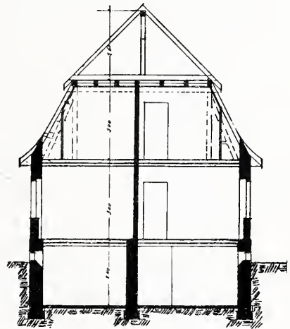
Querschnitt.
