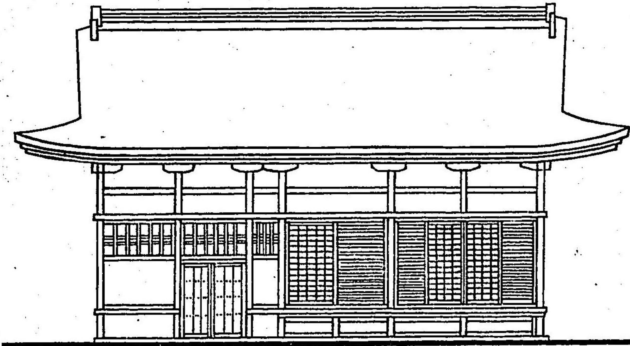
神饌所制限正面図
