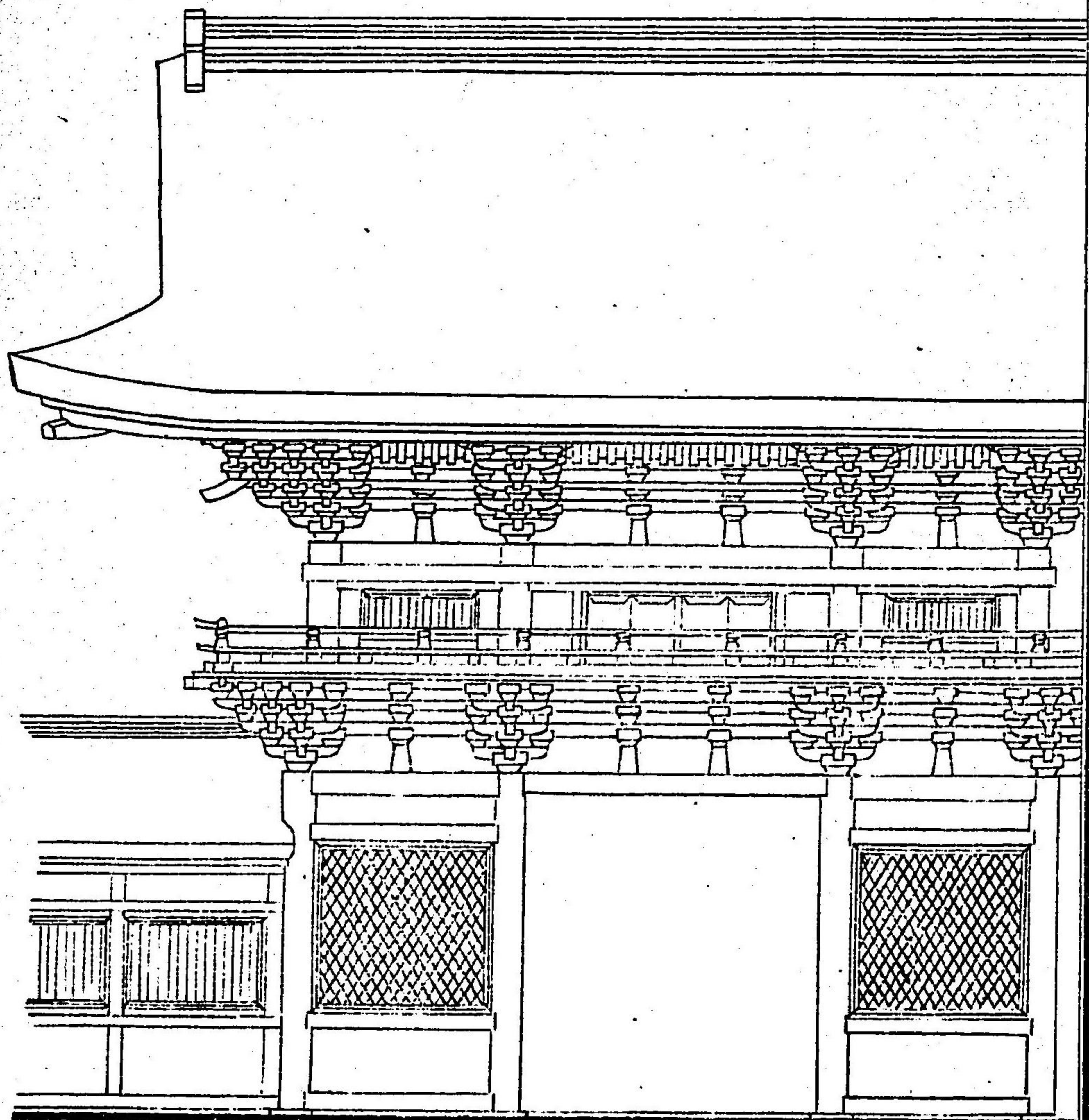
樓門正 面圖
