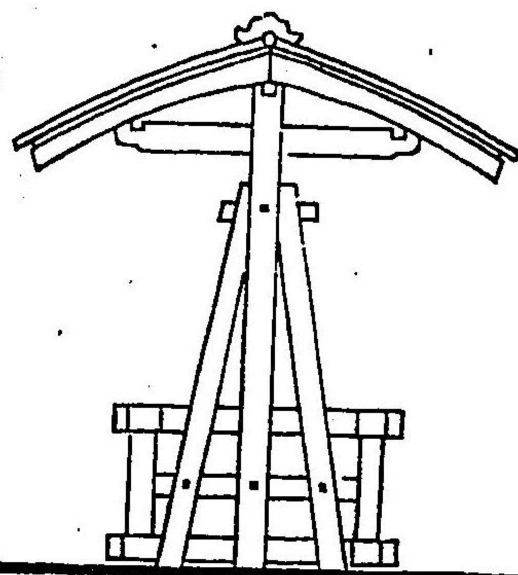
手水舎制限正面圖 井戸屋形制限圖
