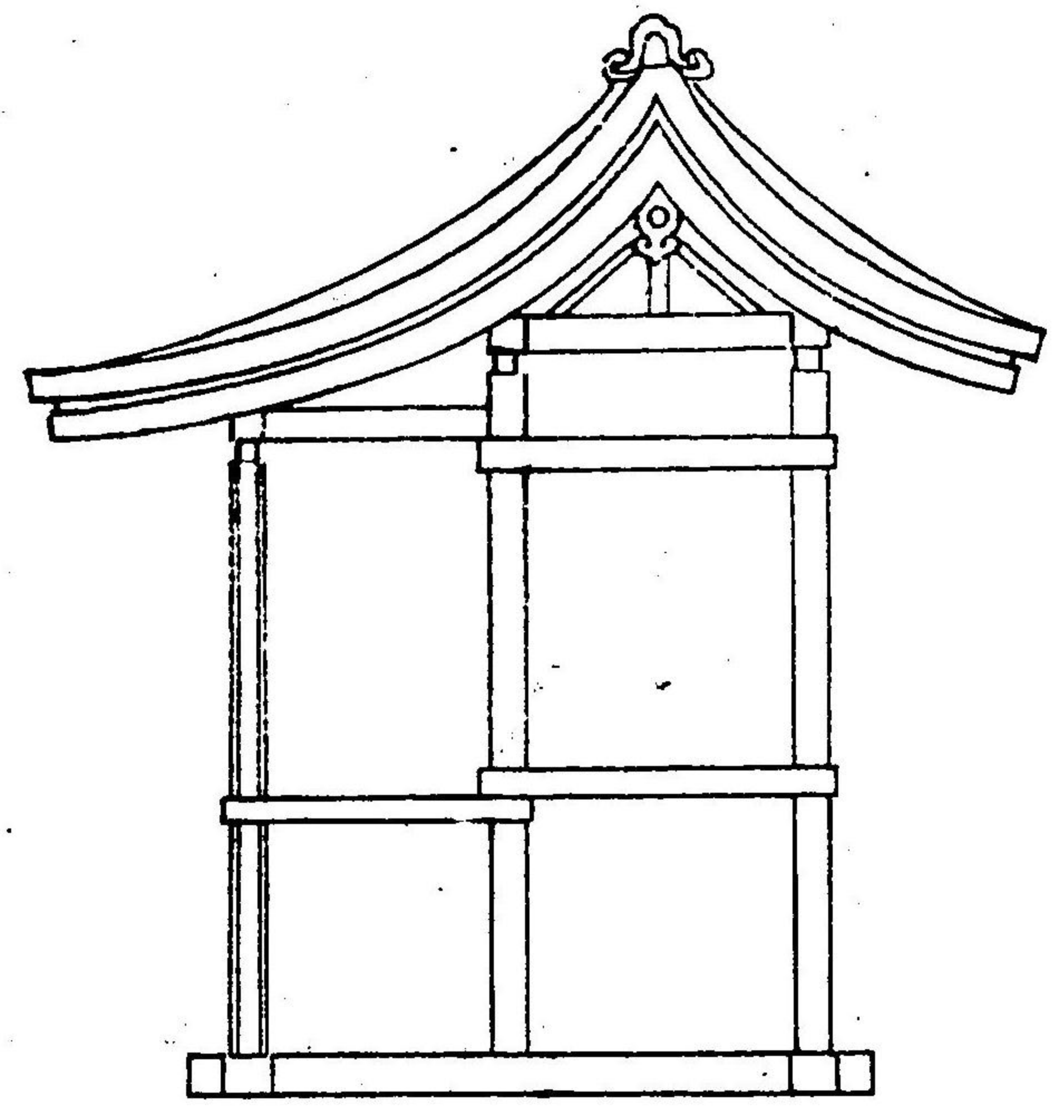
同敷図
