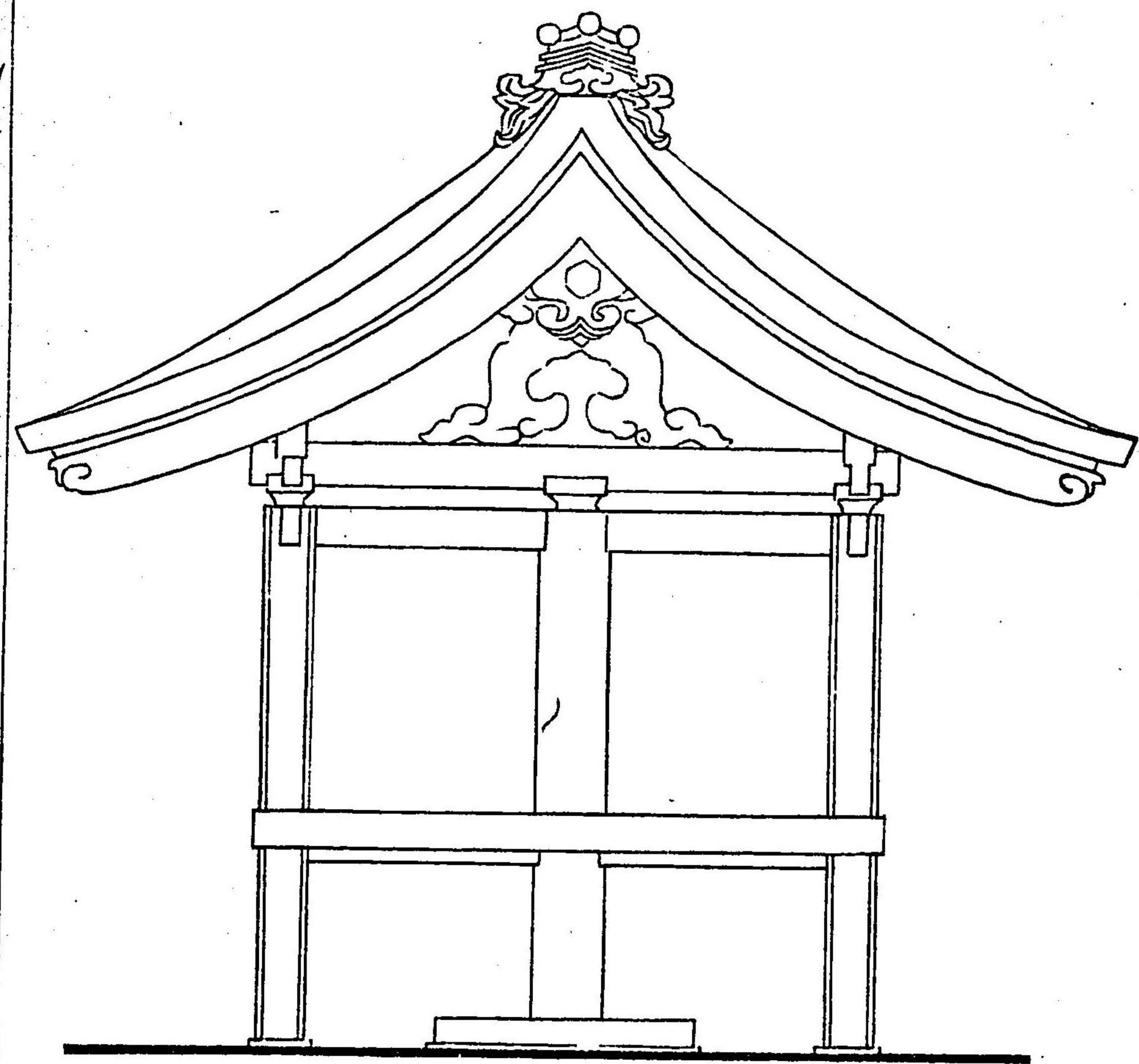
同側面圖
