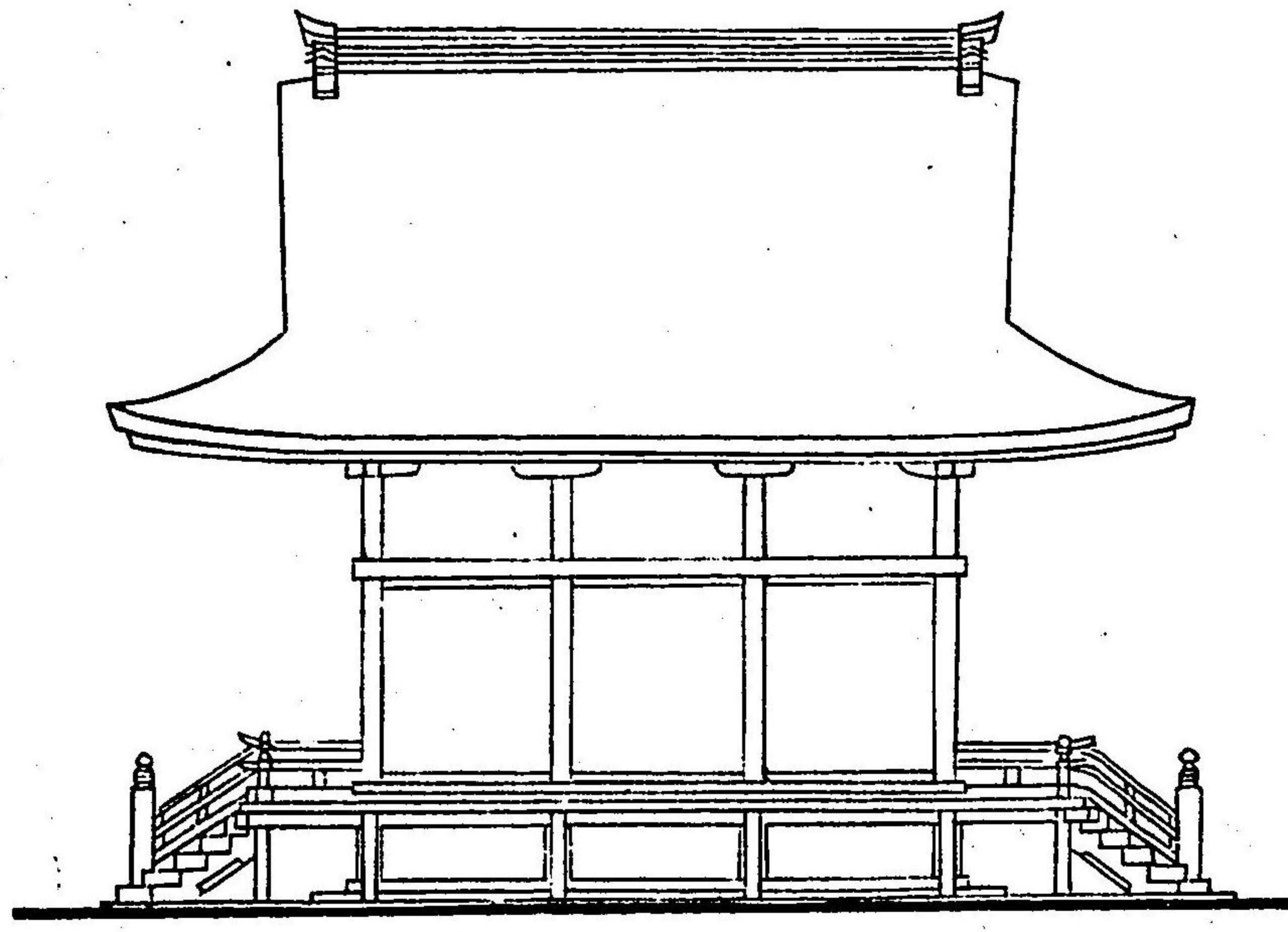
同側面圖
