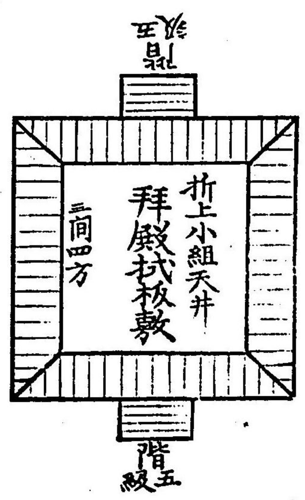
中社拜殿制限敷圖
