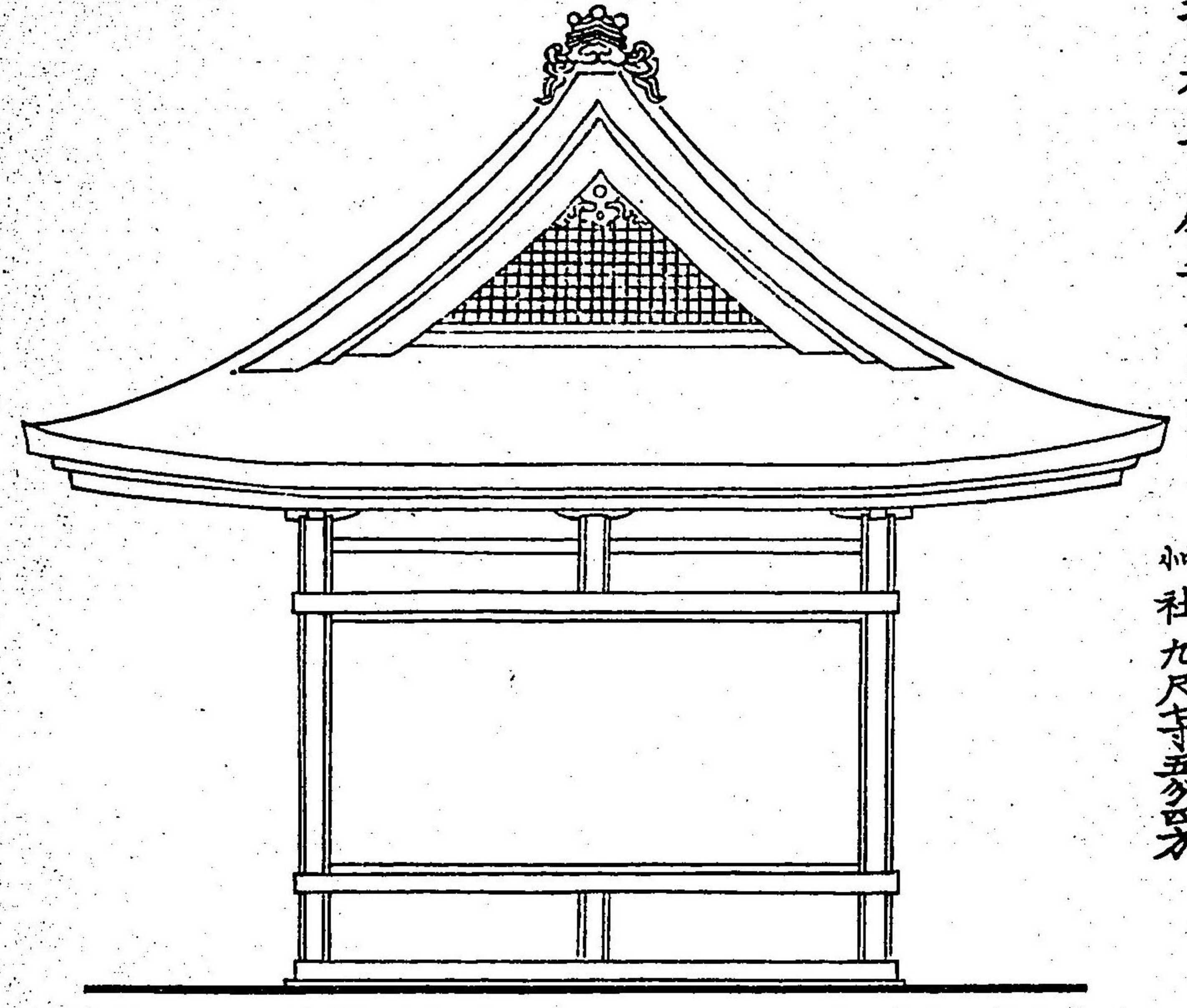
同敷圖
