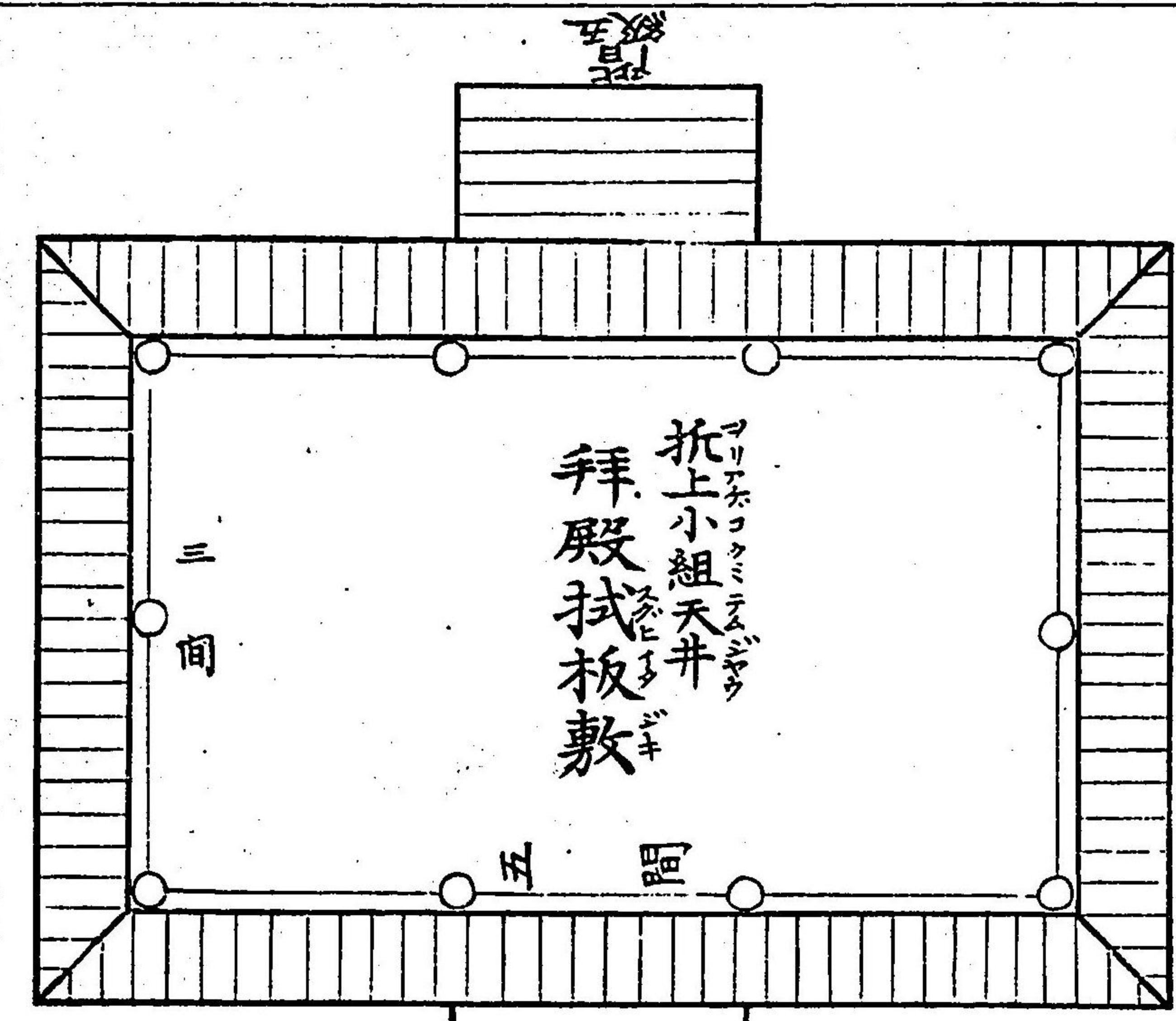
大社拜殿制限敷圖 舞殿とも云ふ
