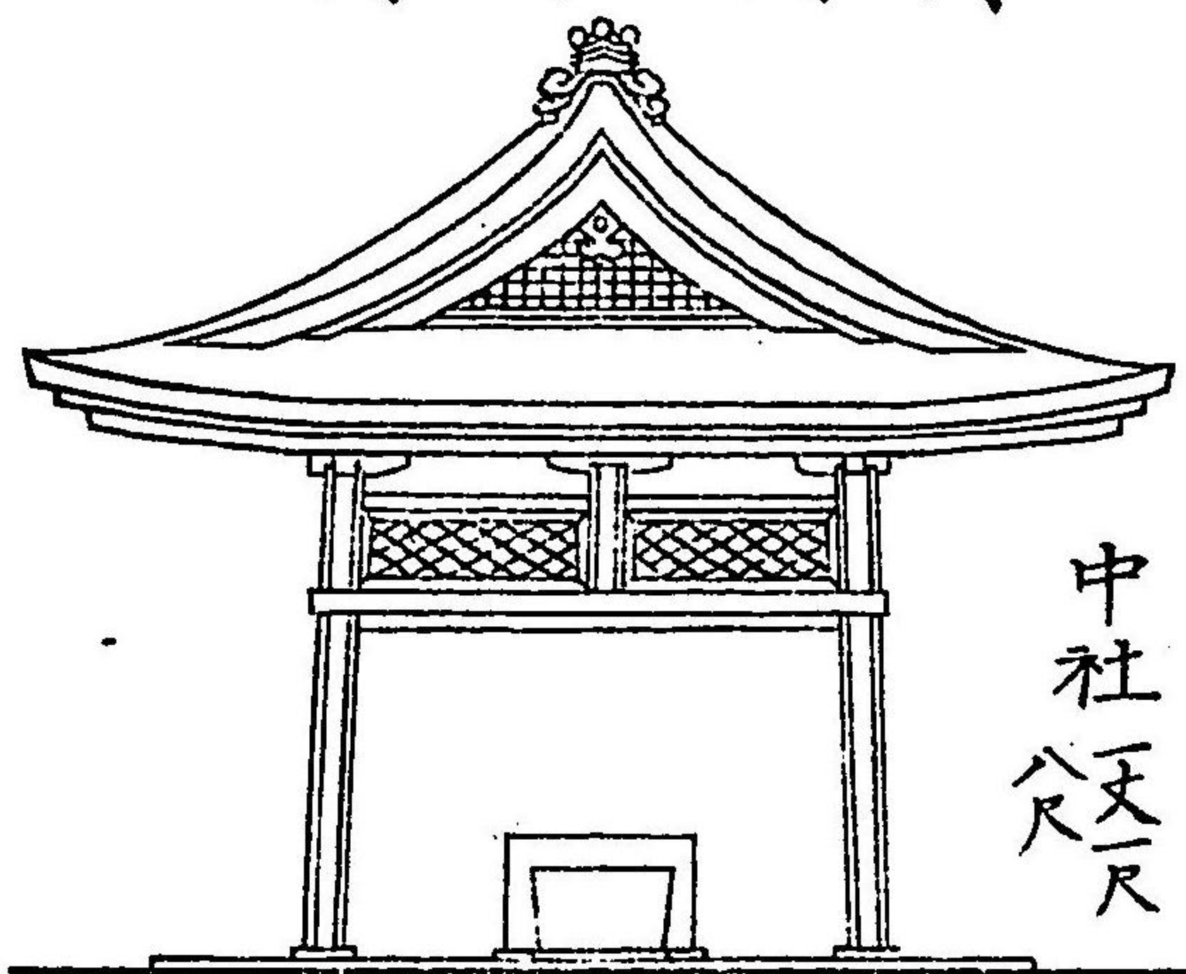
同敷圖
