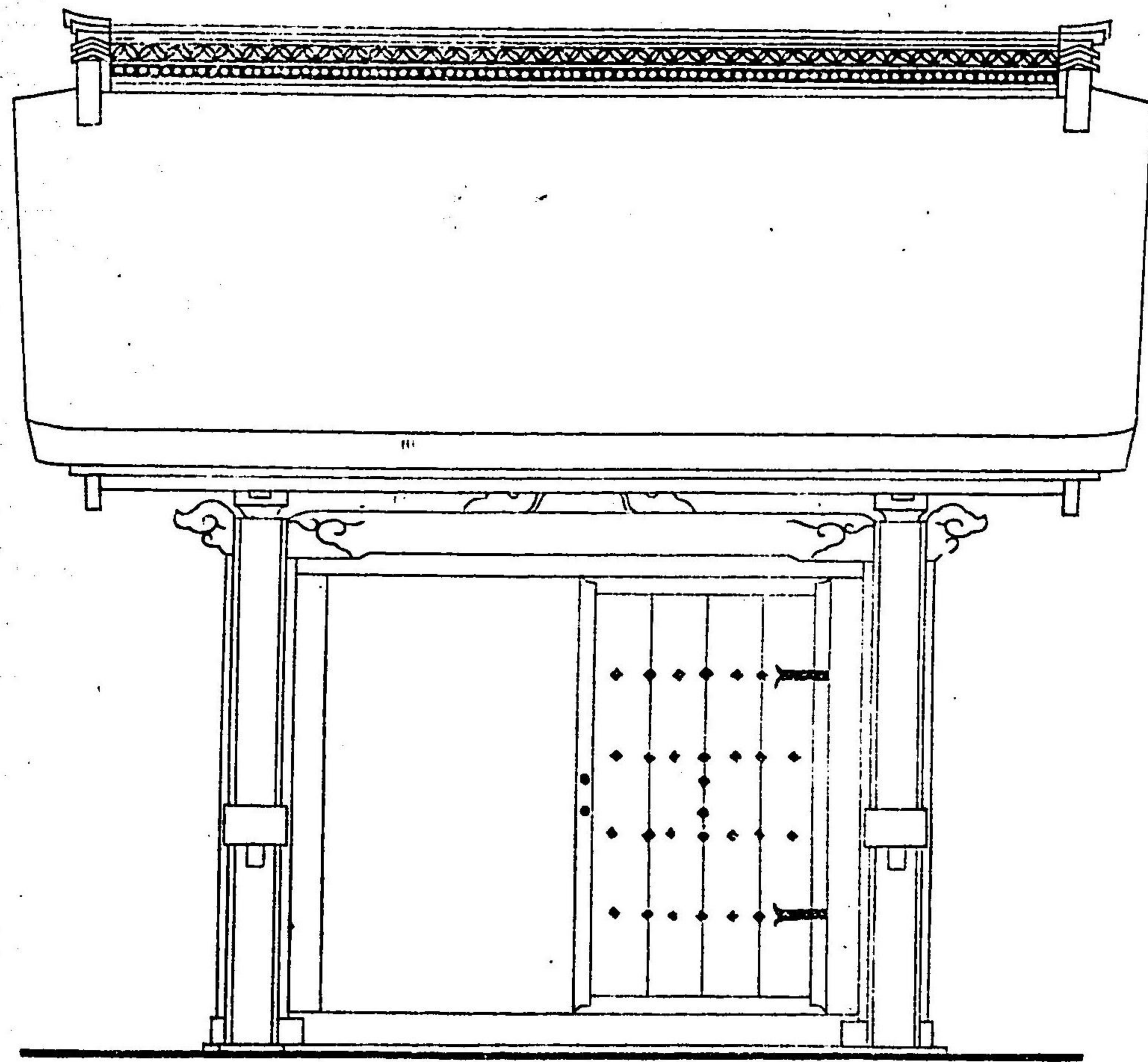
中門正面圖
