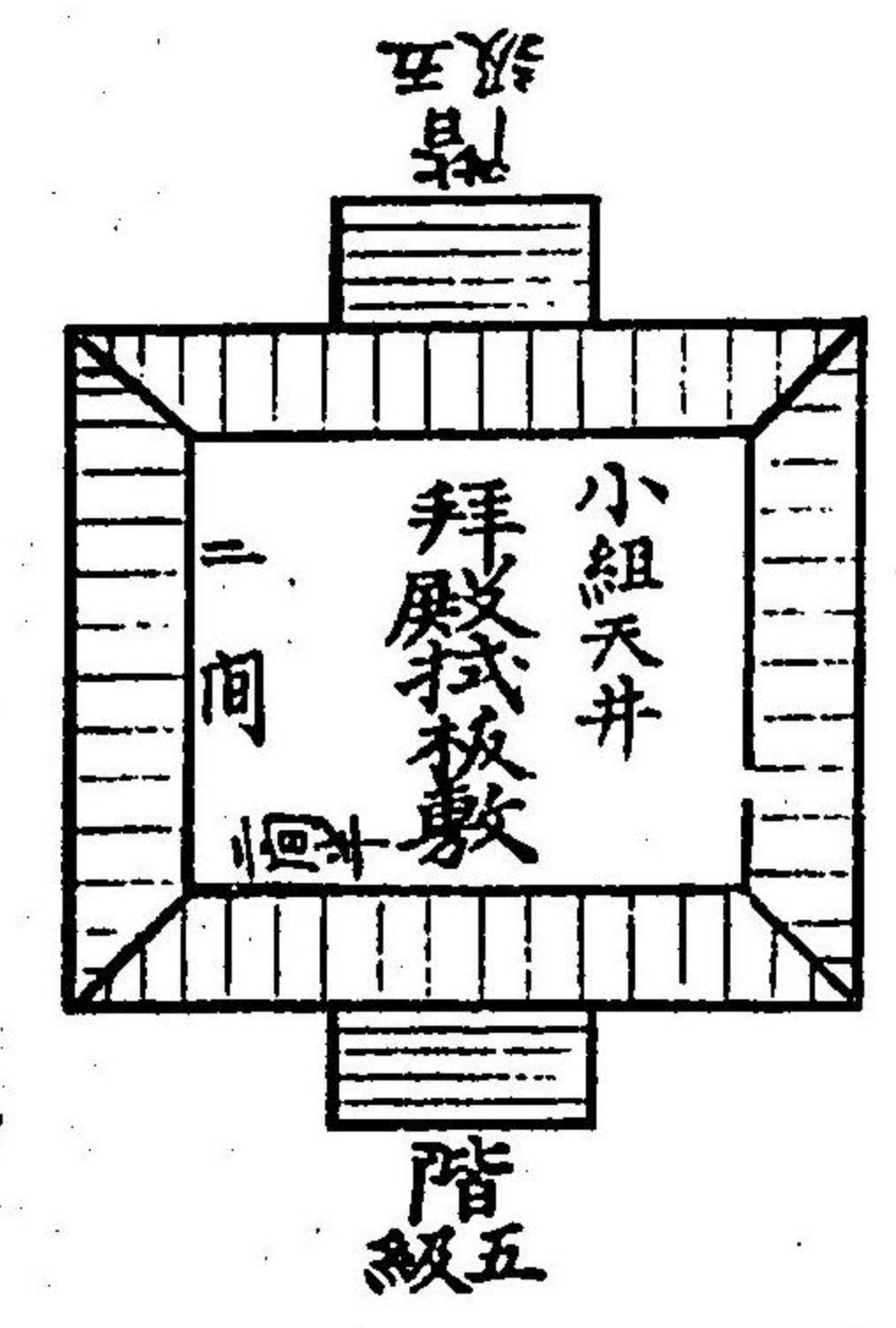
小社拜殿制限敷圖
