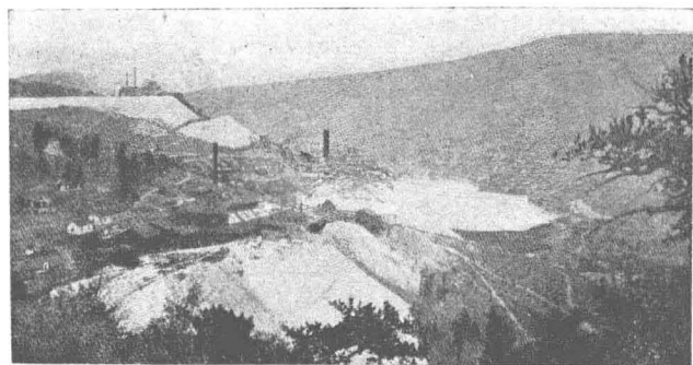
美國的 Cripple Creek, 金礦曾稱霸世界
