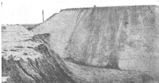
南非 Transvaal 金礦之石山
