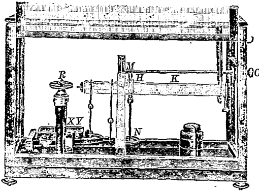
第二五圖 北尾氏剛性試驗器
