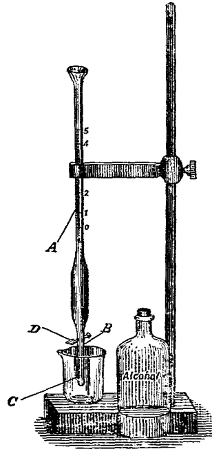
第三六圖 穀粒容積計
