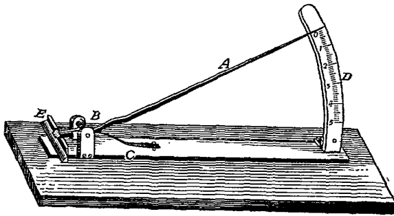
第二八圖 測莖器
