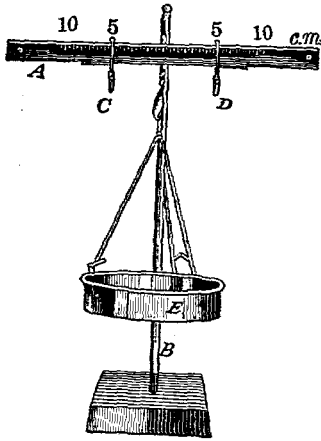
第二九圖 稻莖彈性測驗器
