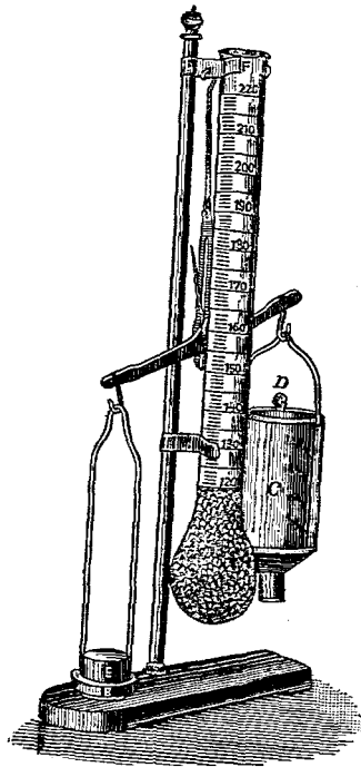
第二一圖 布勞燕氏穀粒檢定器
