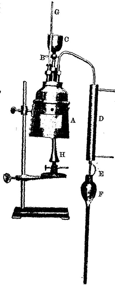
第三二圖 賀富曼氏水分測驗器
