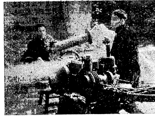
南县浪湖公社农机站应用射流技术研制成功无底筒水泵。这种水泵提高扬程、增大出水量，降低油耗，并且操作简便可靠。因为两水大队在使用无底筒水泵抽水灌溉。
