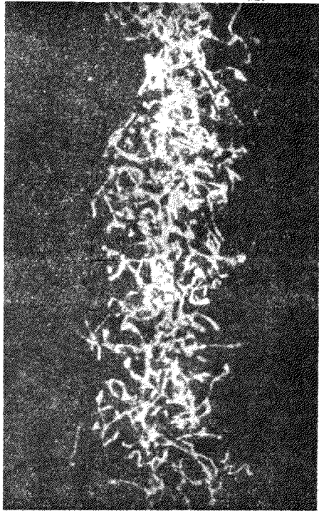
X光經過空氣時所生之電子
