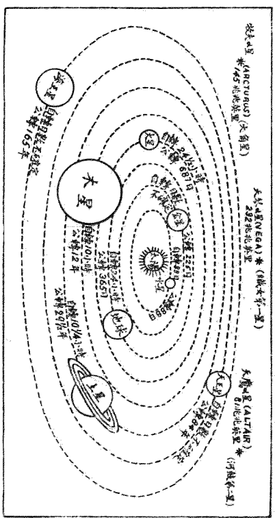
第一圖 太陽系之全圖
