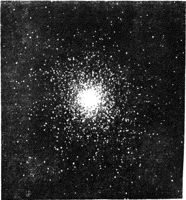
第十七圖 武仙座 (Hercules) 中之星團 (加拿大維多利亞 (Victoria B. C.) 天文臺攝影)
