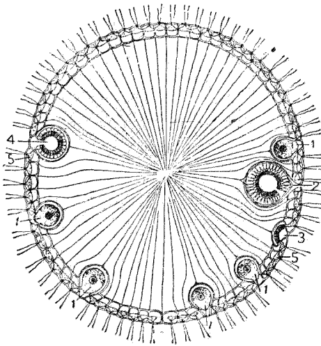
團藻
