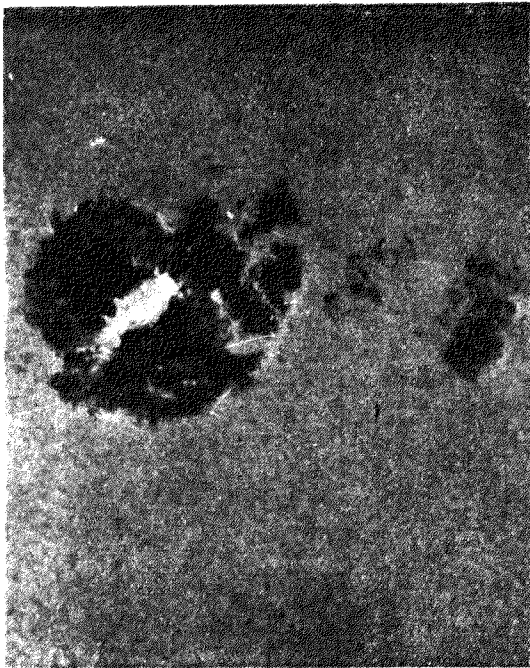
第七圖 一九〇五年七月十七日之大日斑
