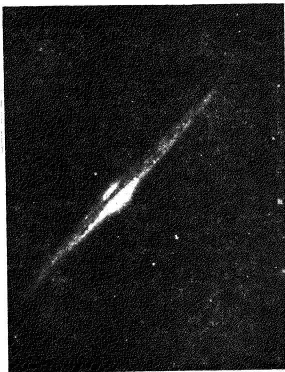
第二十圖 一旋渦星雲之側形(威爾遜山天文臺攝影)
