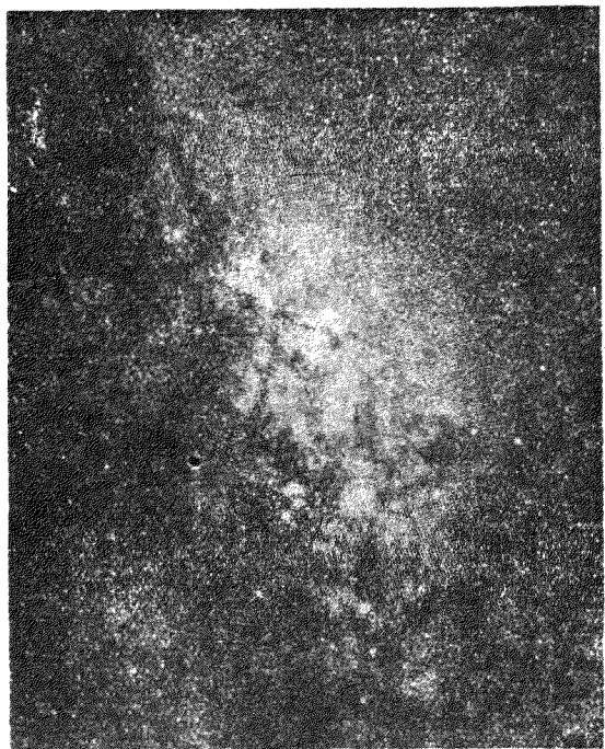
第三圖 天河 (哈佛 Harvard 大學天文臺攝影) 注意星體之密集如雲。
