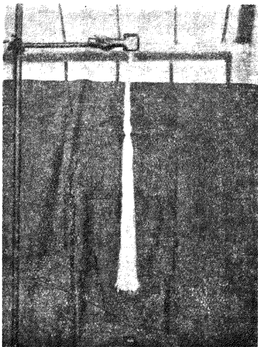
經鈹射線照過後絲縷失電之狀
