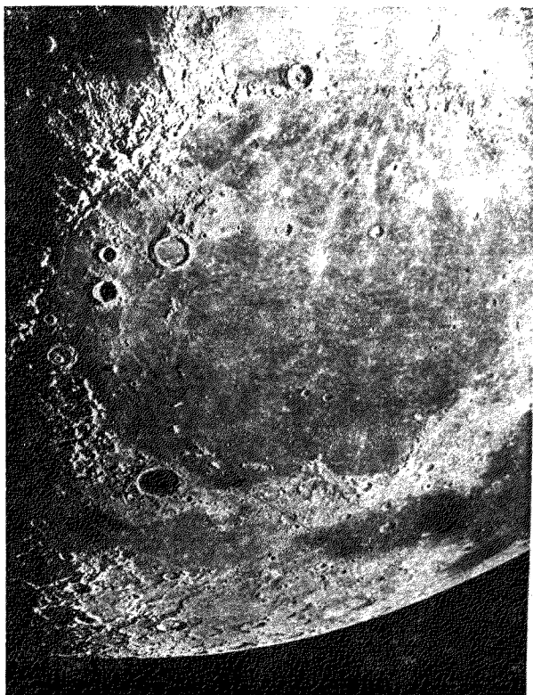
第十三圖 月球
