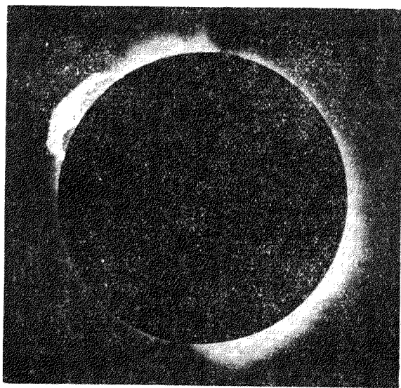
第五圖 一九一九年五月二十九日全蝕時日珥之影攝於巴西 (Brazil) 之索布拉爾 (Sobral) (格林維基 (Greenwich) 皇家天文臺攝影)
