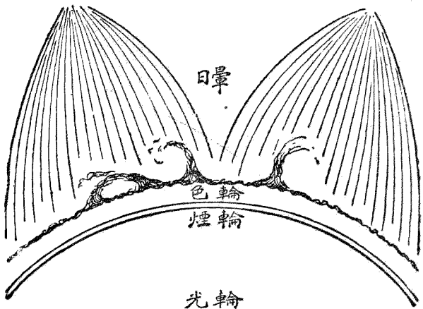
第四圖 太陽各氣層之圖 可與卷首之圖參閱。
