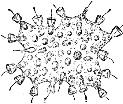
原始海綿
