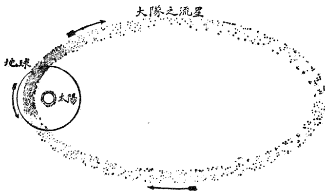
第十五圖 大隕流星之圖並示地球之經過其流
