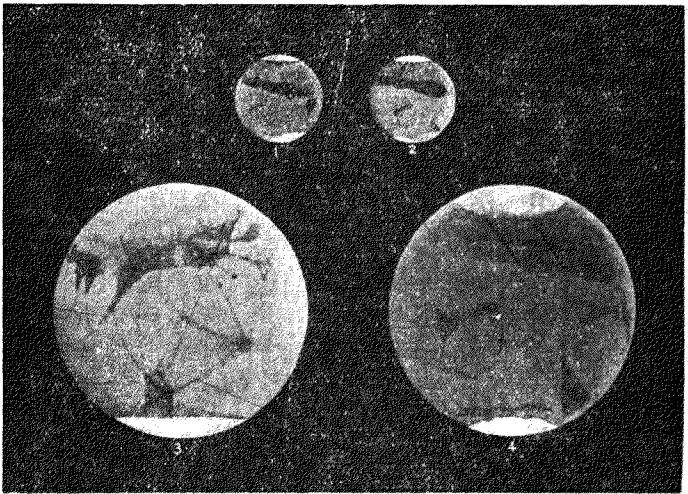
第十圖 火星
