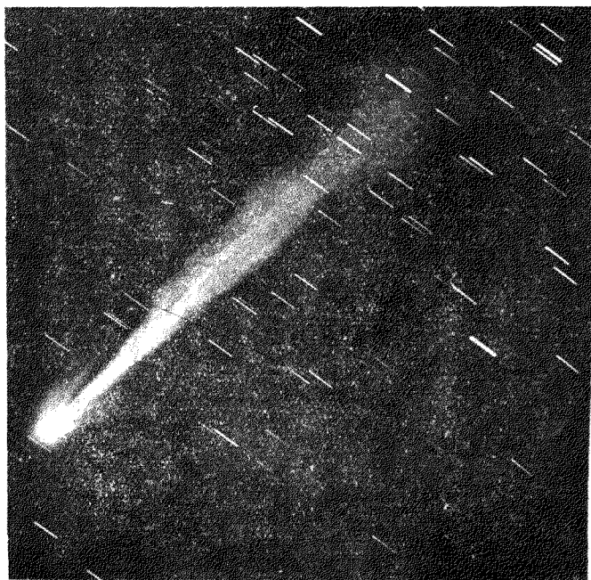
第十六圖 一九〇八年九月二十九日之彗星(格林維基皇家天文臺攝影)
