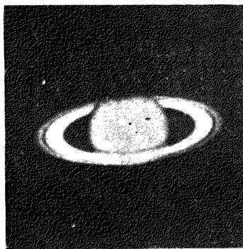
第十二圖 一九一一年十一月十九日之土星
