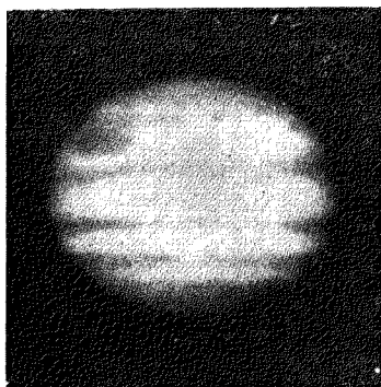
第十一圖 木星
