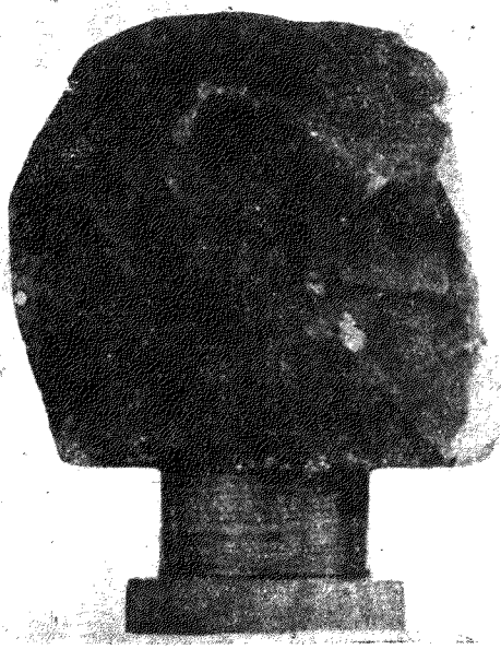
在 斯卡巴洛 (Scarborough) 墜落之隕石 現存自然科學館中，重約五十六磅，爲一石質之隕星。
