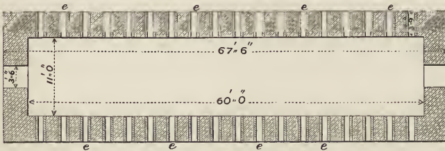
Fig. 9. Ground-plan.
