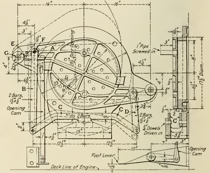
Simple Gravity Fire Door
