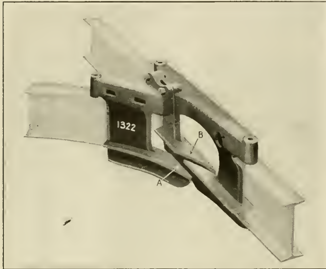
Fig. 2—Cast Stéel Track Switch
