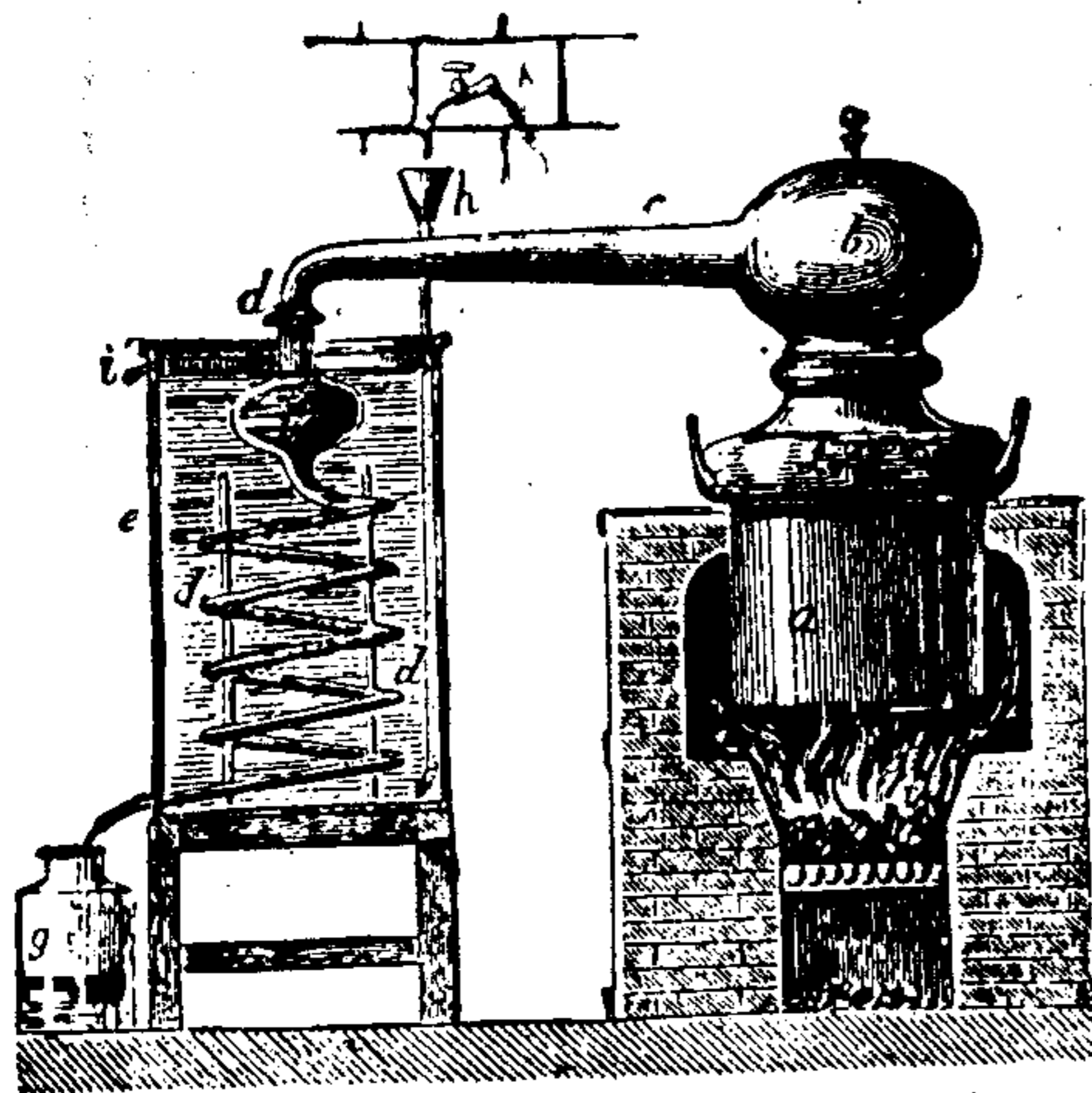
Рис. 15. Перегонный кубъ.
