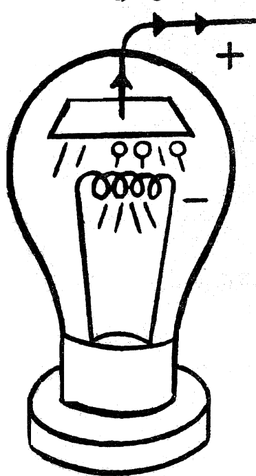
படம் 10: எடிசன் அமைத் துச் சோதித்த மின்குமிழைக் காட்டுவது
