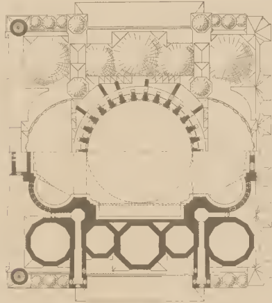
HORIZONTALSCHNITT DURCH DEN TAMBUR DER KLEINEN KUPPELN
