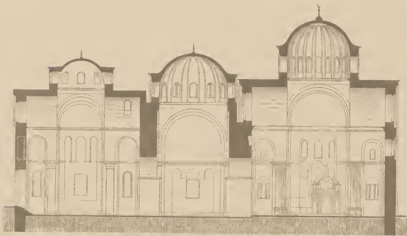
QUERSCHNITT
