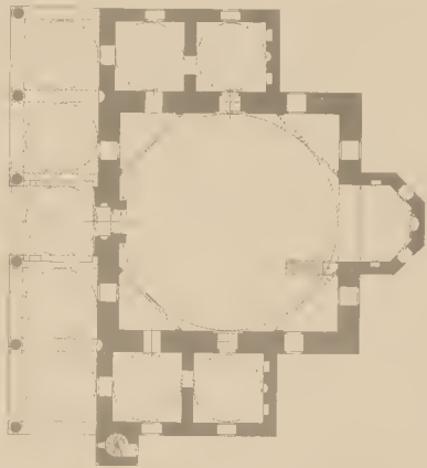
18,b SEKI HÜDREM DSCHAMI, AWRET BASARI ZWICKELÖSUNG DER KUPPEL - GRUNDRISS
