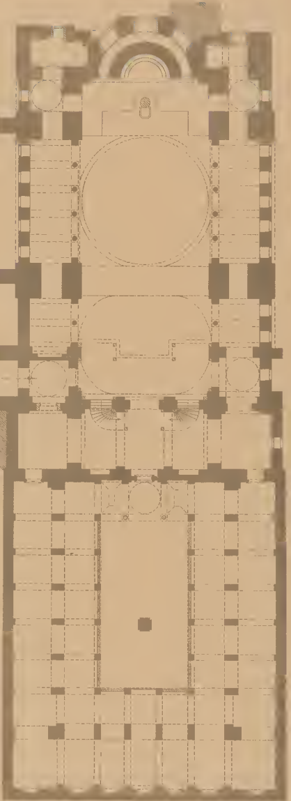
6d IRENE-KIRCHE - OR. N. 114 - 1731 GRUNDRISS
