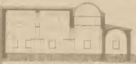
LÄNGSSCHNITT
