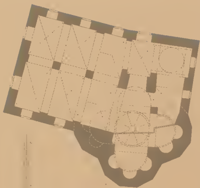
9h KIRCHE MOGLION, JENI KAPU GRUNDRISS
