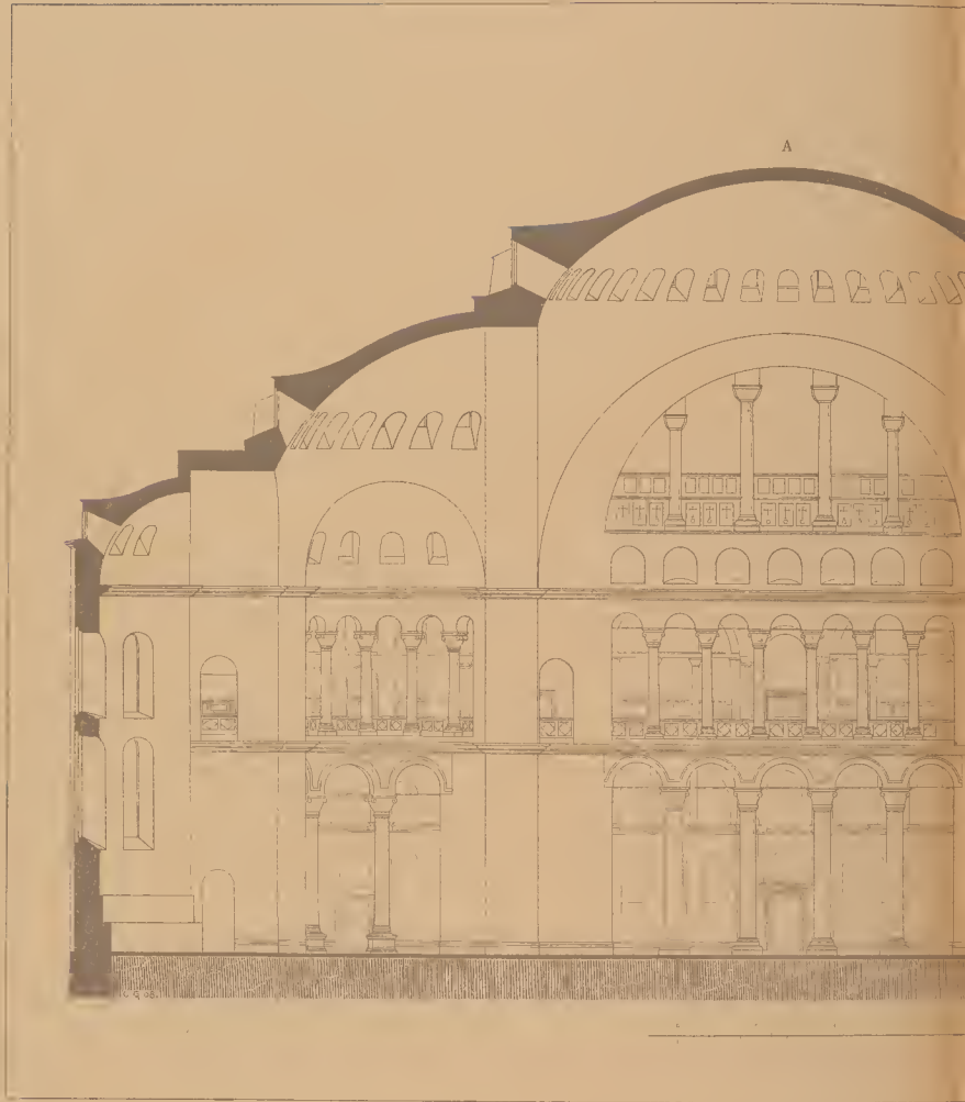
8,d AJA SOFIA, LÄNGSSCHNITT, URSPRÜNGLICH
