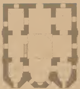
GRUNDRISS
