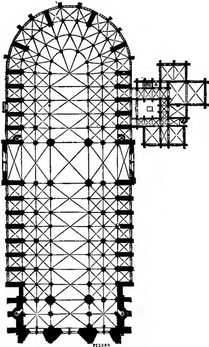
PLAN OF NOTRE-DAME DE PARIS FROM VIOLLET-LE-DUC'S "DICTIONNAIRE DE L'ARCHITECTURE"
