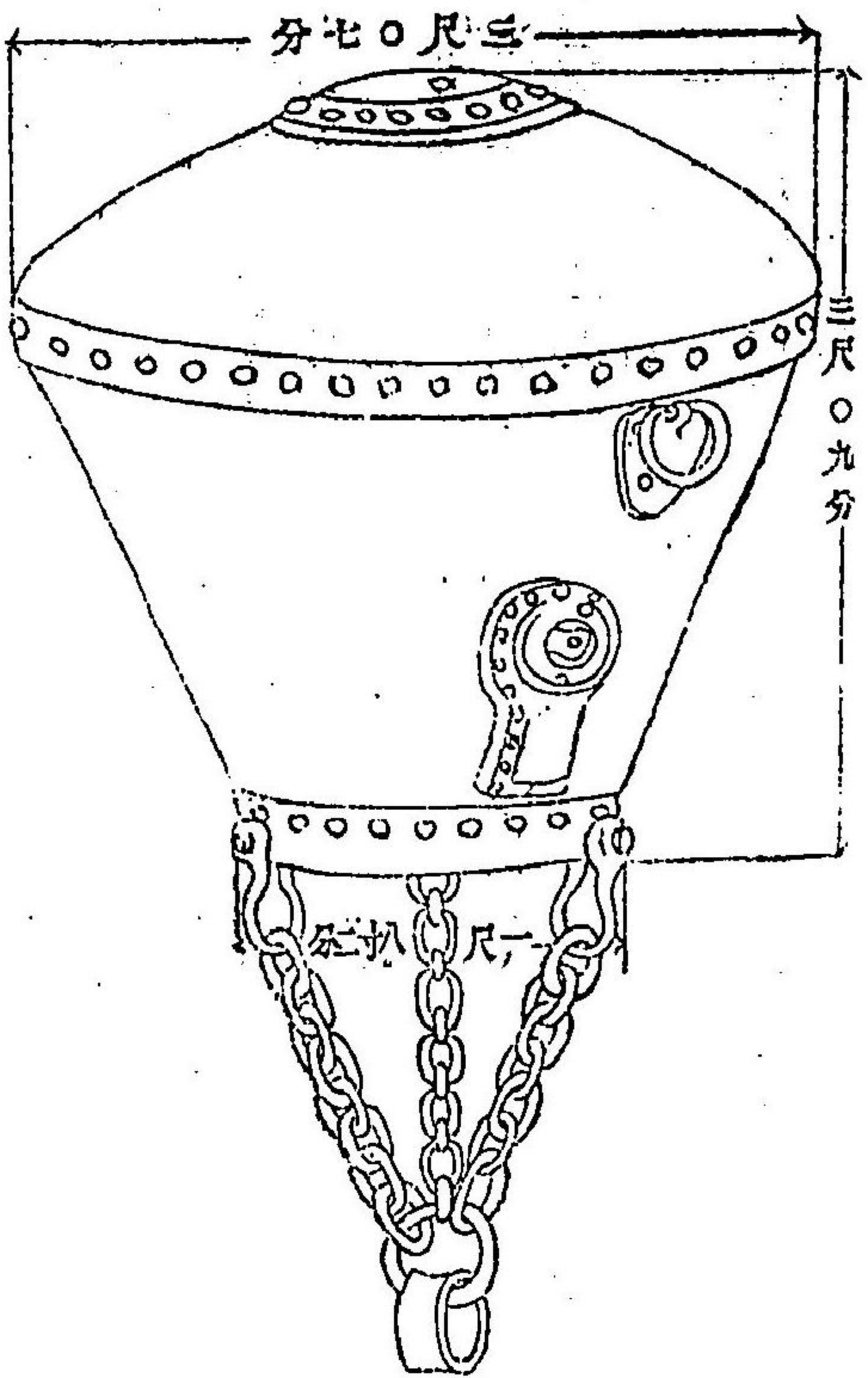
露式電氣機標水雷鐘
