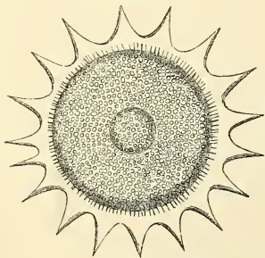
FIG. 212. Haliomma Humboldtii .
