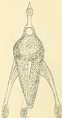
FIG. 210. Podocyrtis Schomburgkii .
