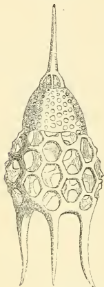
FIG. 210. Podocyrtis Schomburgkii .
