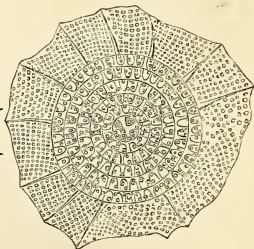
FIG. 212. Haliomma Humboldtii .
