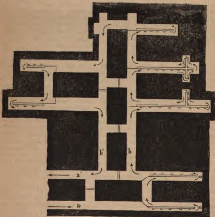
Способъ вентилярованія каменноугольныхъ воней, выдѣляющихъ гремучій газъ. Воздухъ, входящій въ a заставляють, при помощи перегородокъ n , m и t , p , проходить во всѣ мѣста работы. Стрѣлки показываютъ ходъ воздуха, выходящаго изъ a' .
