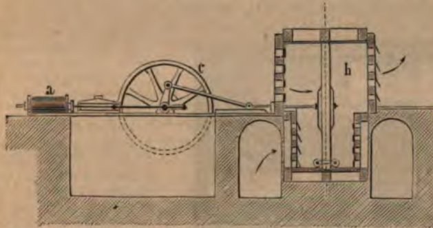
Рудничный поршневои вентиляторъ системы Ньюсона. Поршень h движется въ моментъ изображенія на рис. съ лѣва на право, а потому высасываніе идетъ изъ лѣваго устья, какъ видно по положенію клапановъ.
