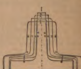
Фиг. 7. Послѣдовательное измѣненіе формы желѣза (и стали) при прокатываніи тавроваго желѣза.
