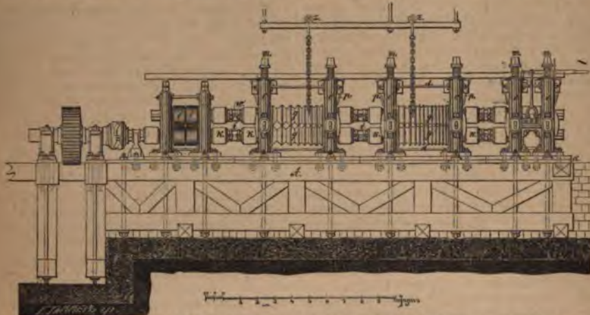
Фиг. 1. Прокатный станъ для полученія сортового желѣза (и стали). Общій продольный видъ.
