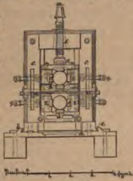
Фиг. 2. Прокатный станъ, какъ на фиг. 1. Поперечный разрѣзъ.
