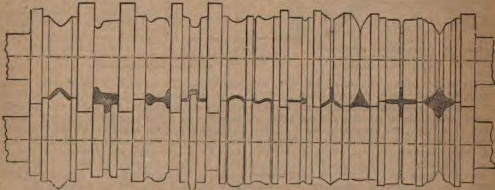
Фиг. 3. Отдѣльные ручьи прокатныхъ вальцовъ для полученія различныхъ сортовъ фасоннаго желѣза (и стали).
