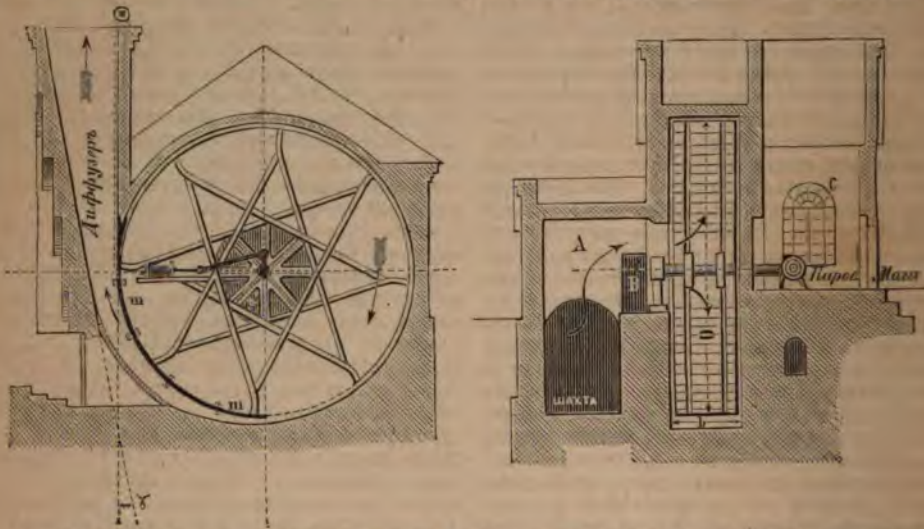
Центробѣжный рудничный вентиляторъ системы Габаля въ вертикальномъ разрѣзѣ, съ зѣва—перпендикулярно оси вращенія, а съ правого по ней. Воздухъ движется отъ оси на окружности и уносится чрезъ диффузоръ.
